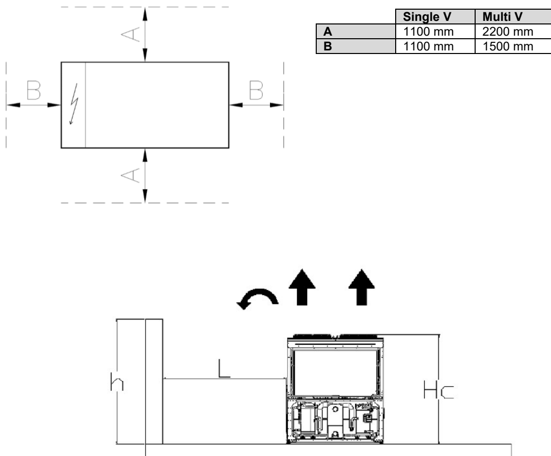
Obrázek 11- Požadavky minimálního prostoru
