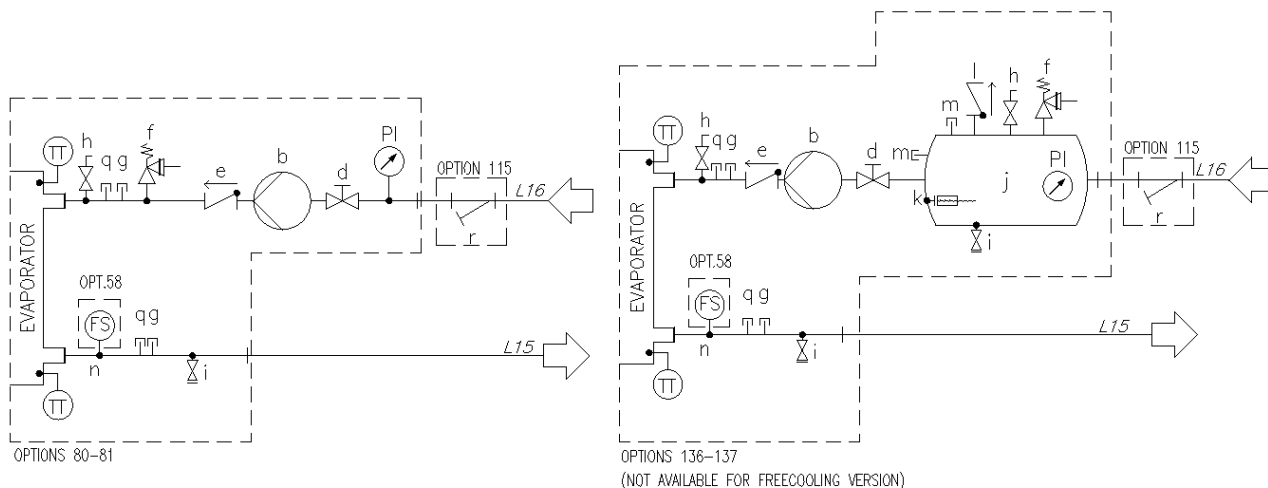
Obrázek 16 - Schéma hydraulické soustavy pro dvojité V (EWATxx5B) čerpadlo (vol. 80-81/136-137) (max. provozní tlak 6 bar)
