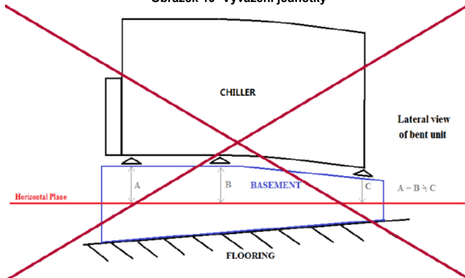
Obrázek 10- Vyvážení jednotky
