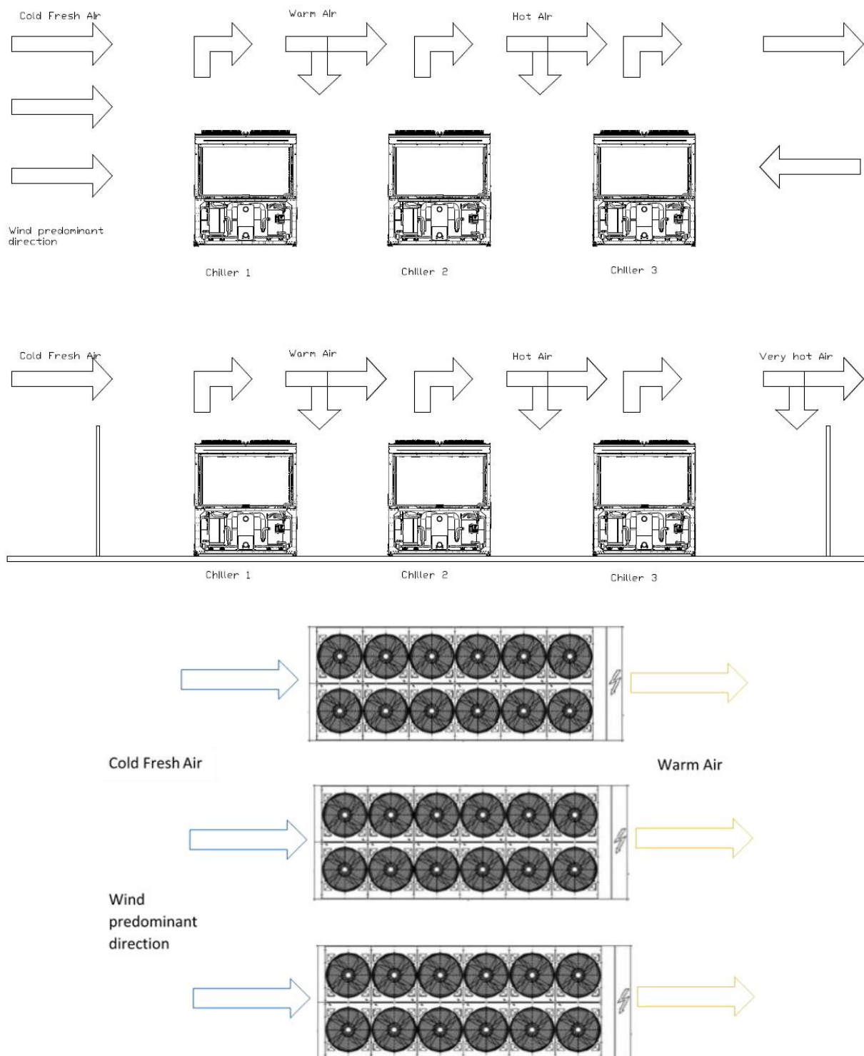
Obrázek 12- Instalace s několika chladiči
