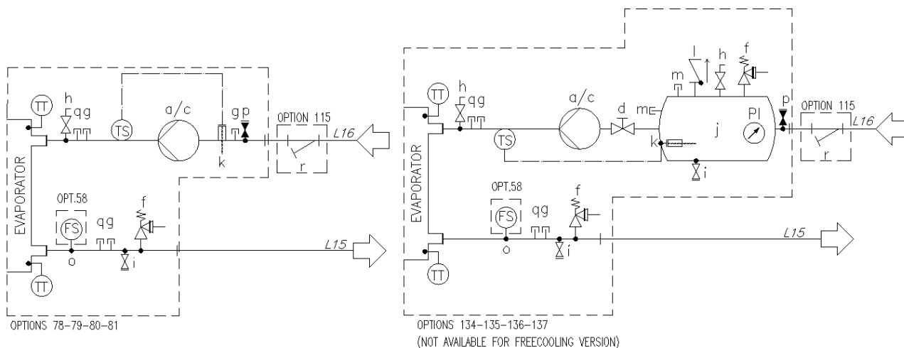
Obrázek 17- Hydraulické schéma pro modulární V (EWATxx0B) (vol. 78-79-80-81/134-135-136-137) (max. provozní tlak 6 bar)
