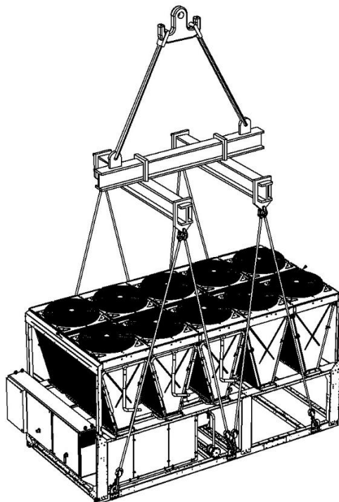
Jednotka se 6 zvedacími body
