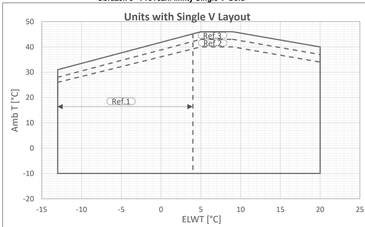
Obrázek 8 - Provozní limity Single V-Gold
