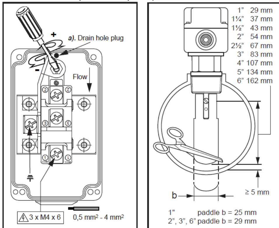
Obrázek 13 – Nastavení průtokového spínače (model F61TB-9100 – Johnson Controls)
