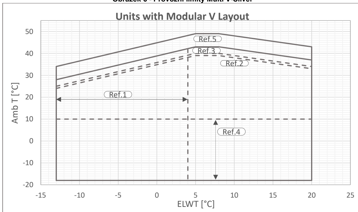
Obrázek 6 - Provozní limity Multi V-Silver
