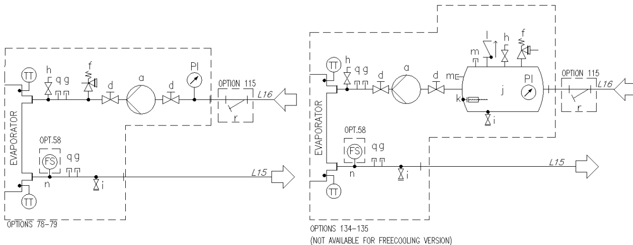
Obrázek 15- Schéma hydraulické soustavy pro jednotlivé V (EWATxx5B) čerpadlo (vol. 78-79/134-135) (max. provozní tlak 6 bar)
