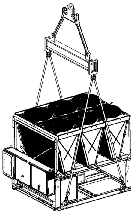
Jednotka se 4 zvedacími body
