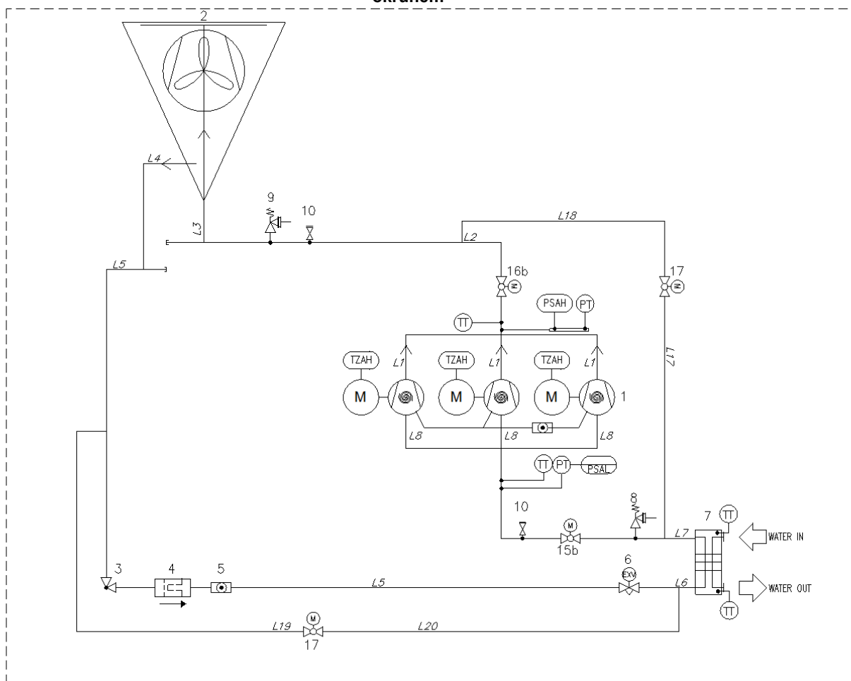
Obrázek 2- Náskres chladicího okruhu (P&ID) jednotka se slabým chlazením venkovním vzduchem jedním okruhem
