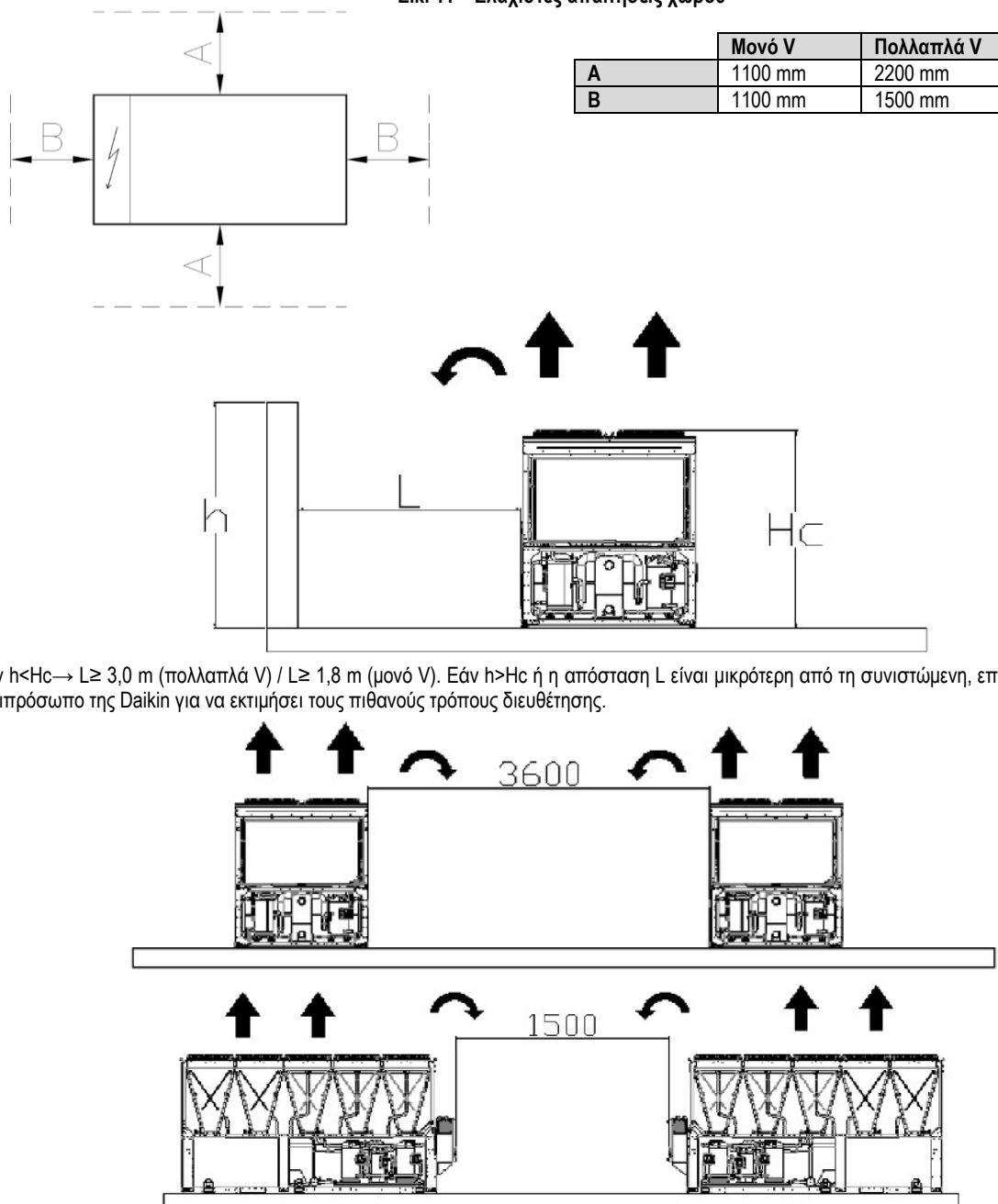
Εικ. 11 – Ελάχιστες απαιτήσεις χώρου
