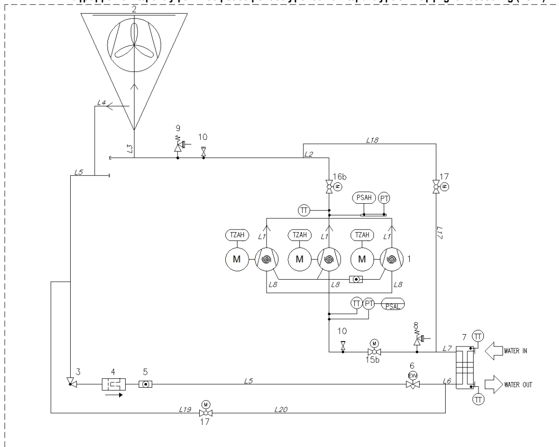
Εικ. 2 – Διάγραμμα κυκλώματος ψυκτικού μέσου μονάδας μονού κυκλώματος με επιλογή light freecooling (P&ID)
