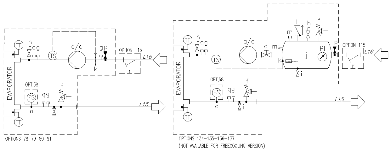
Εικ. 17 – Διάγραμμα υδραυλικού κυκλώματος για Αρθρωτή V (EWATxx0B) (επιλογές 78-79-80-81/134-135-136-137) (μέγιστη πίεση λειτουργίας 6 bar)
