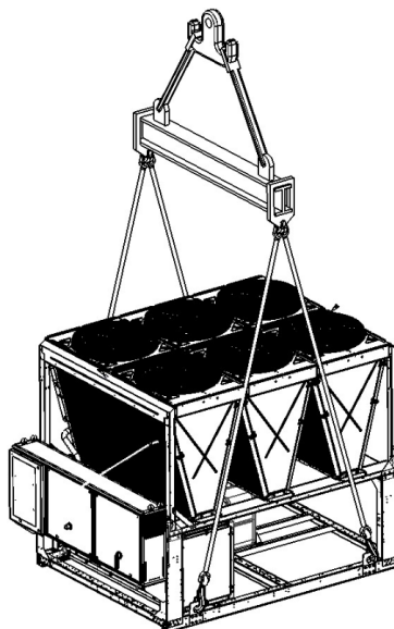
Μονάδα με 4 σημεία ανύψωσης
