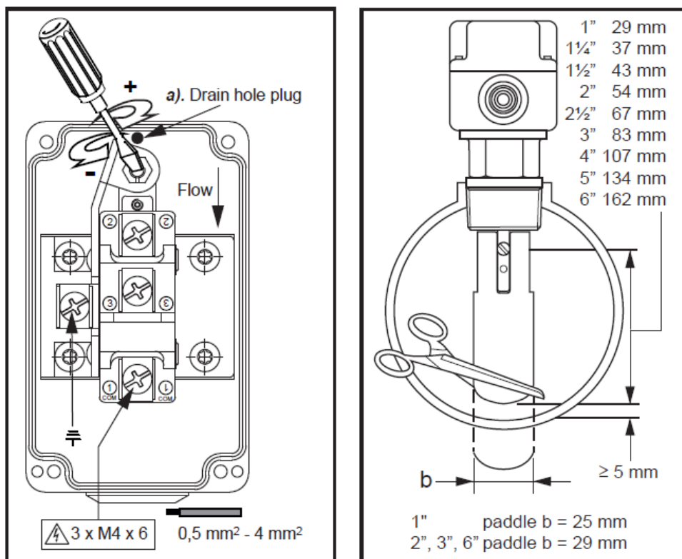
Εικ. 13 – Ρύθμιση διακόπτη ροής (μοντέλο F61TB-9100 – Έλεγχος Johnson)
