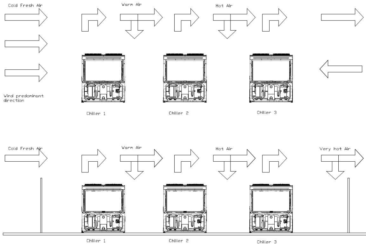
Εικ. 12 – Εγκατάσταση πολλών ψυκτών
