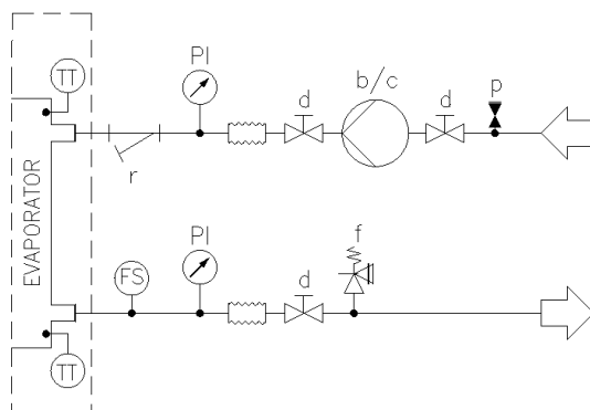
Εικ. 15 – Διάγραμμα υδραυλικού κυκλώματος για μονή αντλία μονού V (EWATxx5B) (επιλογές 78-79/134-135) (μέγιστη πίεση λειτουργίας 6 bar)
