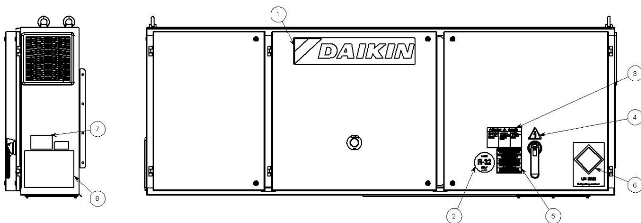
Εικ. 4 – Περιγραφή των ετικετών που υπάρχουν στον ηλεκτρικό πίνακα
