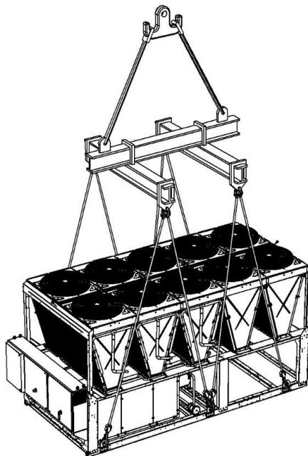
Μονάδα με 6 σημεία ανύψωσης
