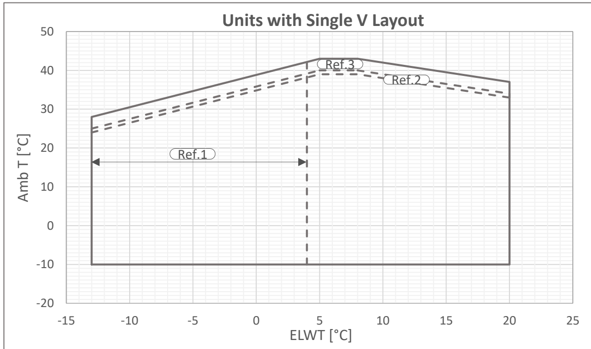
Εικ. 8 – Μονό V - Όρια λειτουργίας Gold
