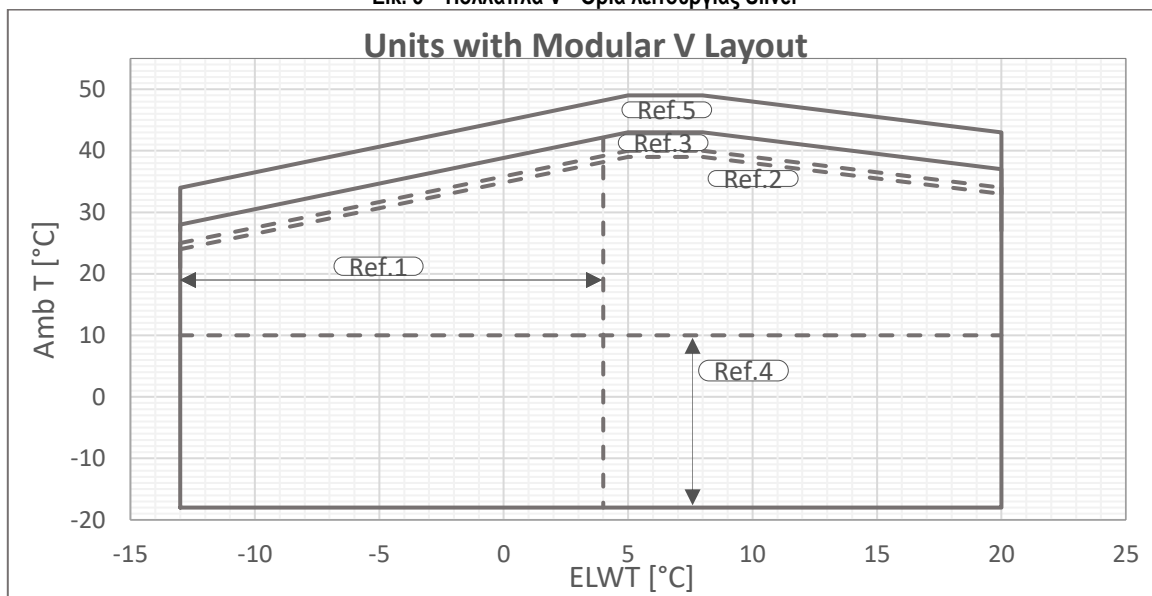
Εικ. 6 – Πολλαπλά V - Όρια λειτουργίας Gold
