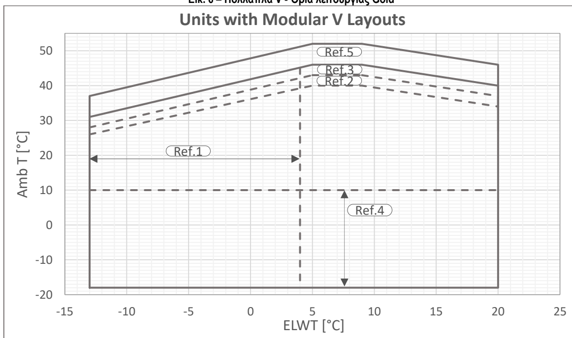
Εικ. 6 – Πολλαπλά V - Όρια λειτουργίας Gold
