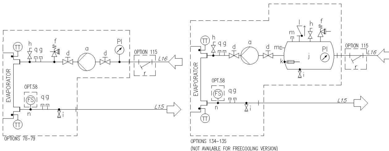
Εικ. 15 – Διάγραμμα υδραυλικού κυκλώματος για μονή αντλία μονού V (EWATxx5B) (επιλογές 78-79/134-135) (μέγιστη πίεση λειτουργίας 6 bar)
