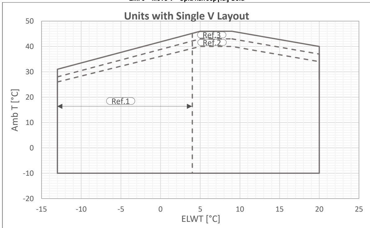
Εικ. 8 – Μονό V - Όρια λειτουργίας Gold
