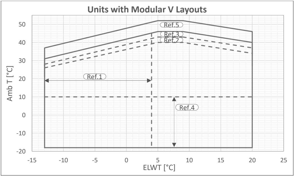
Fig. 6 - Límites operativos de Multi V-Oro
