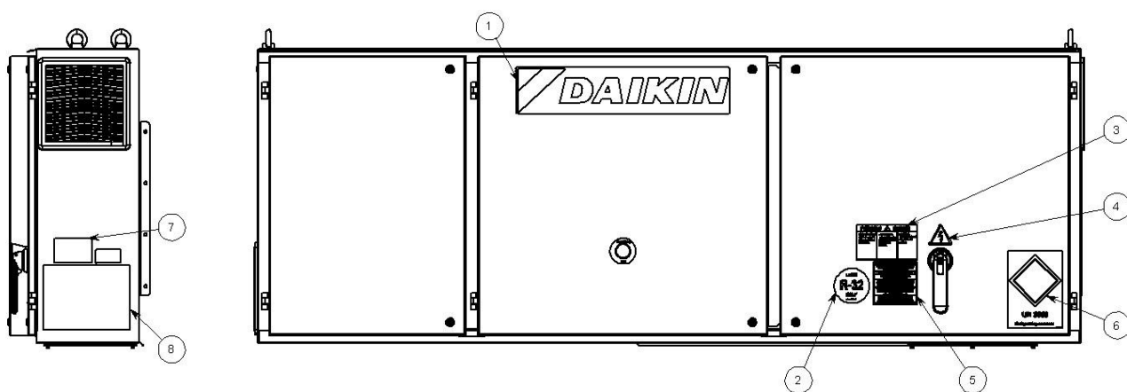
Fig. 4 - Descripción de las etiquetas aplicadas al panel eléctrico
