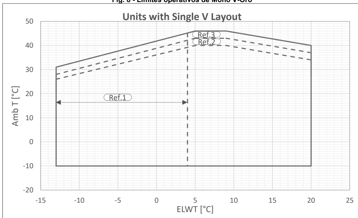
Fig. 8 - Límites operativos de Mono V-Oro
