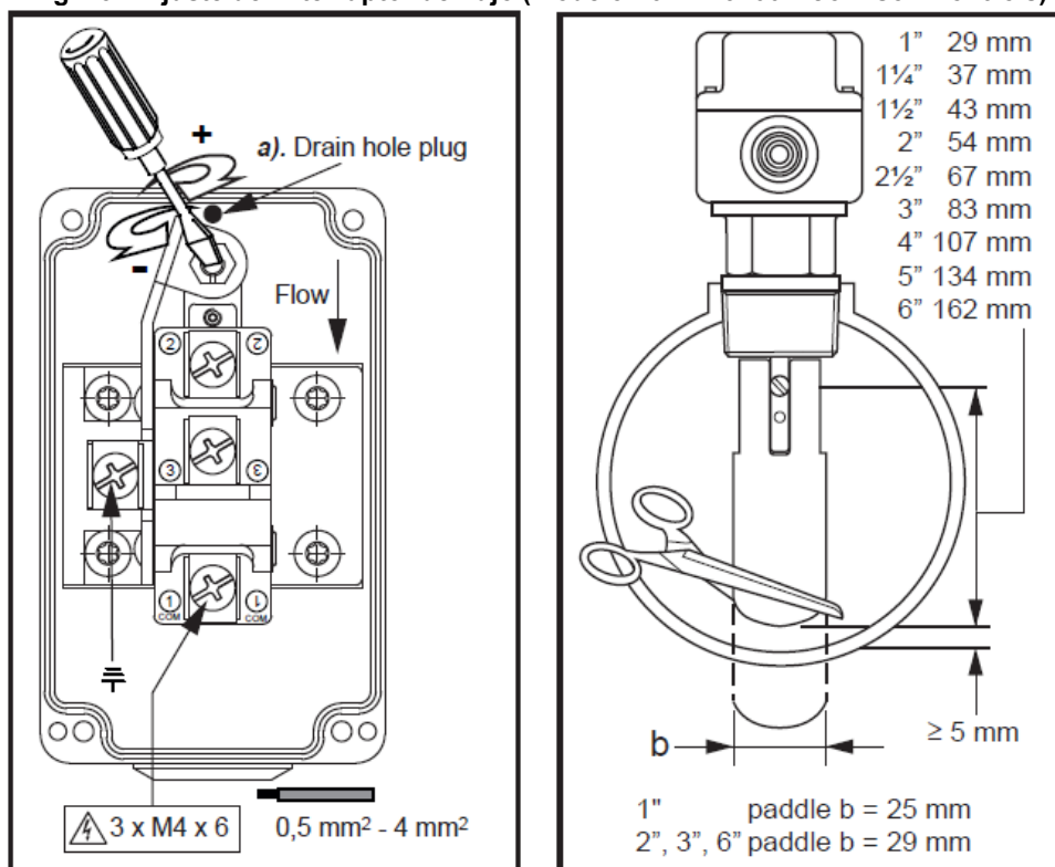
Fig. 13 – Ajuste del interruptor de flujo (modelo F61TB-9100 – Johnson Controls)
