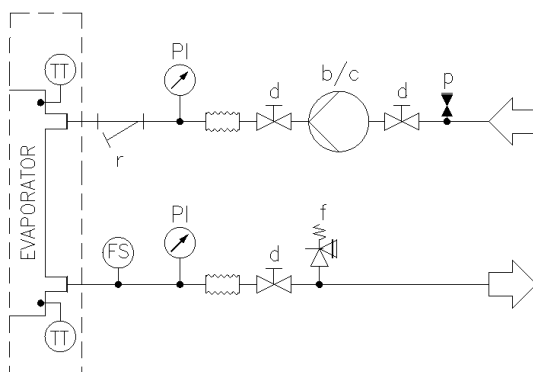
Fig. 15 – Diagrama hidráulico para mono V (EWATxx5B) única bomba (opc. 78-79/134-135) (presión operativa máxima 6 bares)
