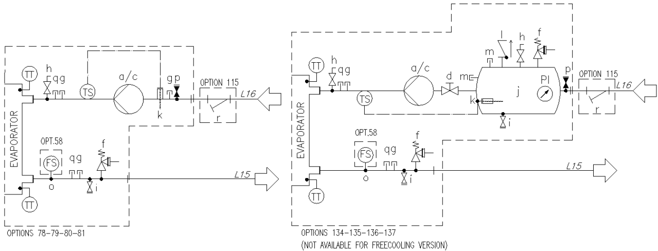
Fig. 17 - Diagrama hidráulico para Modular V (EWATxx0B) (opc. 78-79-80-81/134-135-136-137) (presión operativa máxima 6 bares)
