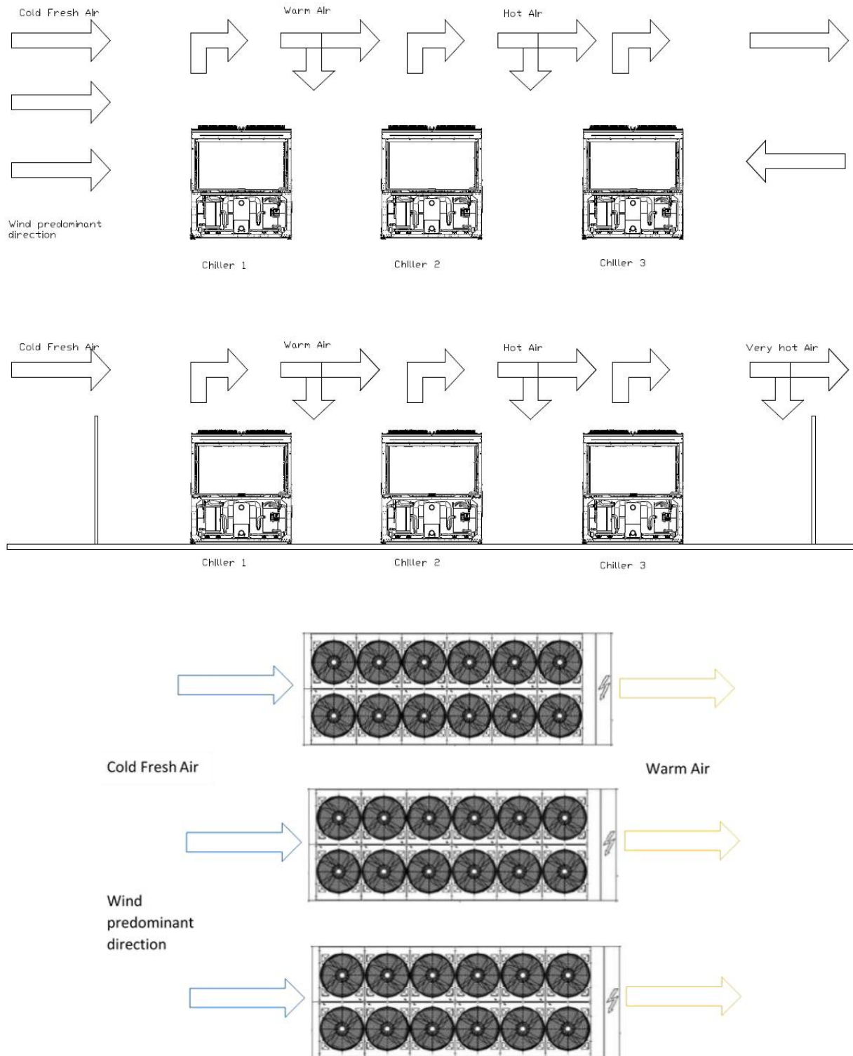
Fig. 12 – Instalación de Múltiples Refrigeradores
