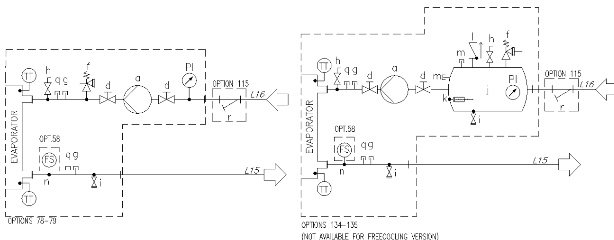
Fig. 15 – Diagrama hidráulico para mono V (EWATxx5B) única bomba (opc. 78-79/134-135) (presión operativa máxima 6 bares)
