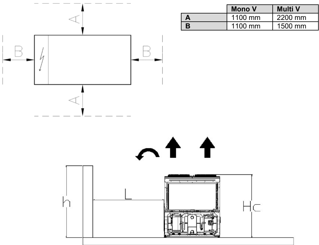
Fig. 11 - Requisitos de espacio mínimo
