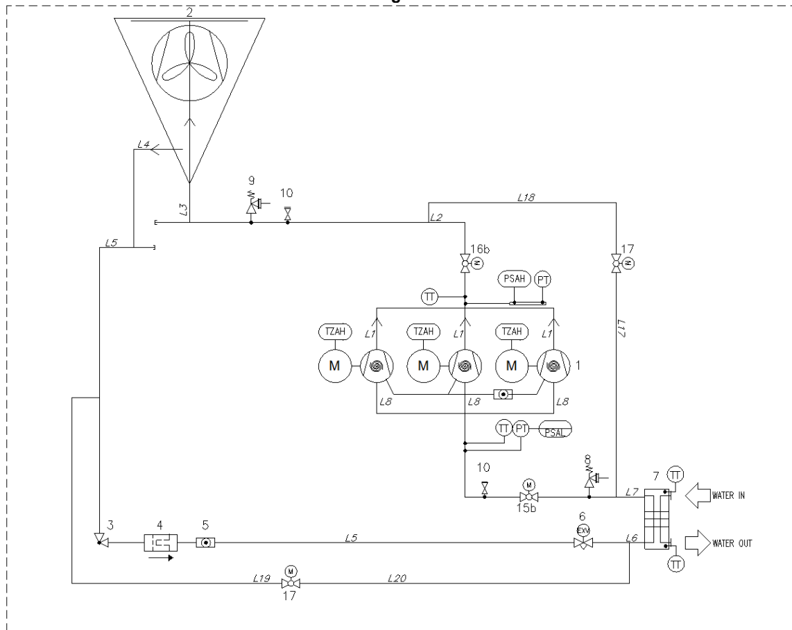
Fig. 2 - Diagrama de circuito refrigerante (P & ID) con unidad de circuito simple con la opción de freecooling ligero
