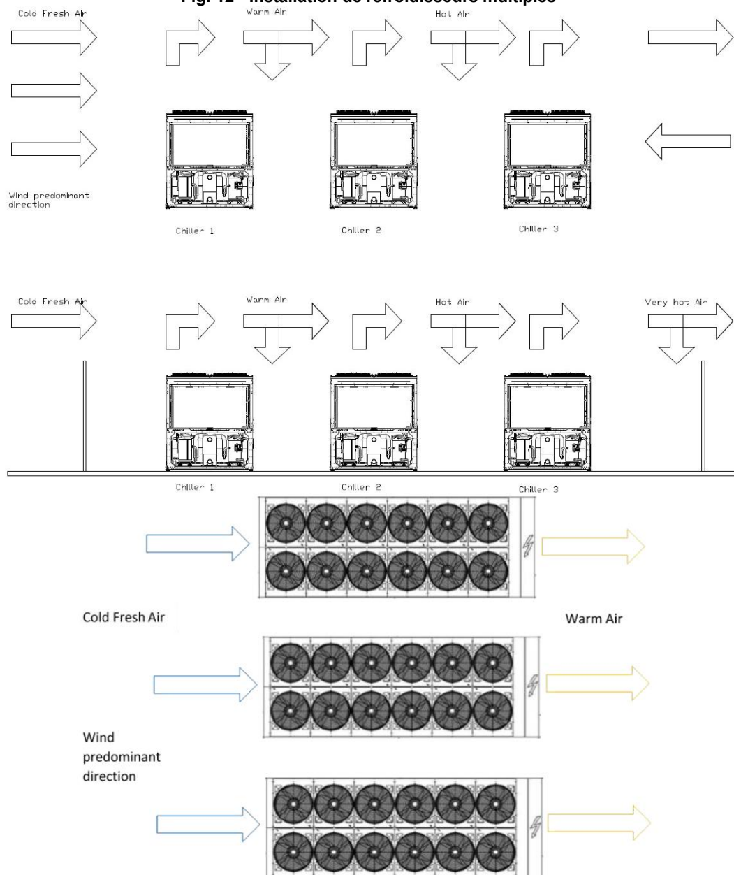
Fig. 12 - Installation de refroidisseurs multiples
