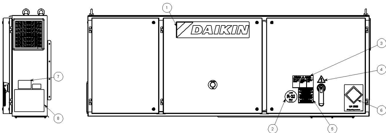
Fig. 4 - Description des étiquettes appliquées sur le Table électrique
