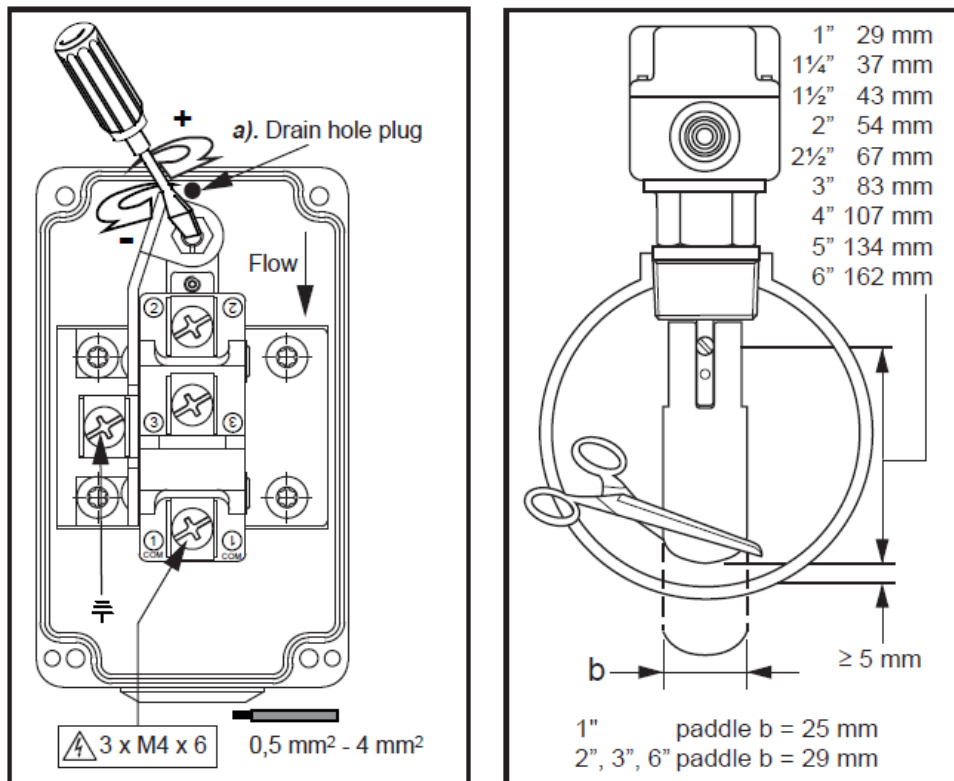
Fig. 13 – Réglage du fluxostat(modèle F61TB-9100 – Johnson Controls)
