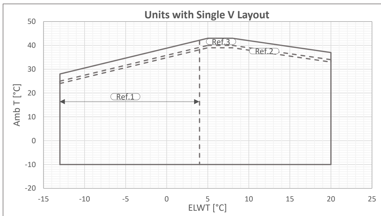
Fig. 8 - Limites opérationnelles Single V-Gold
