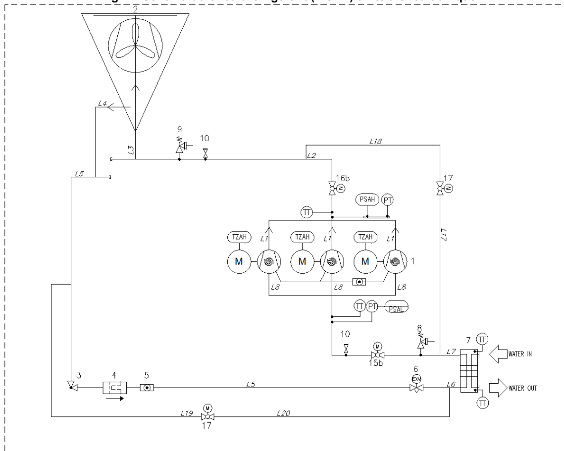
Fig. 2 - Schéma du circuit réfrigérant (P & ID) unité à circuit unique
