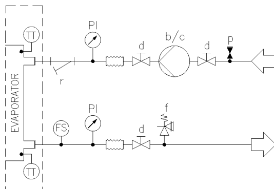
Fig. 15 - Diagramme hydraulique pour V unique (EWATxx5B) pompe unique (opt. 78-79/134-135) (pression de service max. 6 bar)
