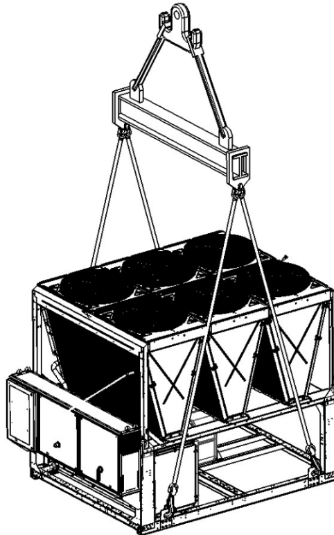
Unité à 4 points de levage
