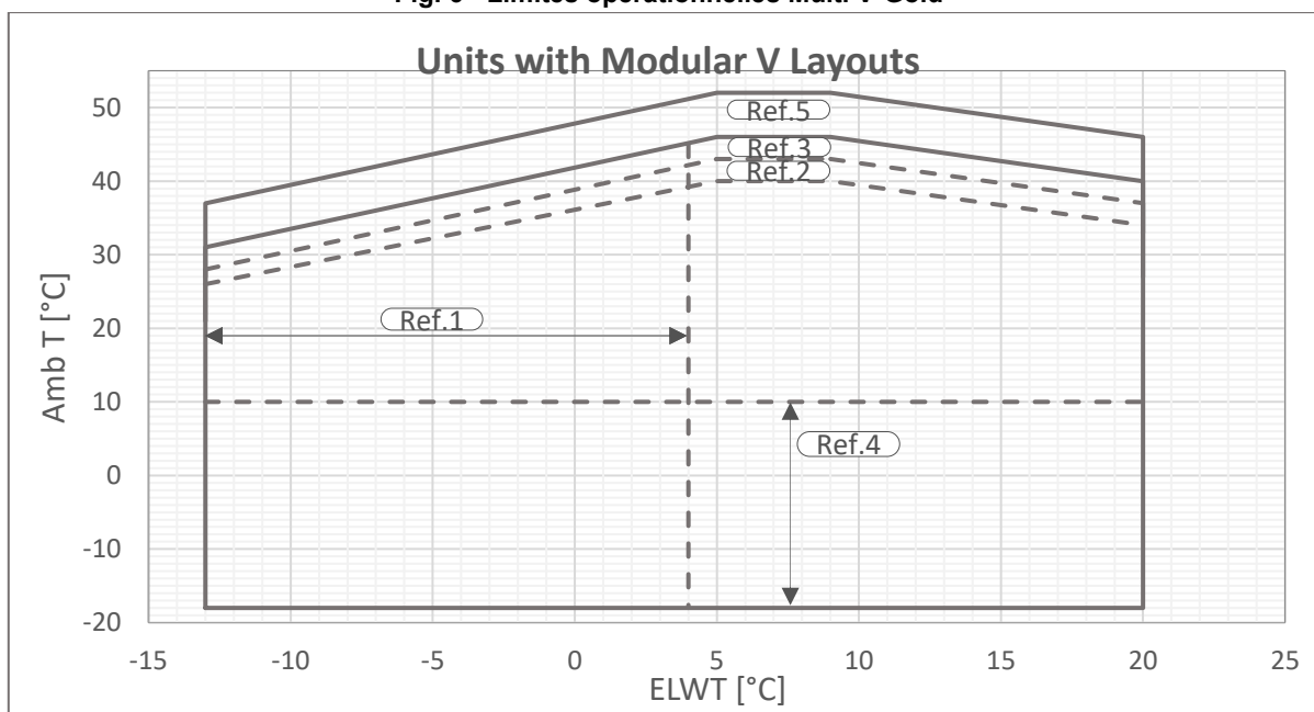
Fig. 6 - Limites opérationnelles Multi V-Gold
