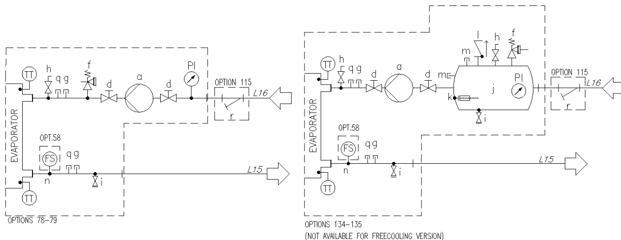
Fig. 15 - Diagramme hydraulique pour V unique (EWATxx5B) pompe unique (opt. 78-79/134-135) (pression de service max. 6 bar)
