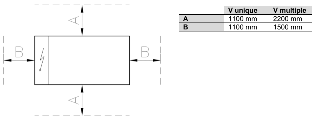
Fig. 11 - Encombrement minimal
