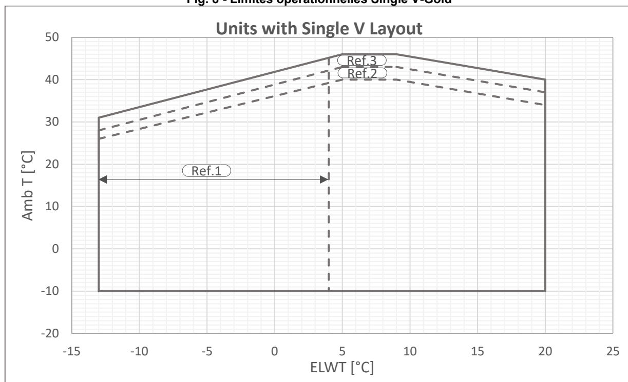
Fig. 8 - Limites opérationnelles Single V-Gold
