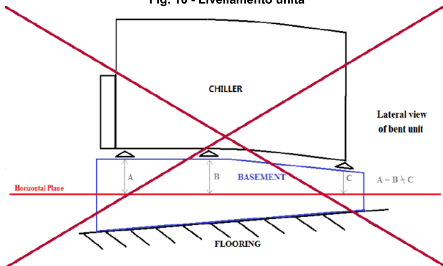
Fig. 10 - Livellamento unità
