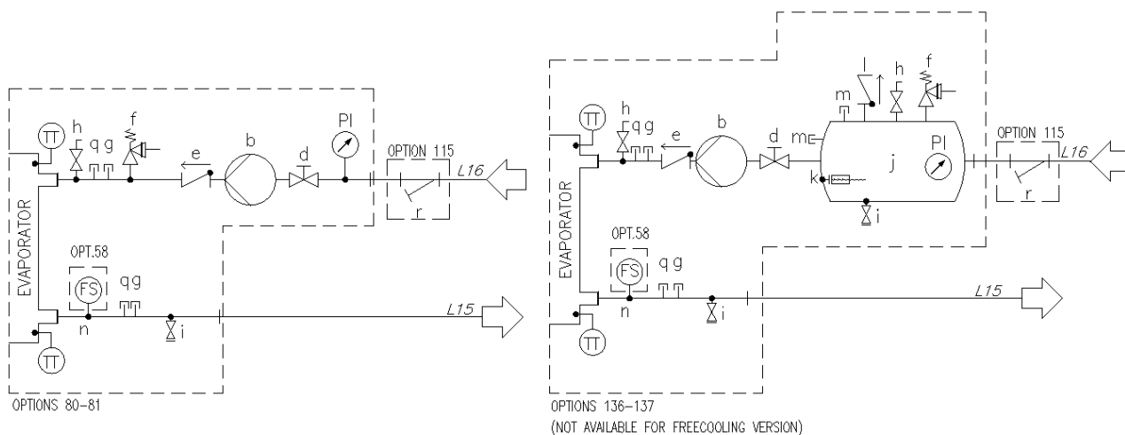
Fig. 16 – Schema idraulico per pompa doppia single V (EWATxx5B) (opz. 80-81/136-137) (pressione massima operativa 6 bar)
