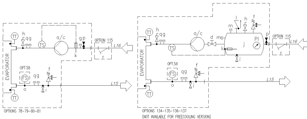
Fig. 17 - Schema idraulico per Modular V (EWATxx0B) (opz. 78-79-80-81/134-135-136-137) (pressione massima operativa 6 bar)
