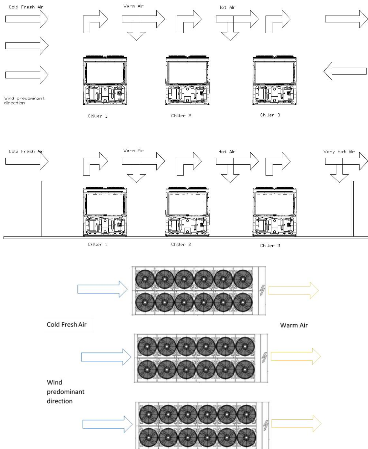
Fig. 12 - Installazione di chiller multipli
