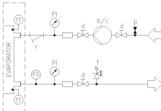
Fig. 15 – Schema idraulico per pompa singola single V (EWATxx5B) (opz. 78-79/134-135) (pressione massima operativa 6 bar)
