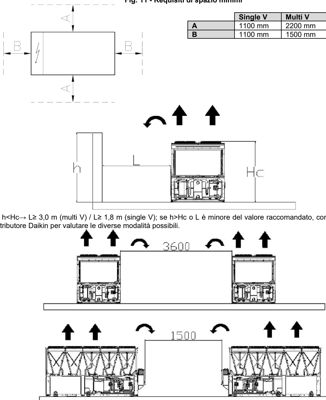
Fig. 11 - Requisiti di spazio minimi
