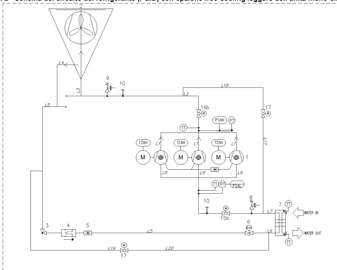
Fig. 2 - Schema del circuito del refrigerante (P&ID) con opzione free-cooling leggero dell'unità mono-circuito
