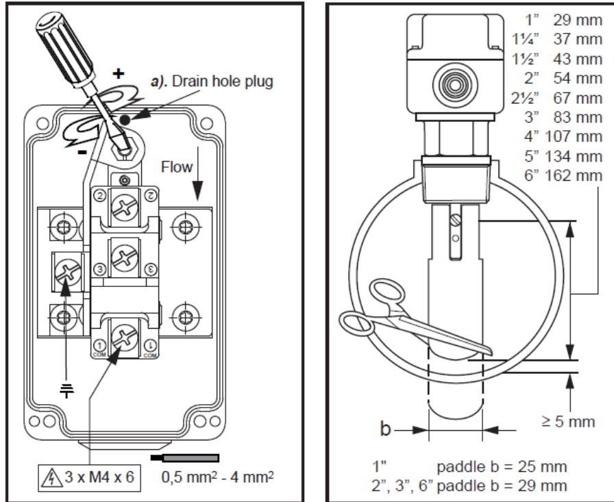
Fig. 13 – Regolazione del flussostato (modello F61TB-9100 – Johnson Controls)
