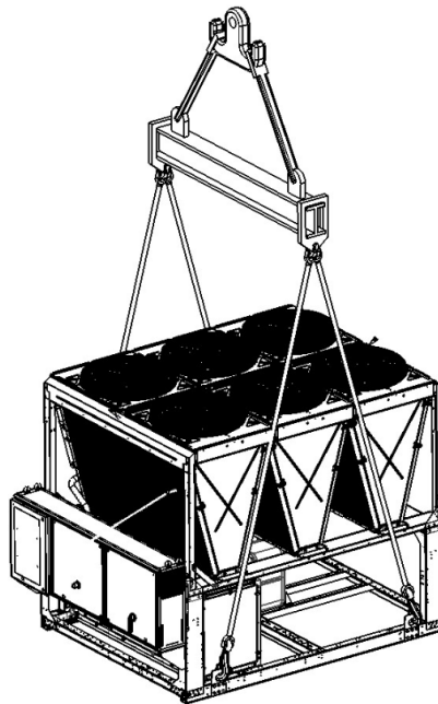
Fig. 9– Istruzioni di sollevamento
