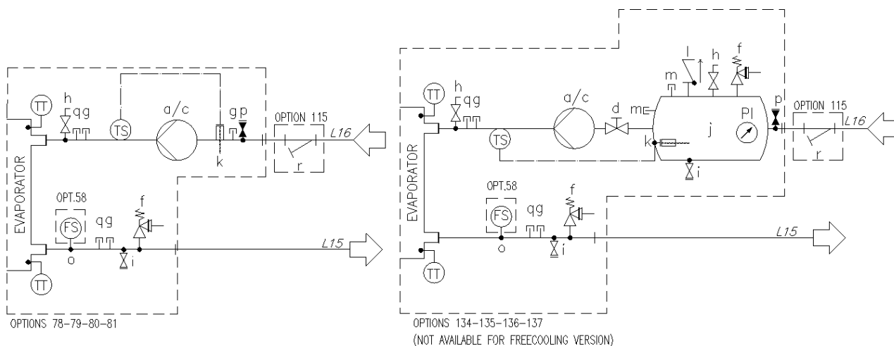
Afb. 17 - Hydraulisch schema voor modulaire V (EWATxx0B) (optie 78-79-80-81/134-135-136-137) (max. bedrijfsdruk 6 bar)
