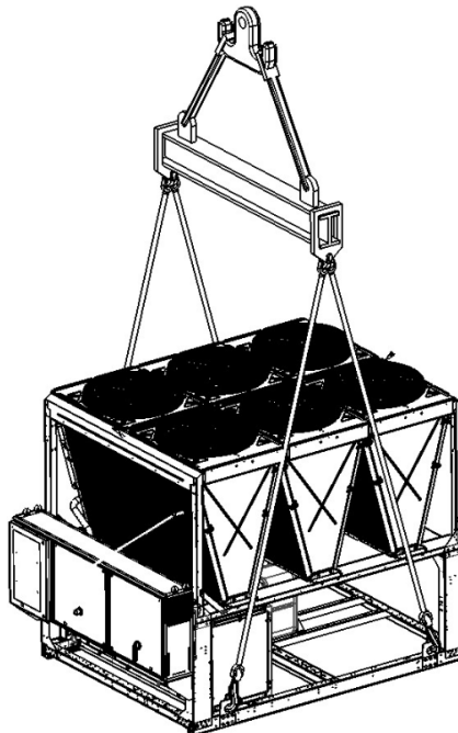
Systeem met 4 hefpunten
