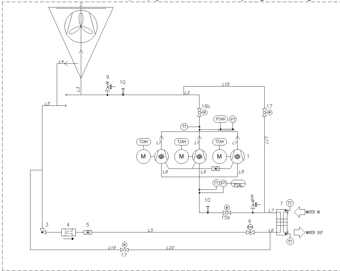
Afb. 2 - Schema koelcircuit (P&ID) systeem enkel circuit en optie light freecooling
