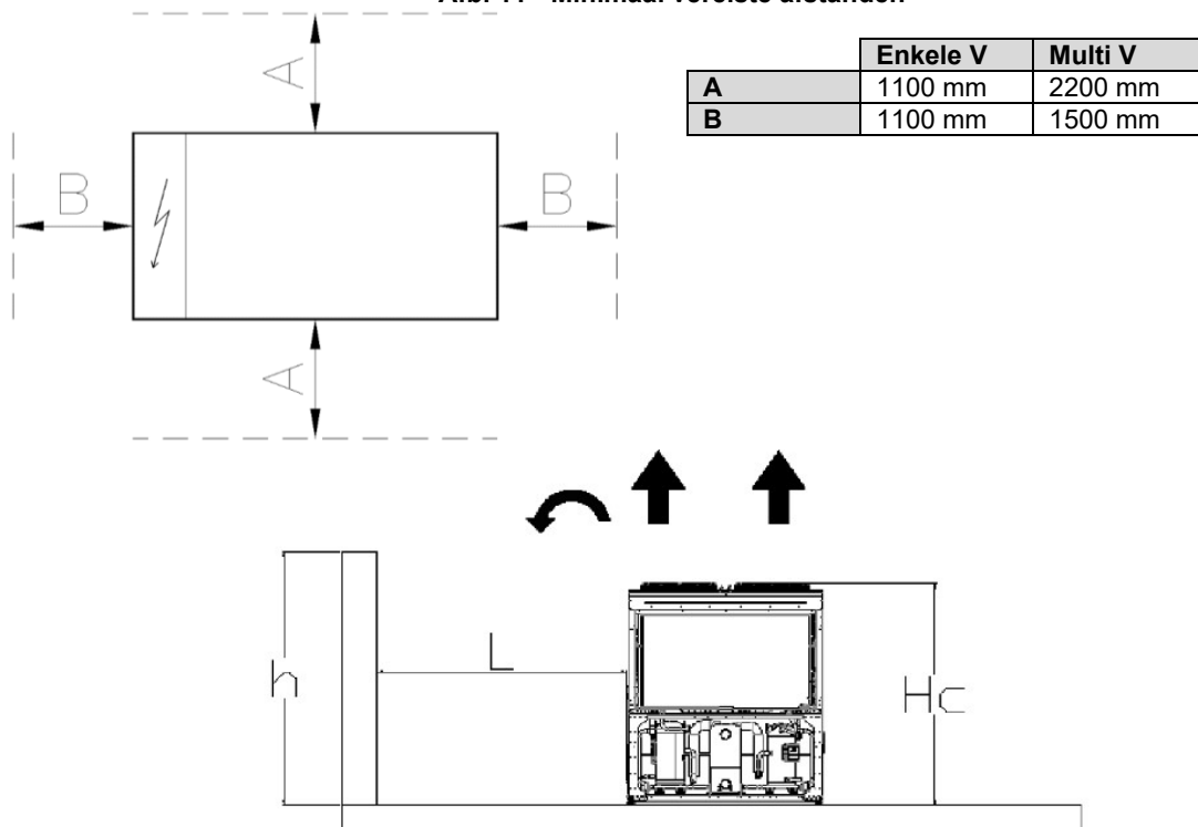
Afb. 11 - Minimaal vereiste afstanden
