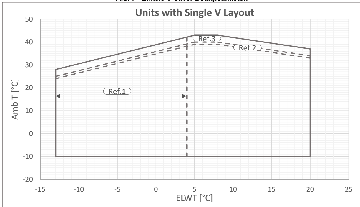
Afb. 8 - Enkele V-Gold Bedrijfslimieten
