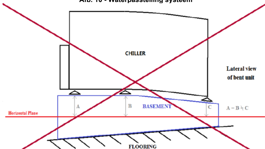
Afb. 10 - Waterpasstelling systeem
