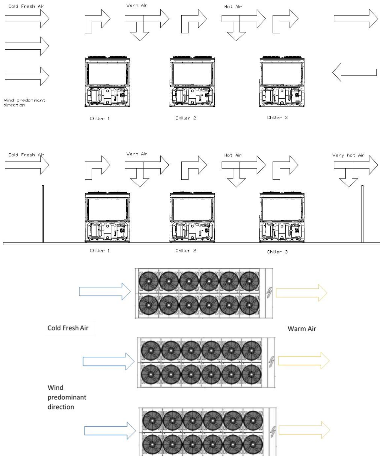
Afb. 12 – Installatie meerdere koelers
