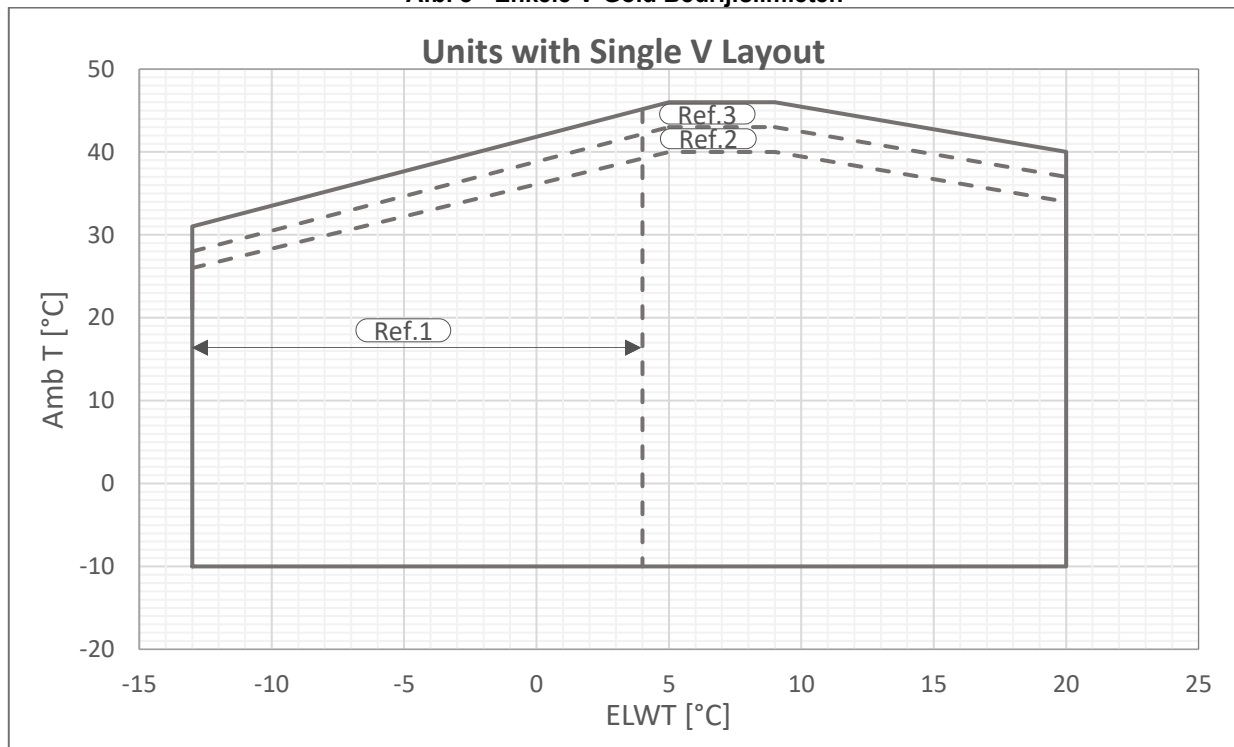
Afb. 8 - Enkele V-Gold Bedrijfslimieten
