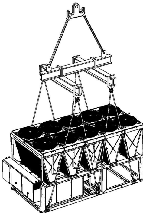
Systeem met 6 hefpunten
