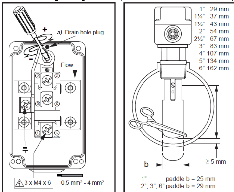
Afb. 13 – Afstelling stromingsschakelaar (model F61TB-9100 – Johnson Controls)
