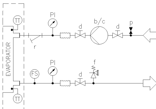
Afb. 15 – Hydraulisch schema voor enkele V (EWATxx5B) enkele pomp (optie 78-79/134-135) (max. bedrijfsdruk 6 bar)
