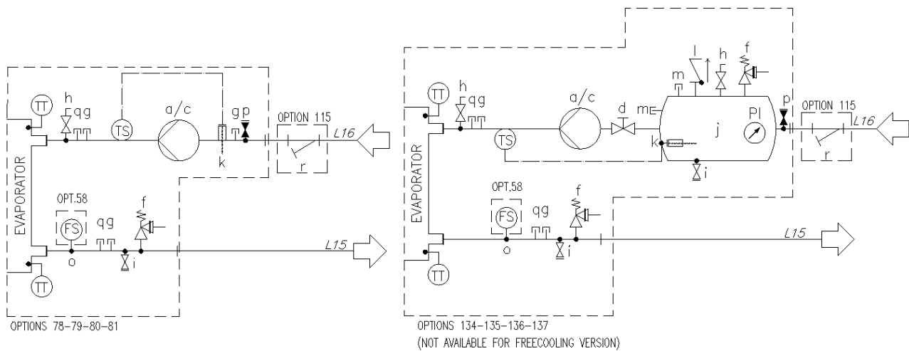
Рис. 17. Гидравлическая схема мультисекционного агрегата (EWATxx5B) (компл. 78-79-80-81/134-135-136-137) (макс. рабочее давление 6 бар)
