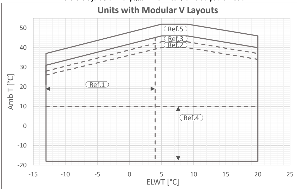
Рис. 6. Эксплуатационные пределы мультисекционного агрегата V-Gold
