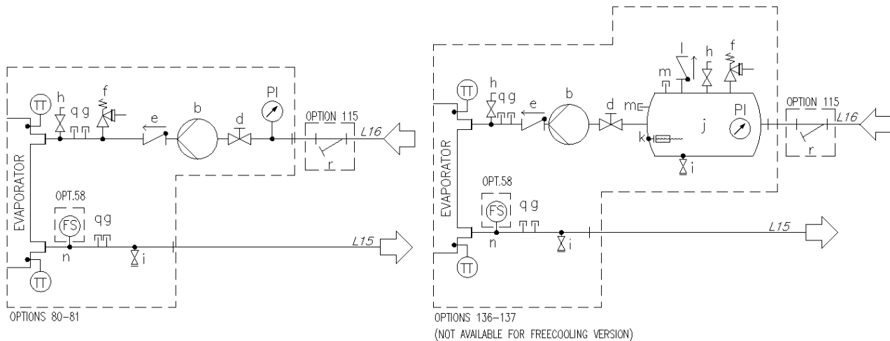
Рис. 16. Гидравлическая схема односекционного агрегата (EWATxx5B) со сдвоенным насосом (компл. 80-81/136-137) (макс. рабочее давление 6 бар)
