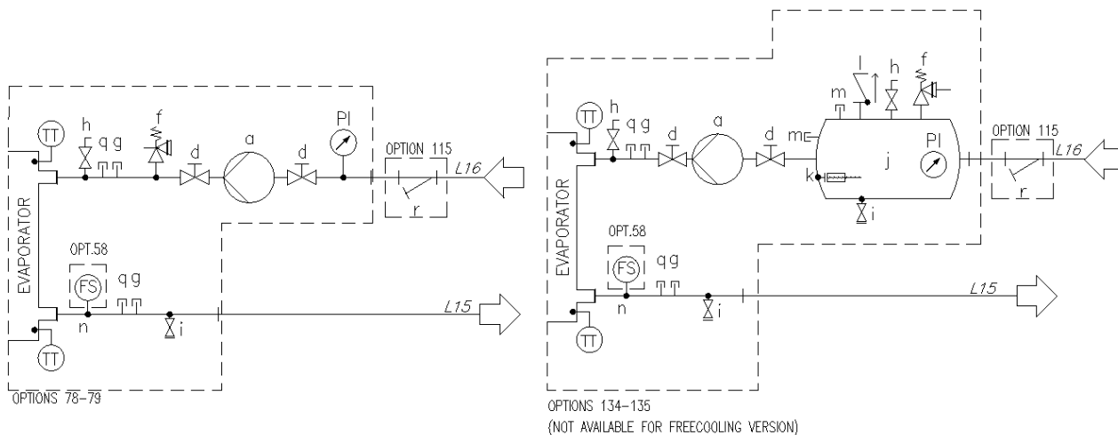
Рис. 15. Гидравлическая схема односекционного агрегата (EWATxx5B) с одним насосом (компл. 78-79/134-135) (макс. рабочее давление 6 бар)
