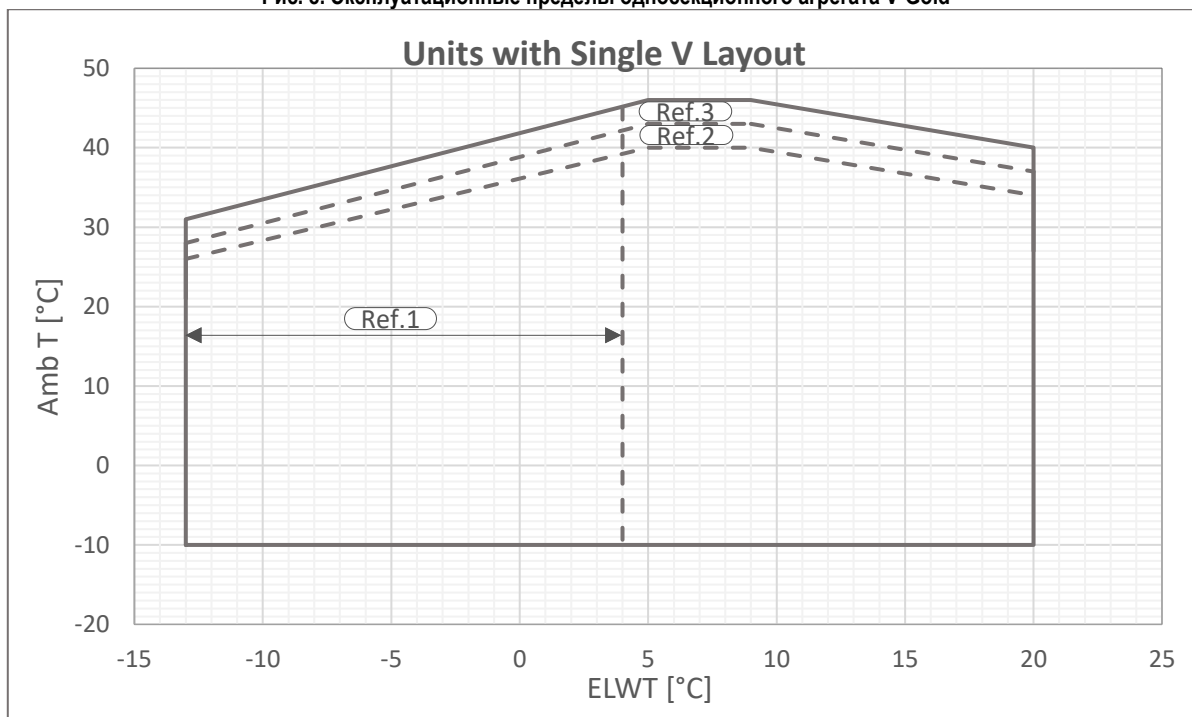
Рис. 8. Эксплуатационные пределы односекционного агрегата V-Gold
