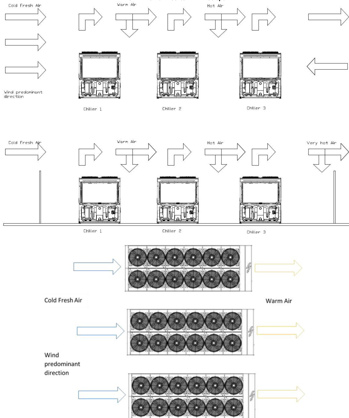
Рис. 12. Монтаж нескольких чиллеров
