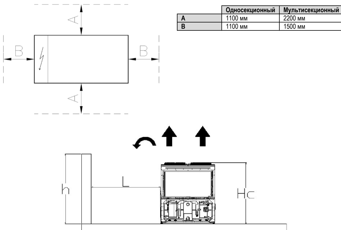
Рис. 11. Требования к расстоянию в свету
