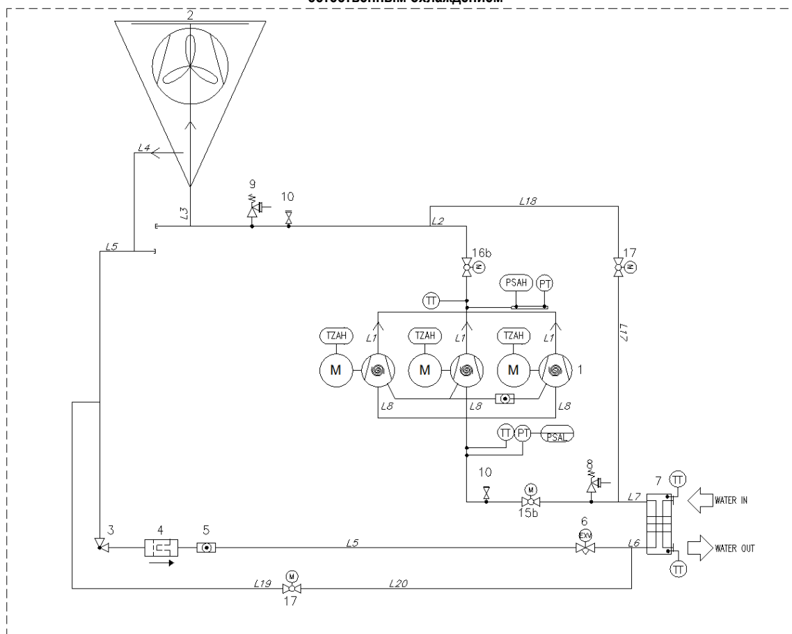
Рис. 2. Схема контура хладагента (схема трубопроводов и КИП) для типового одноконтурного агрегата с частичным естественным охлаждением
