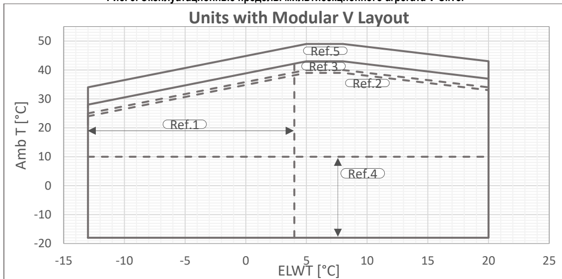
Рис. 6. Эксплуатационные пределы мультисекционного агрегата V-Gold
