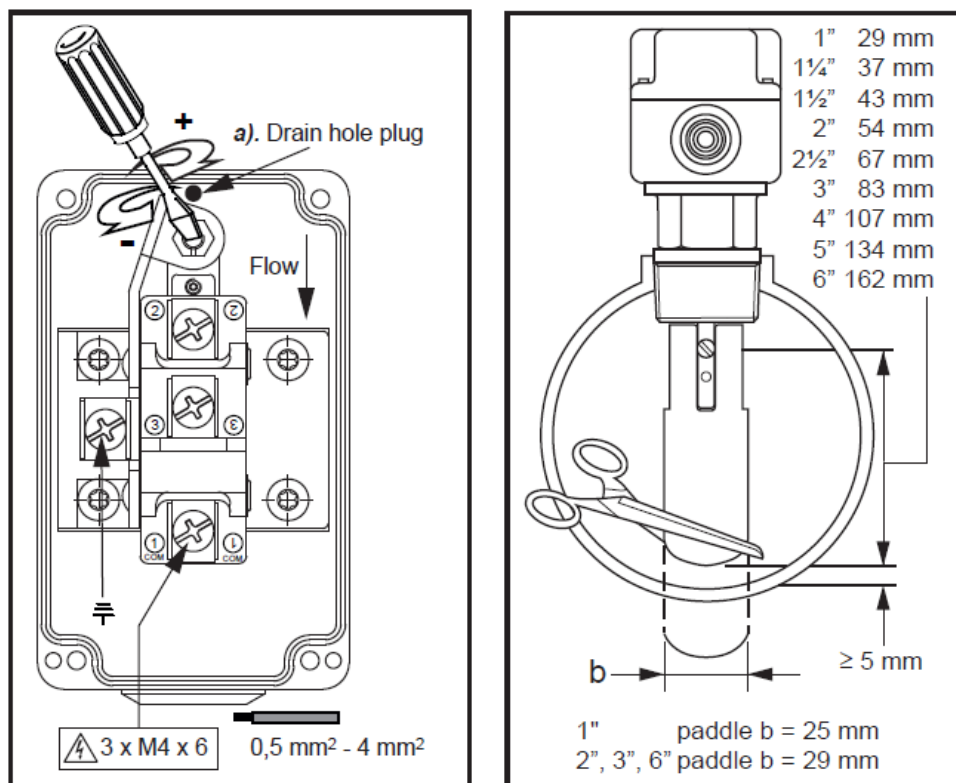
Рис. 13 – Регулировка реле протока (модель F61TB-9100 – Johnson Controls)
