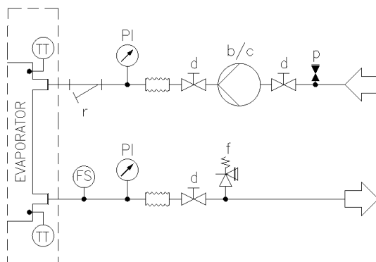
Рис. 15. Гидравлическая схема односекционного агрегата (EWATxx5B) с одним насосом (компл. 78-79/134-135) (макс. рабочее давление 6 бар)
