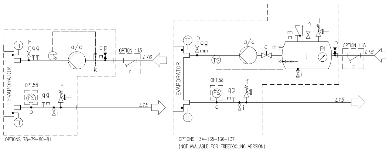
Obr. 17 – Hydraulická schéma pre Modular V (EWATxx0B) (vol. 78-79-80-81/134-135-136-137) (max. prevádzkový tlak 6 barov)
