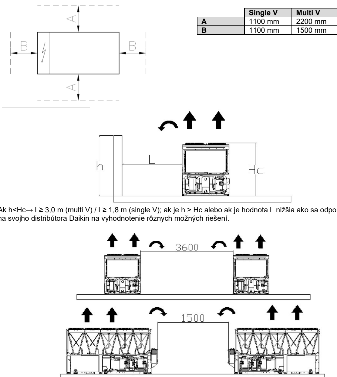
Obr. 11 – Minimálne požiadavky na priestor
