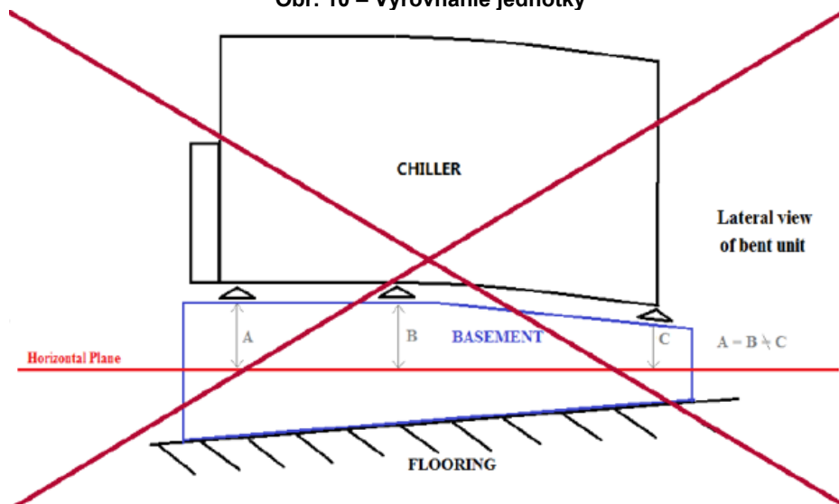
Obr. 10 – Vyrovnanie jednotky
