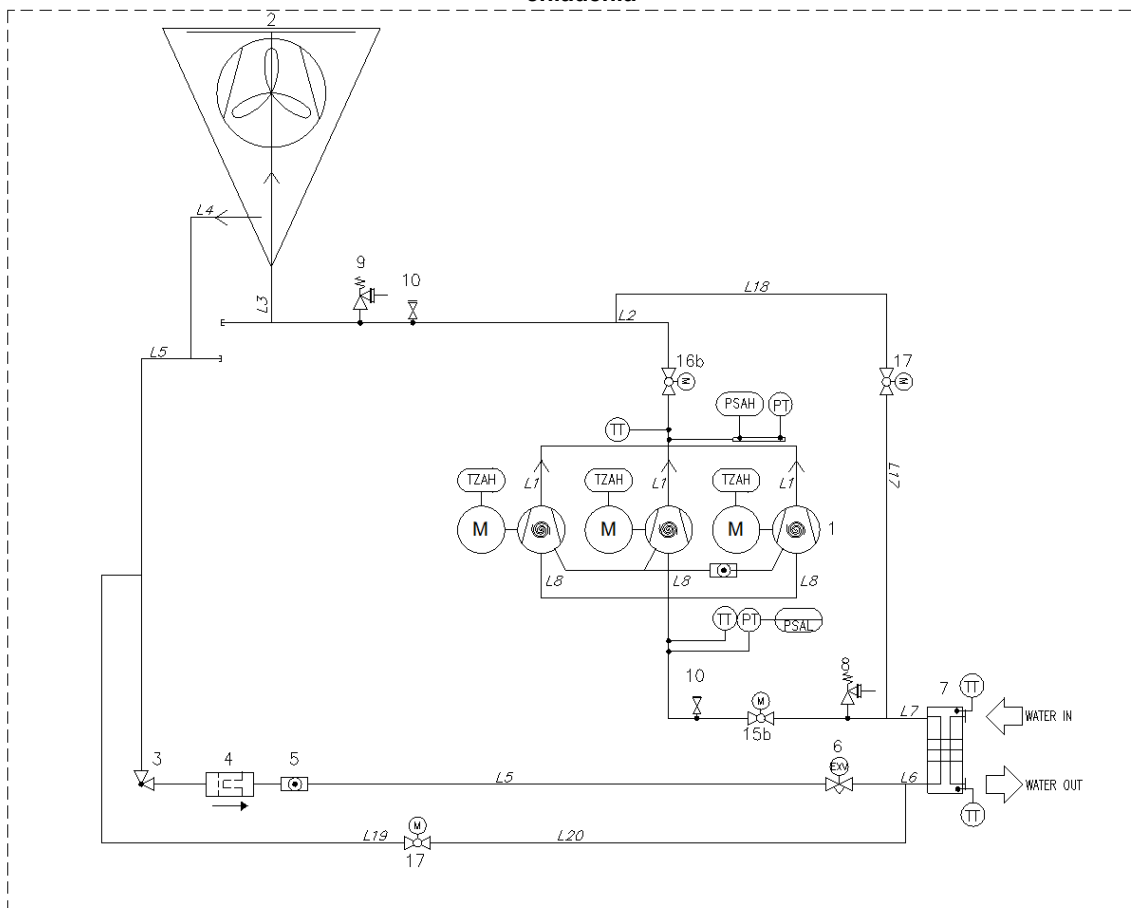
Obr. 2 – Schéma chladiaceho okruhu (P&ID) s jednookruhovým zariadením s možnosťou ľahkého voľného chladienia
