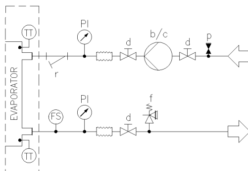
Obr. 15 – Hydraulická schéma pre samostatné čerpadlo Single V (EWATxx5B) (vol. 78-79/134-135) (max. prevádzkový tlak 6 barov)
