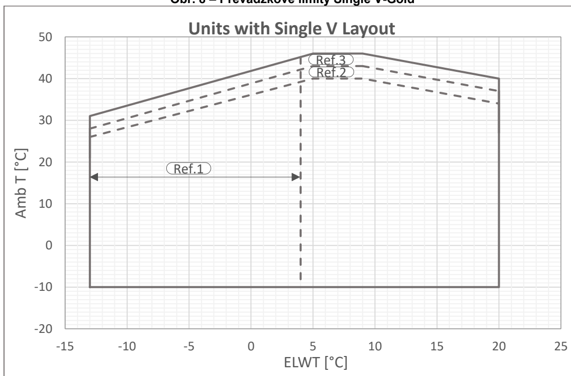
Obr. 8 – Prevádzkové limity Single V-Gold
