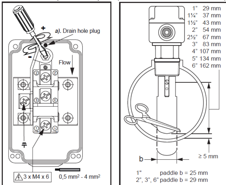
Obr. 13 Nastavenie prietokového spínača (model F61TB-9100 – Johnson Controls)
