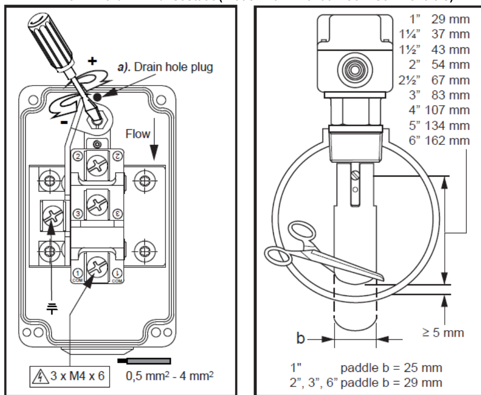
Fik. 13 – Akordimi i fluksostatit (modeli F61TB-9100 – Johnson Controls)
