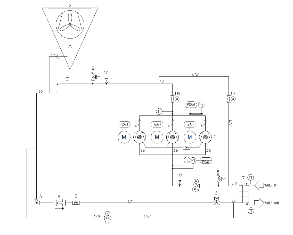
Fik. 2 – Diagrami i qarkut të ftohësit (P&ID) me njësi me një qark të vetëm me opsion ftohjeje të lirë
