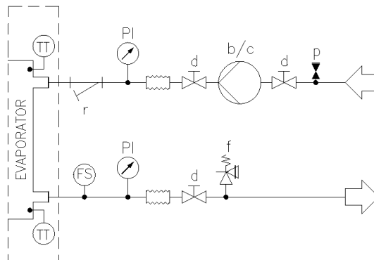
Fik. 15 – Diagrami hidraulik për pompën e vetme V (EWATxx5B) të vetme (opt. 78-79/134-135) (presioni maksimal i funksionimit 6 bar)
