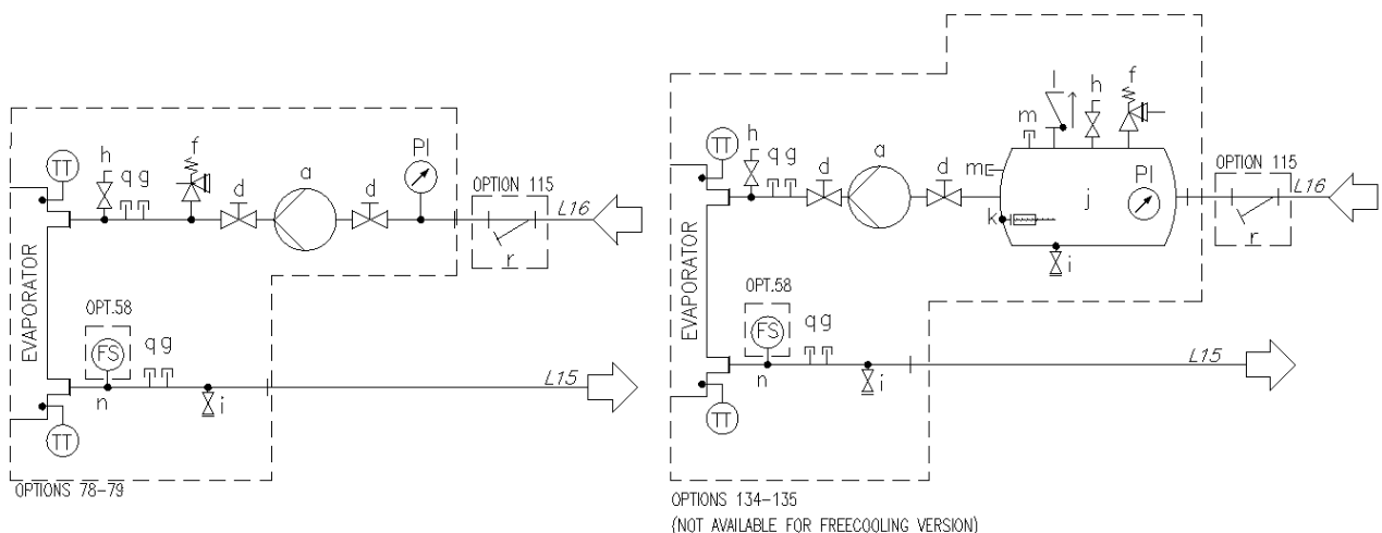
Fik. 15 – Diagrami hidraulik për pompën e vetme V (EWATxx5B) të vetme (opt. 78-79/134-135) (presioni maksimal i funksionimit 6 bar)
