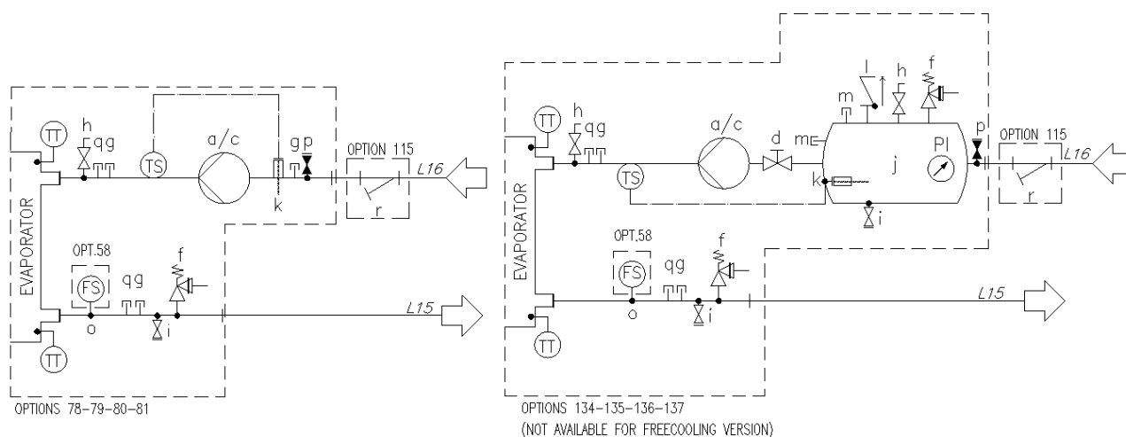
Fig. 17 – Hydrauliskt diagram för modulär V (EWATxx0B) (alt.78-79-80-81/134-135-136-137) (max arbetstryck 6 bar)
