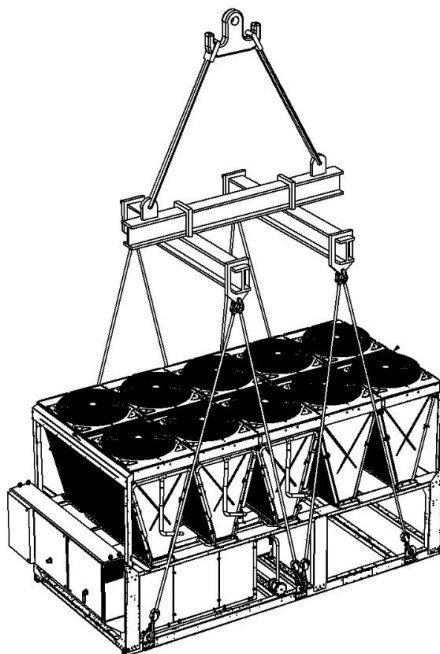
Enhet med sex lyftpunkter
