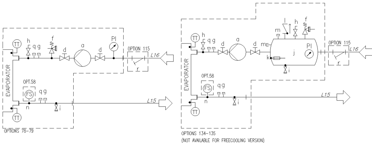
Fig. 15 – Hydraulisk diagram för enkel V (EWATxx5B) enkel pump (alt.78-79/134-135) (max arbetstryck 6 bar)
