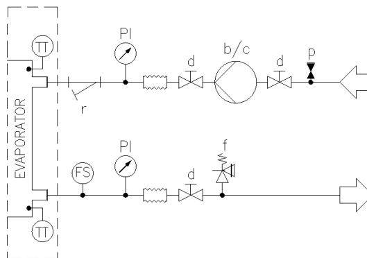
Fig. 15 – Hydraulisk diagram för enkel V (EWATxx5B) enkel pump (alt.78-79/134-135) (max arbetstryck 6 bar)
