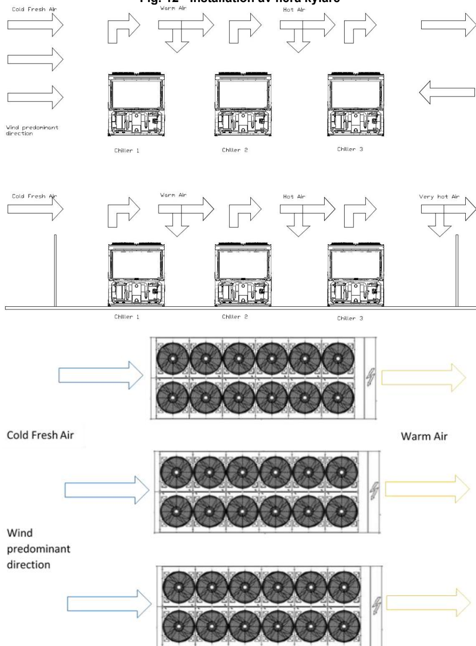
Fig. 12 - Installation av flera kylare
