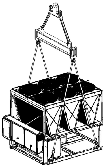
Enhet med fyra lyftpunkter
