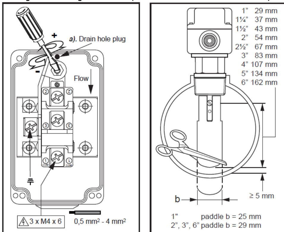
Fig. 13 – Justering av flödesvakt (modell F61TB-9100 – Johnson Controls)
