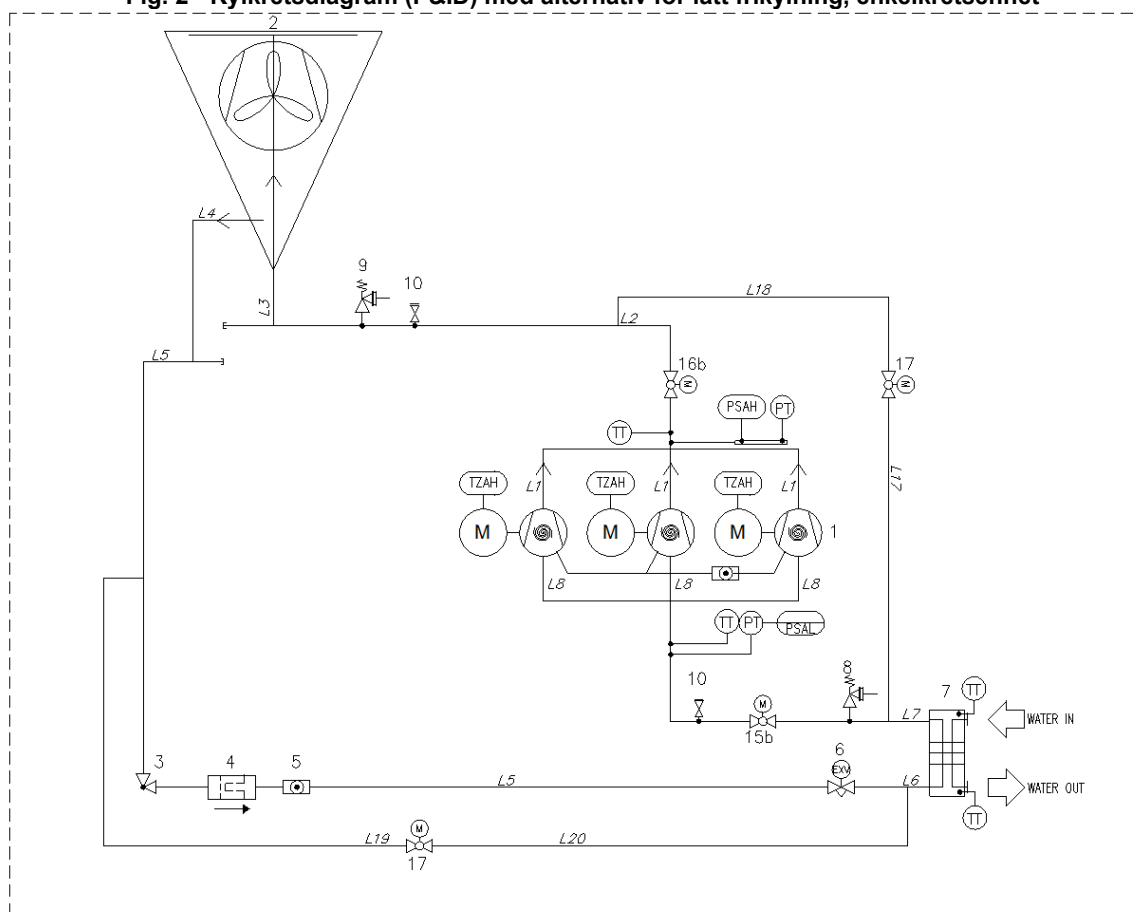
Fig. 2 - Kylkretsdiagram (P&ID) med alternativ för lätt frikylning, enkelkretsenshet
