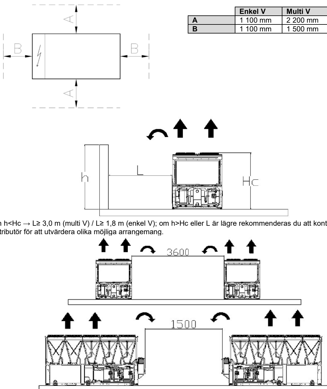
Fig. 11 - Krav på minsta utrymme
