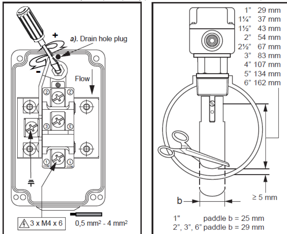
Рис. 13 – Налаштування реле потоку (модель F61TB-9100 – Johnson Controls)
