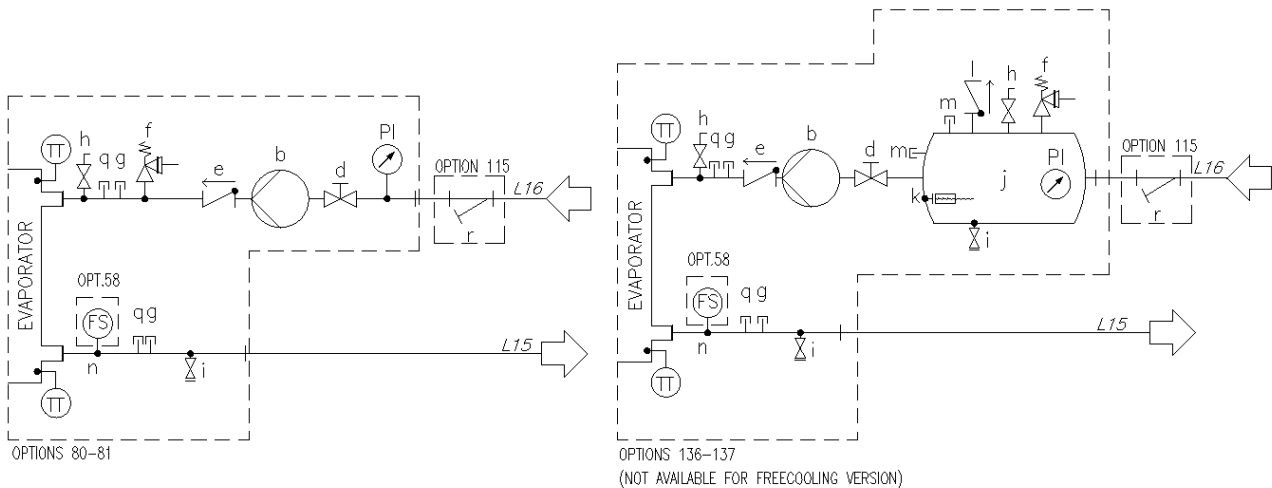
Рис. 17. Гідравлічна схема мультисекційного агрегату (EWATxx0B) (компл. 78-79-80-81/134-135-136-137) (макс. робочий тиск 6 бар)
