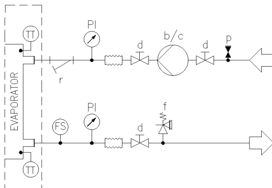
Рис. 15. Гідравлічна схема односекційного агрегату (EWATxx5B) з одним насосом (компл. 78-79/134-135) (макс. робочий тиск 6 бар)
