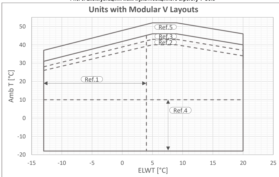
Рис. 6. Експлуатаційні межі мультисекційного агрегату V-Gold
