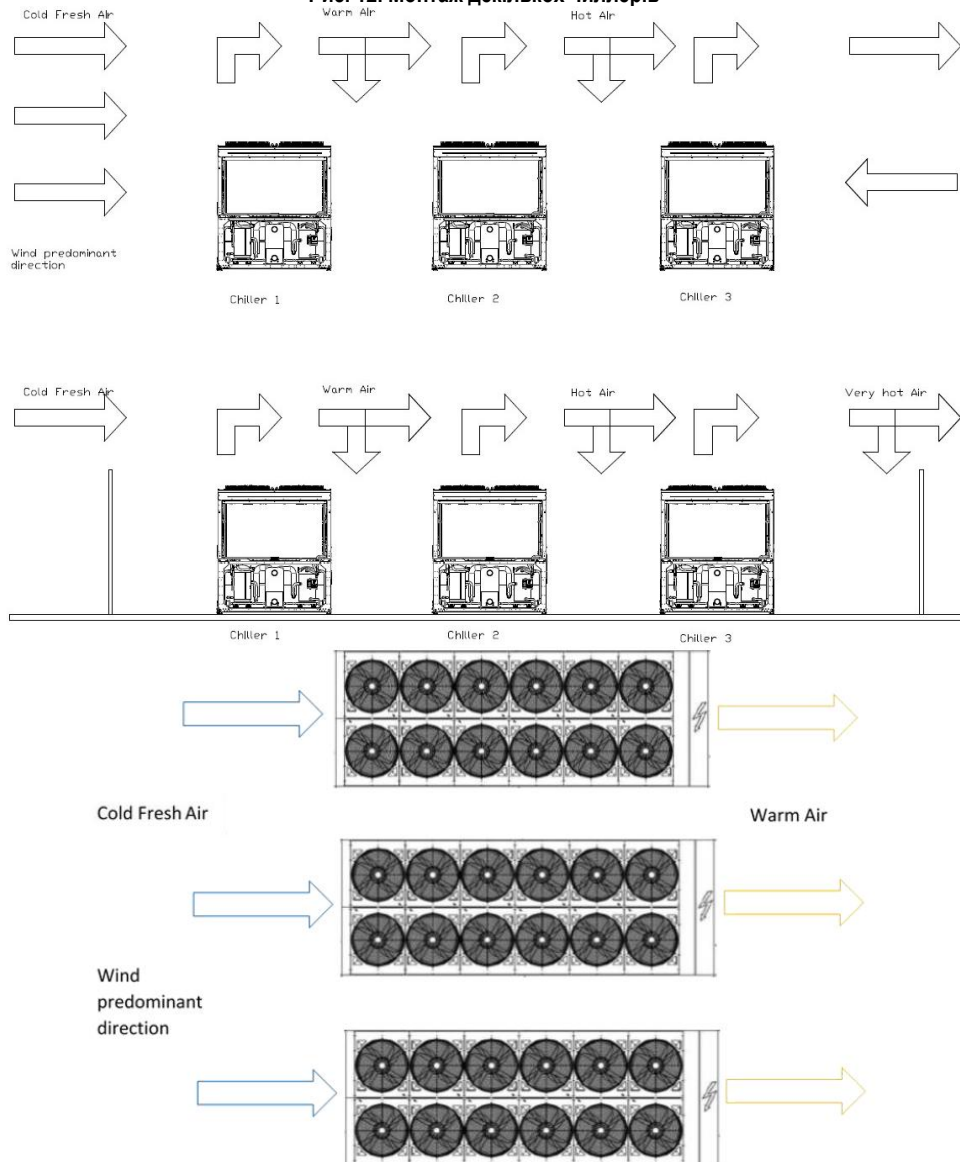
Рис. 12. Монтаж декількох чиллерів
