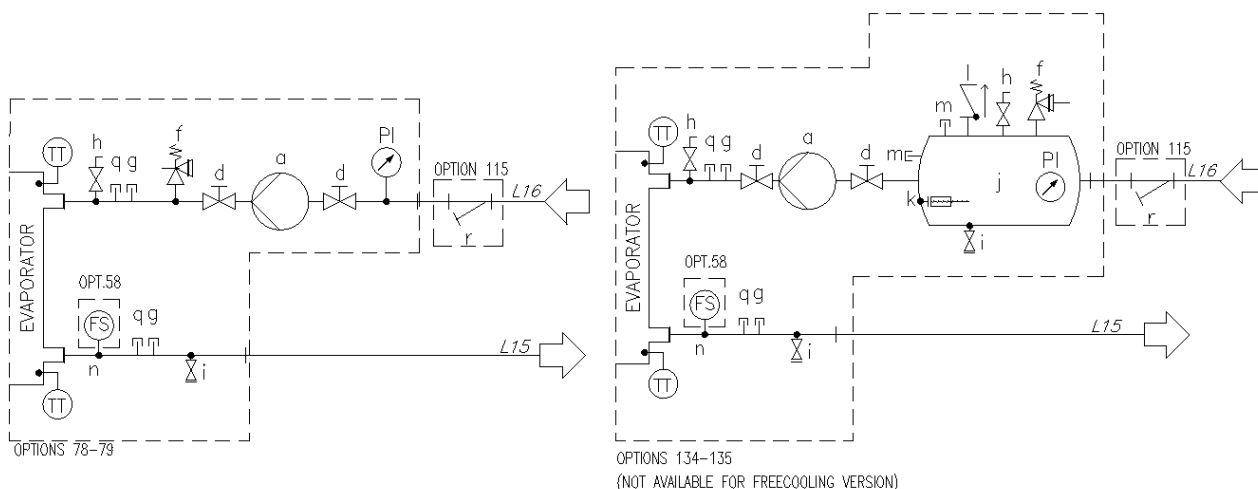
Рис. 15. Гідравлічна схема односекційного агрегату (EWATxx5B) з одним насосом (компл. 78-79/134-135) (макс. робочий тиск 6 бар)
