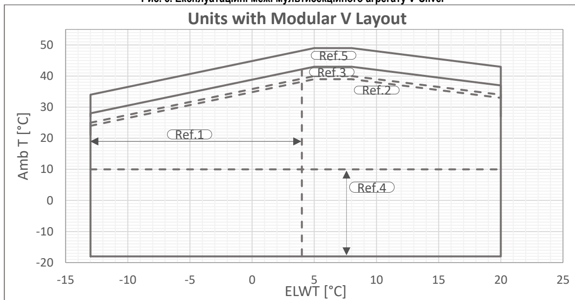
Рис. 6. Експлуатаційні межі мультисекційного агрегату V-Gold
