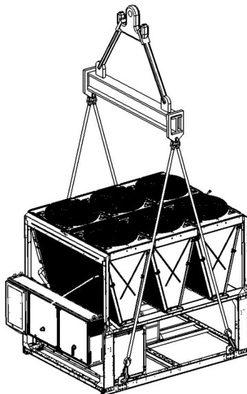
Рис. 9. Інструкції з підйому
