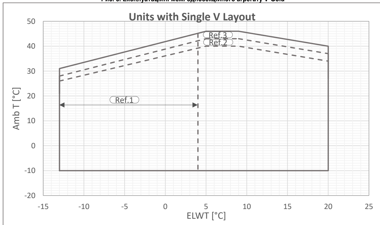
Рис. 8. Експлуатаційні межі односекційного агрегату V-Gold
