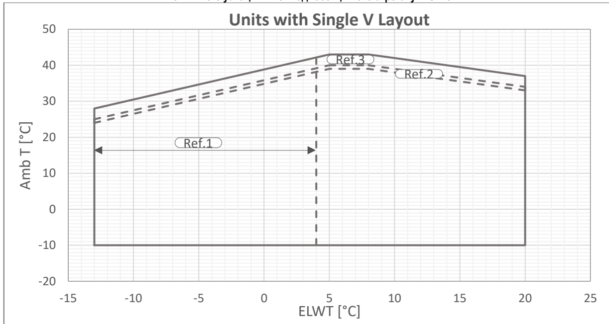
Рис. 8. Експлуатаційні межі односекційного агрегату V-Gold
