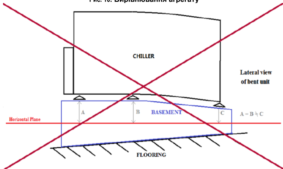
Рис. 10. Вирівнювання агрегату
