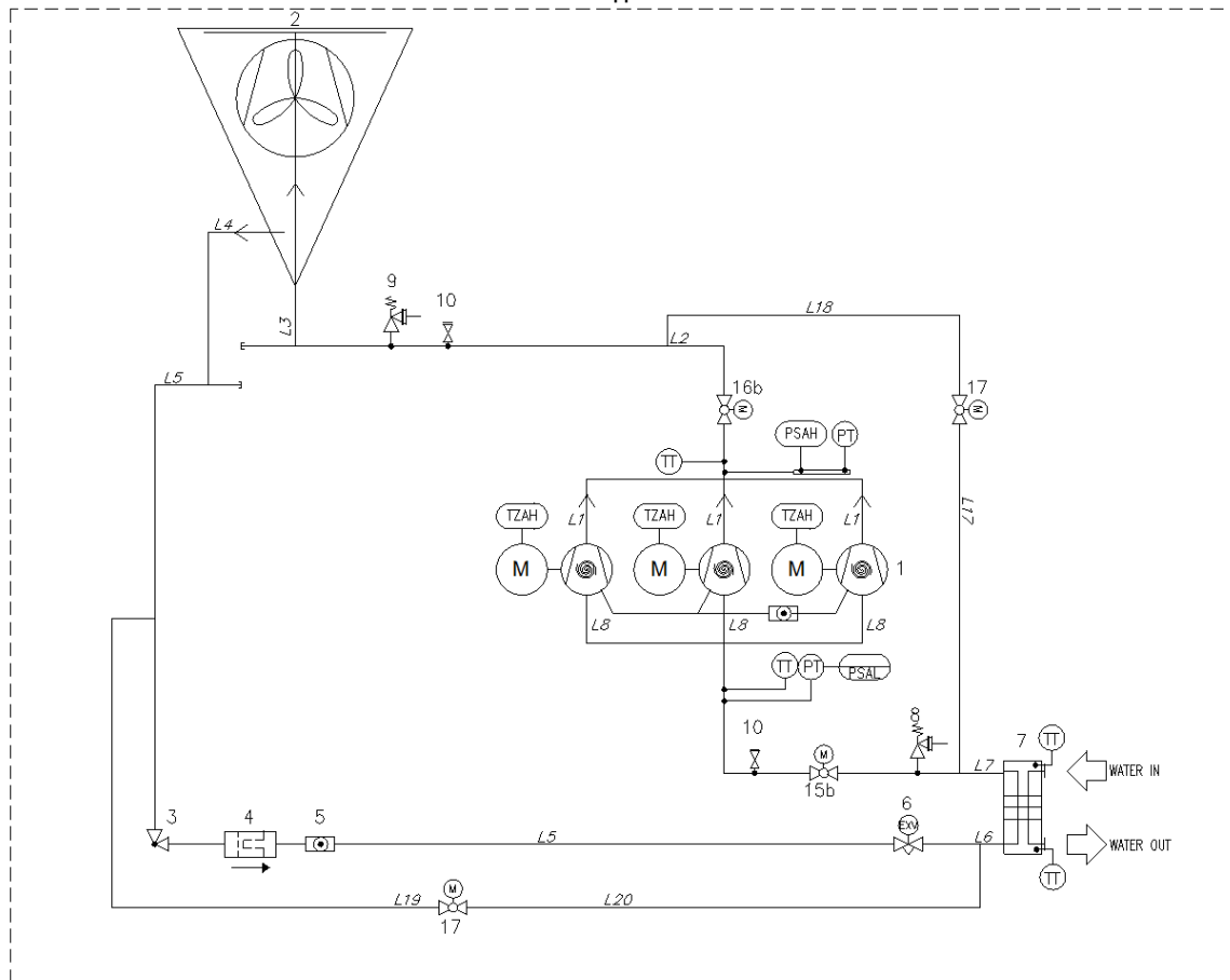
Рис. 2. Схема контуру холодоагенту (схема трубопроводів і КВП) для типового одноконтурного агрегату з частковим природним охолодженням
