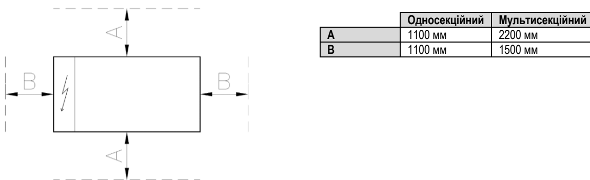
Рис. 11. Мінімальні вимоги до відстані
