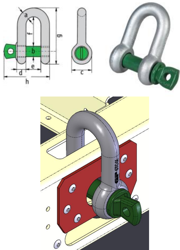
Fig. 10 - Fijación de los grilletes de elevación
