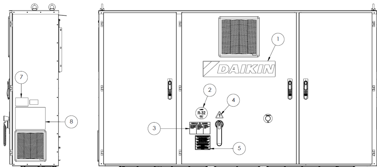
Fig. 23– Descripción de las etiquetas aplicadas al panel eléctrico medio
