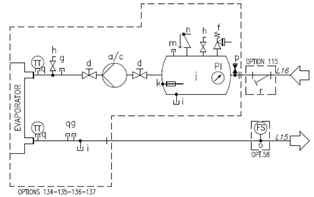
Fig. 19– Diagrama hidráulico (opt. 78-79-80-81/134-135-136-137)
