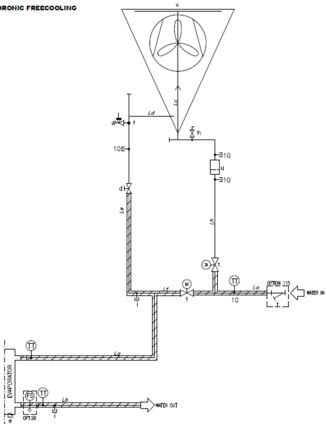
Fig. 3– Diagrama de circuito de refrigerante (P & ID) con unidad de circuito simple con freecooling
