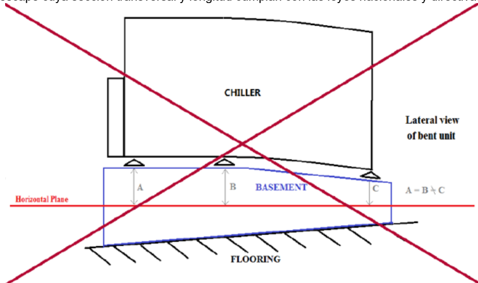
Fig. 13– Nivelación de unidades
