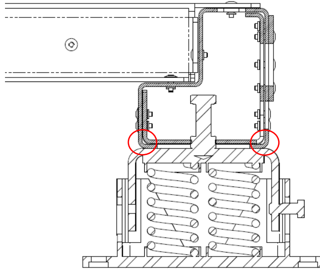
Kuva 20- Värinänvaimennuselementtien asentaminen (toimitetaan lisävarusteena)
