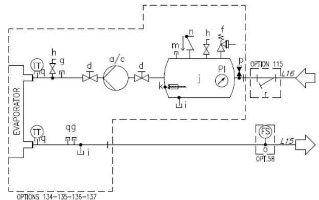
Kuva 24- Hydraulikaavio (lisävaruste 78-79-80-81/134-135-136-137)
