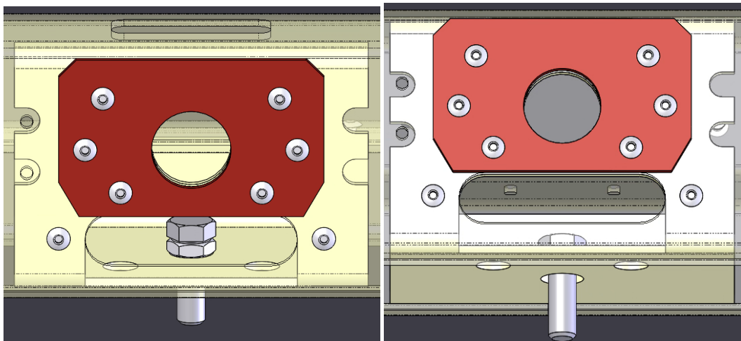
Kuva 21- Värinänvaimentimen kiinnitysruuvien yksityiskohdat
