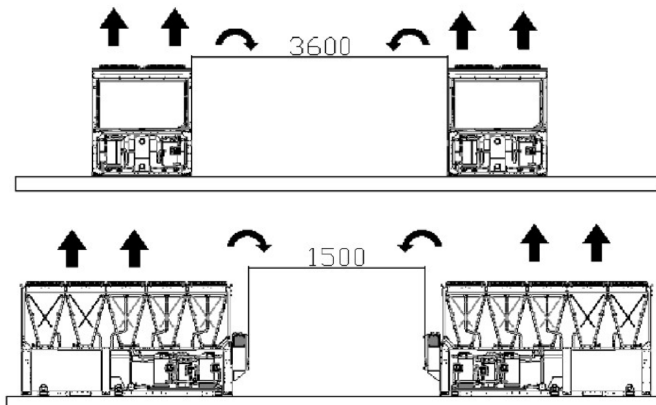
Kuva 16- Vähimmäistilavaatimukset
