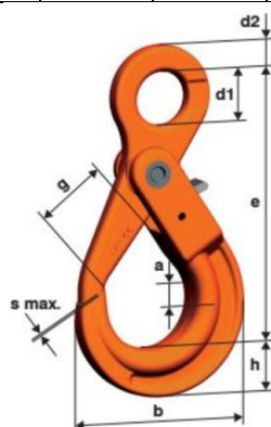
Kuva 9- Nostokoukun ominaisuudet
