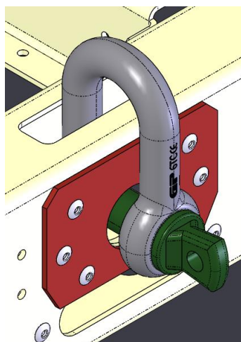
Fig. 10- Fixation des manilles de levage
