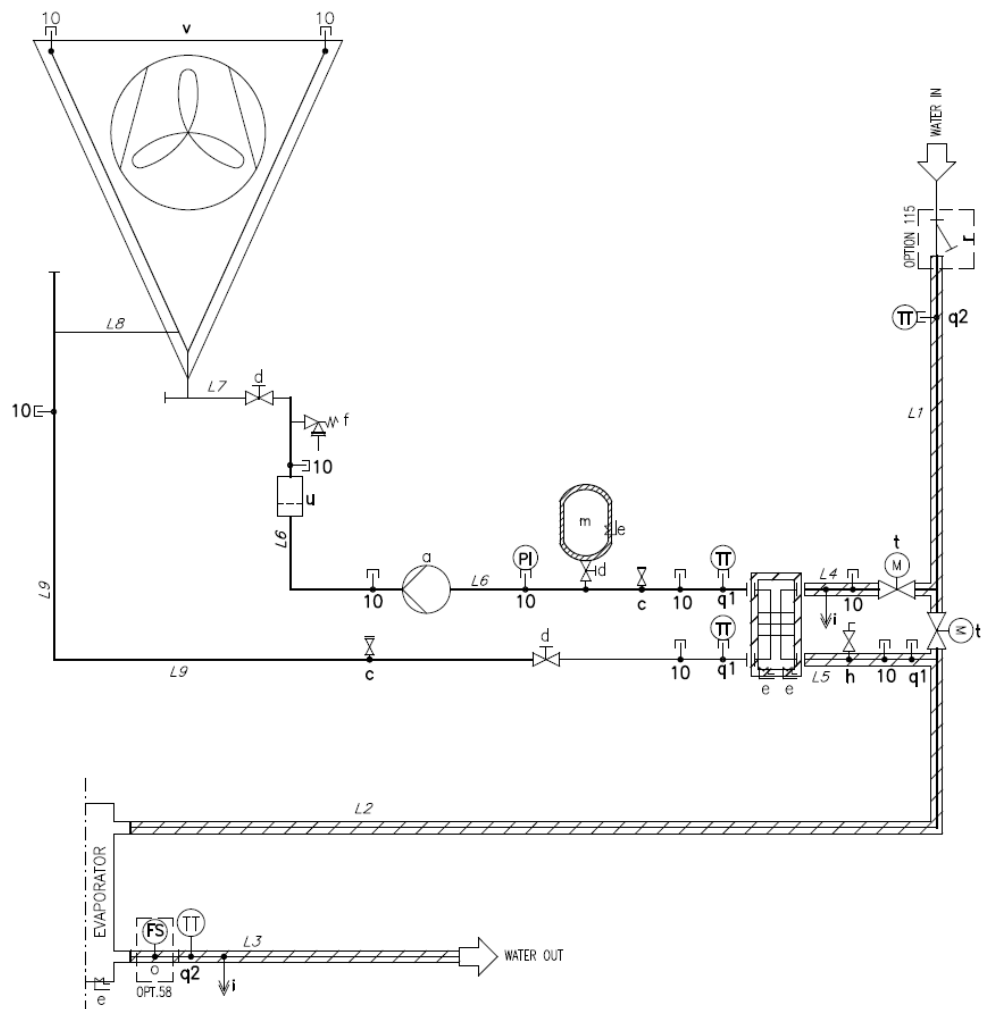
Fig. 21– P&ID del Free cooling idronico a ciclo chiuso (Opt. 231)
