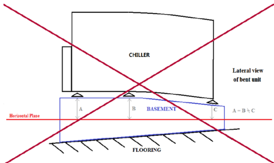
Fig. 13– Livellamento unità
