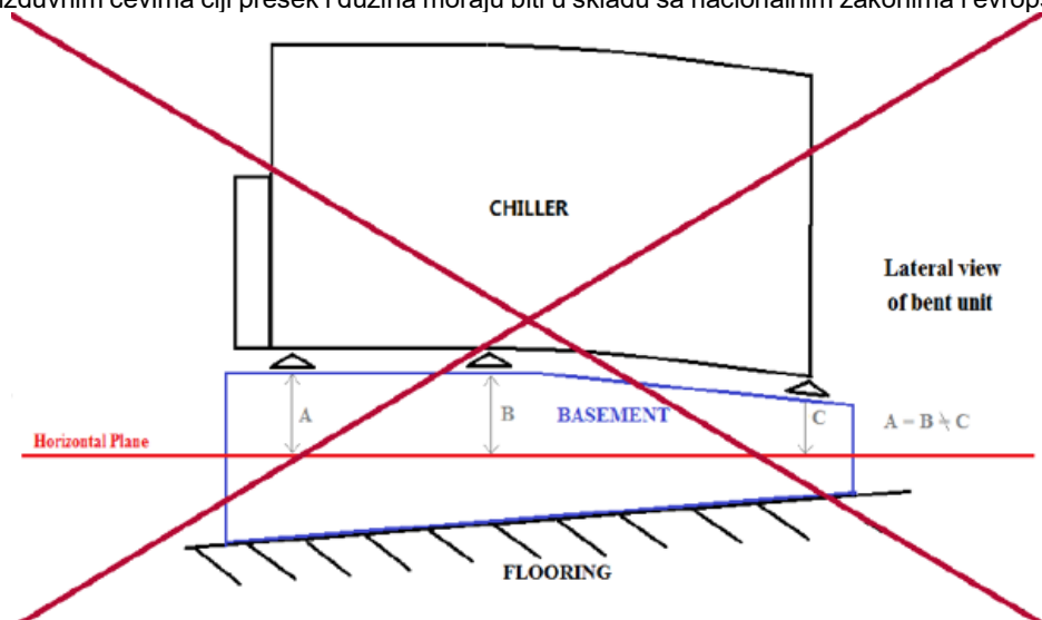
Sl. 15- Nivelisanje jedinice
