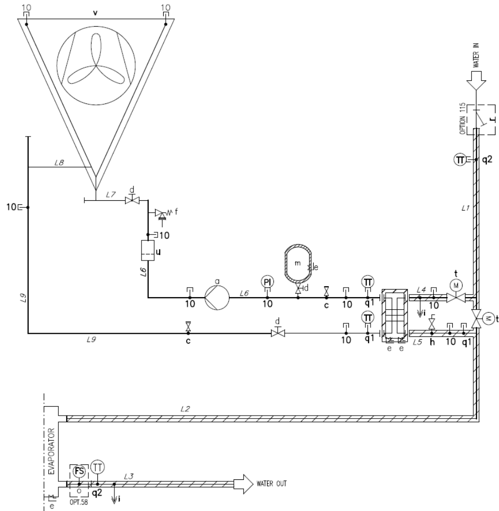
Fig. 26- Hydronisk frikyla med sluten krets P&ID (Opt. 231)
