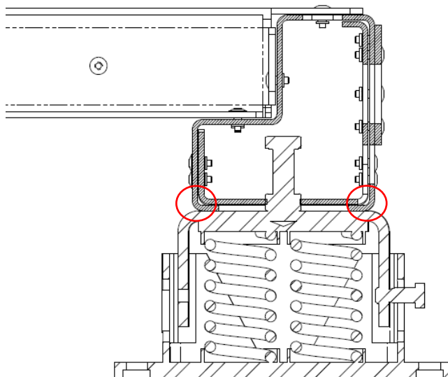
Fig. 20 - Montering av vibrationsdämpande element (levereras som tillval)
