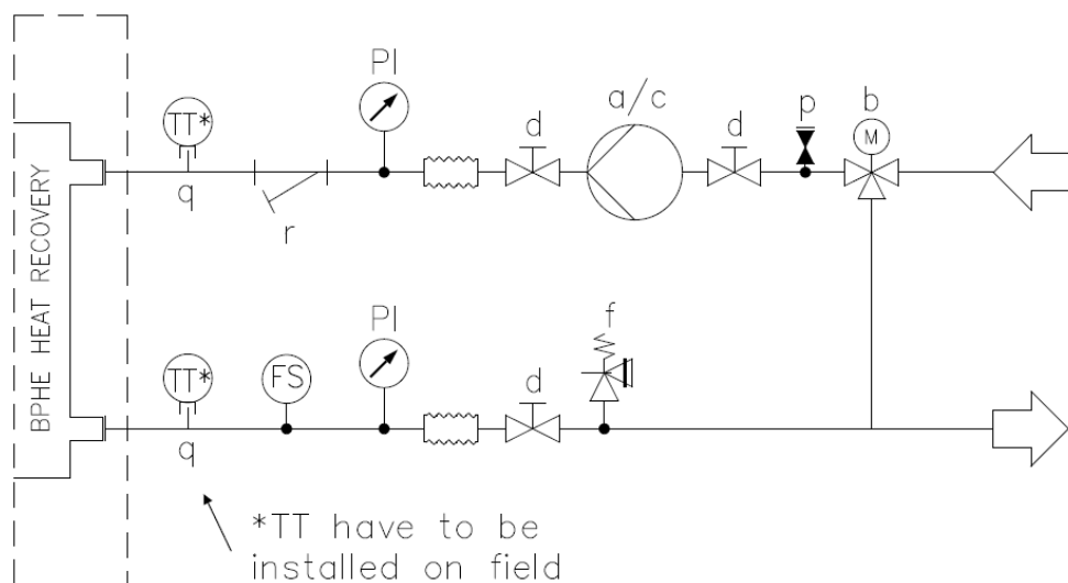
Fig. 25- Vattenledningens anslutning för värmeväxlarna för värmeåtervinning (max. tryck 20 bar)
