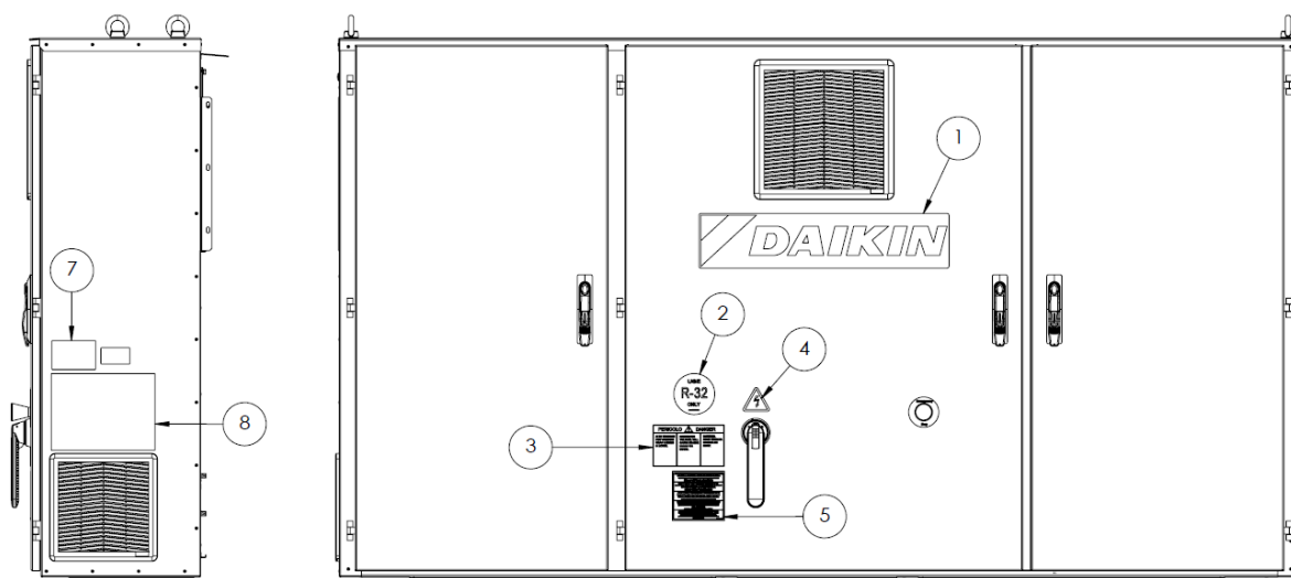
Fig. 27– Beskrivning av märkningarna applicerade på elpanelen liten.
