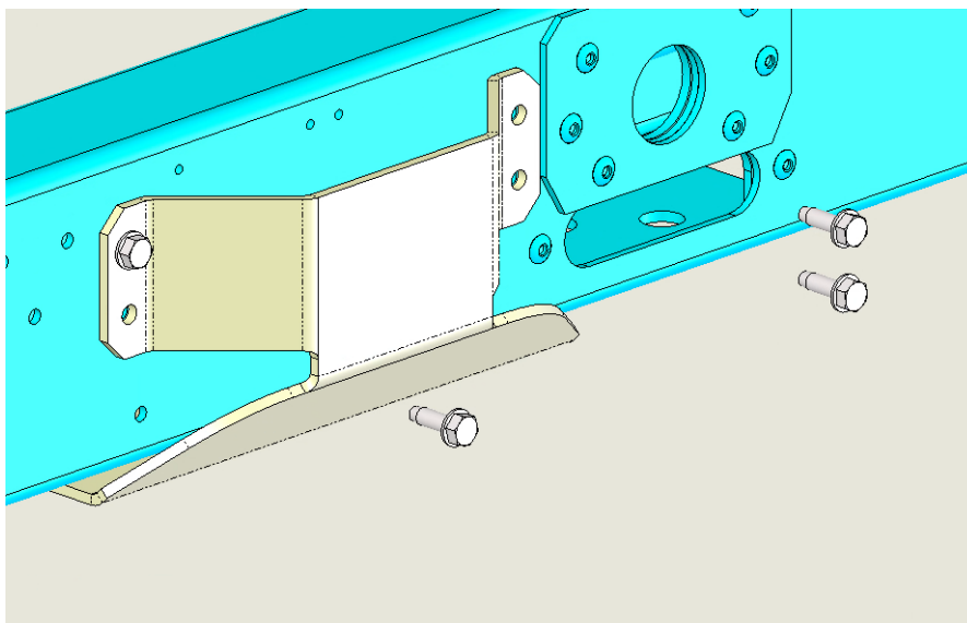
Fig. 14 – M8-bultar för anslutning av platta-enhetsram
