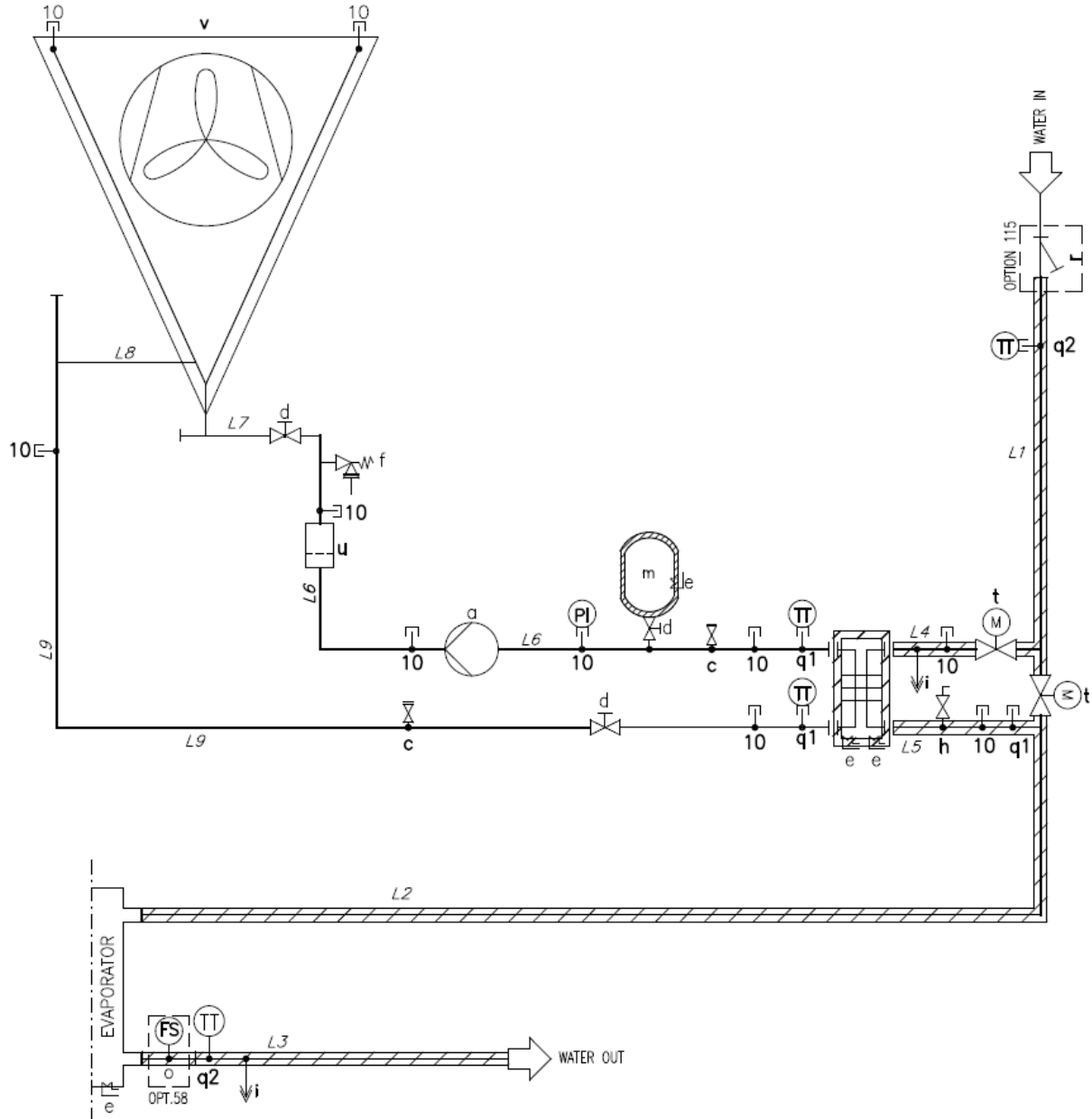
Kuva 26- Suljettu silmukka Hydroninen vapaa jäähdytys P&ID (lisävaruste 231)
