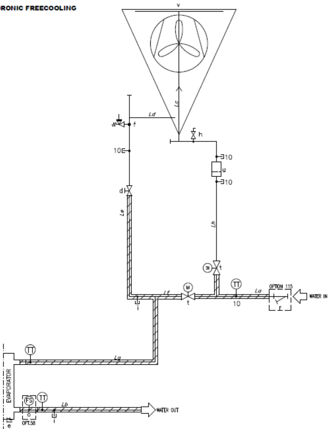
Fig. 3– Schéma du circuit d'eau (P&ID) du système de refroidissement naturel hydraulique
