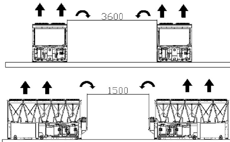
Fig. 14– Encombrement minimal
