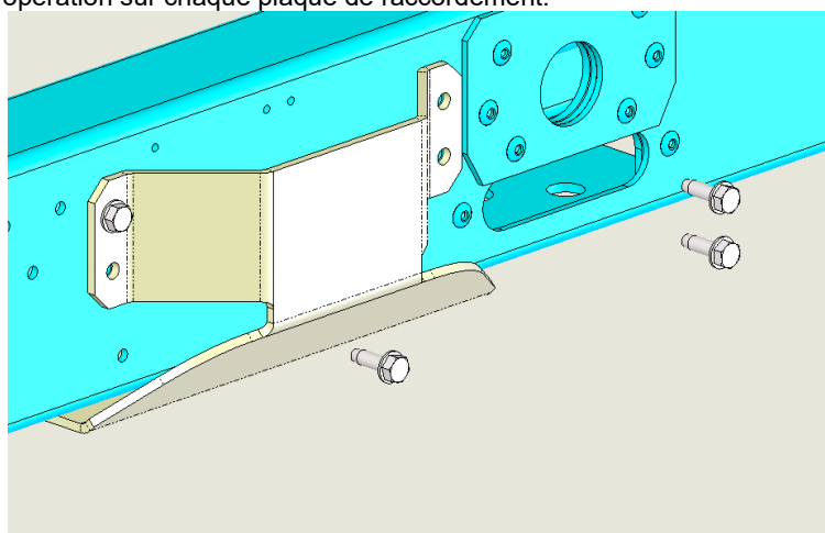
Fig. 12 – Boulons M8 pour le raccordement des plaques au châssis de l'appareil
