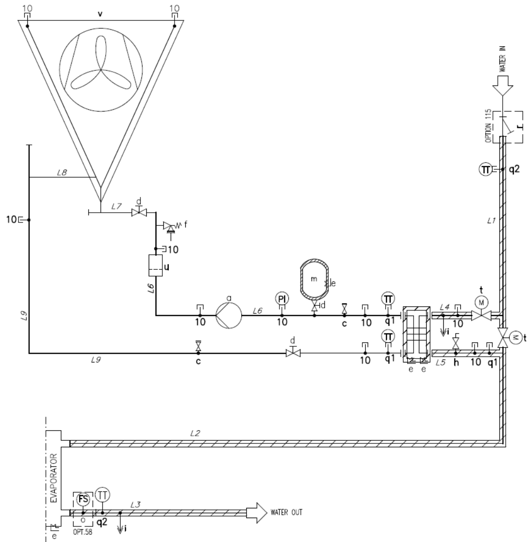
Fig. 21– Circuit fermé Hydronic Free cooling P&ID (Opt. 231)
