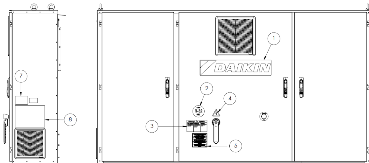
Fig. 23- Description des étiquettes appliquées sur le Table électrique (moyen)
