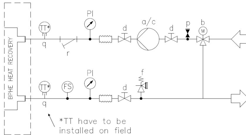
Fig. 20- Raccordement de la tuyauterie d'eau pour les échangeurs de récupération de chaleur (pression maximale de 20 bar)
