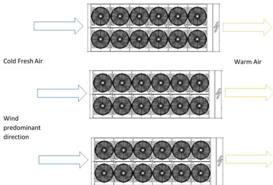
Fig. 15– Installazione di chiller multipli
