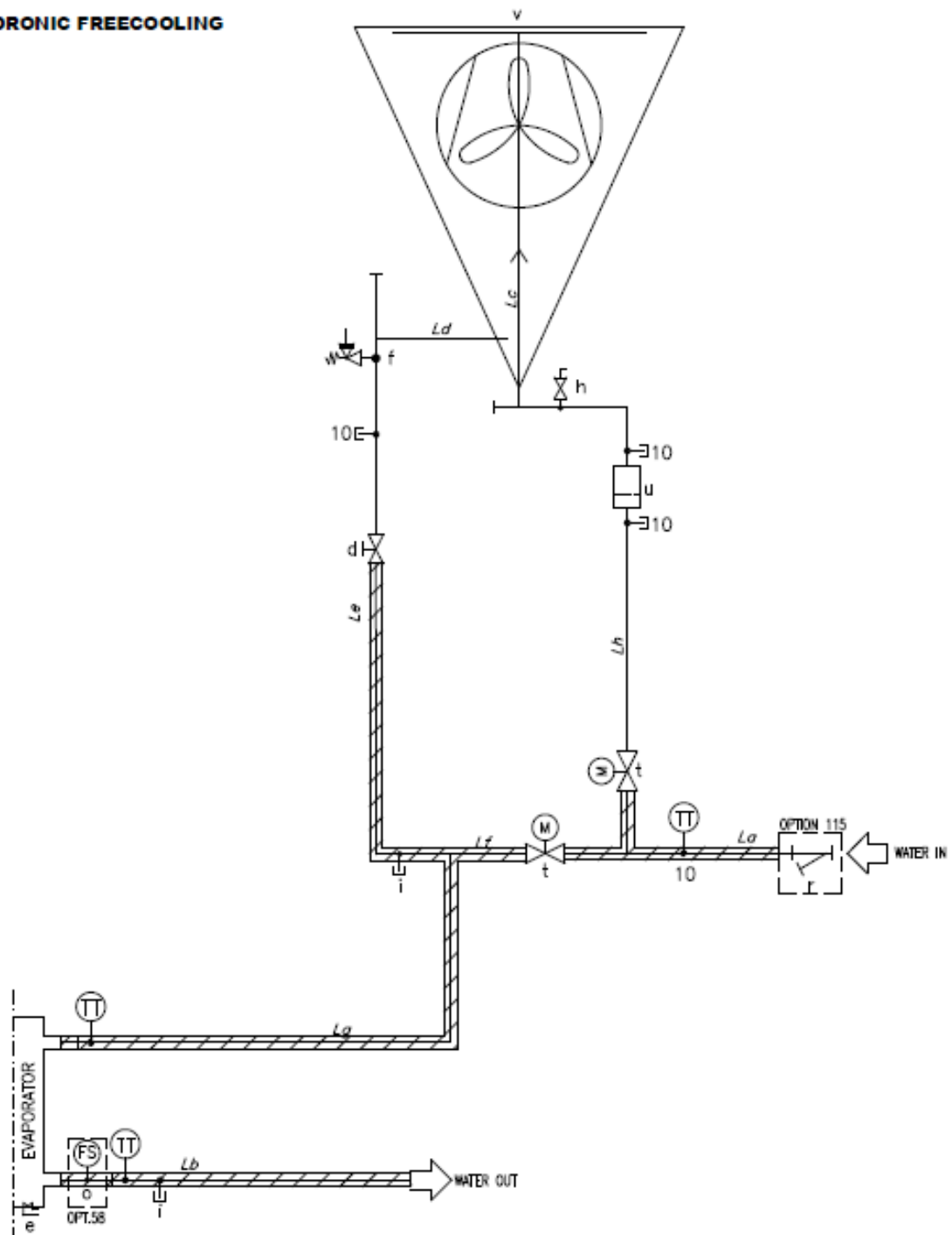
Fig. 3– Sistema idronico Freecooling (P&ID)
