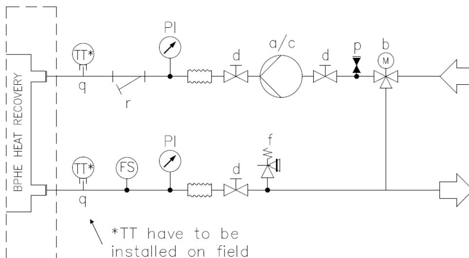
Fig. 20- Collegamento circuito dell'acqua per scambiatori con recupero di calore (pressione massima 20bar)
