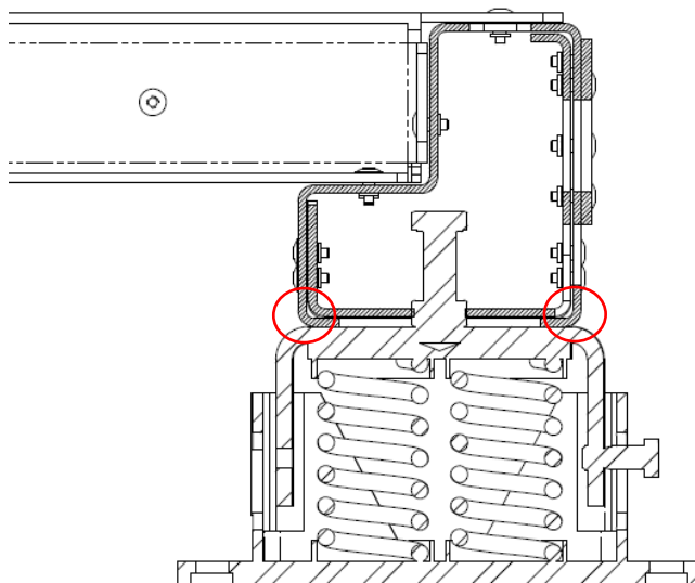
Fig. 18– Montaggio elementi antivibranti (forniti come optional)
