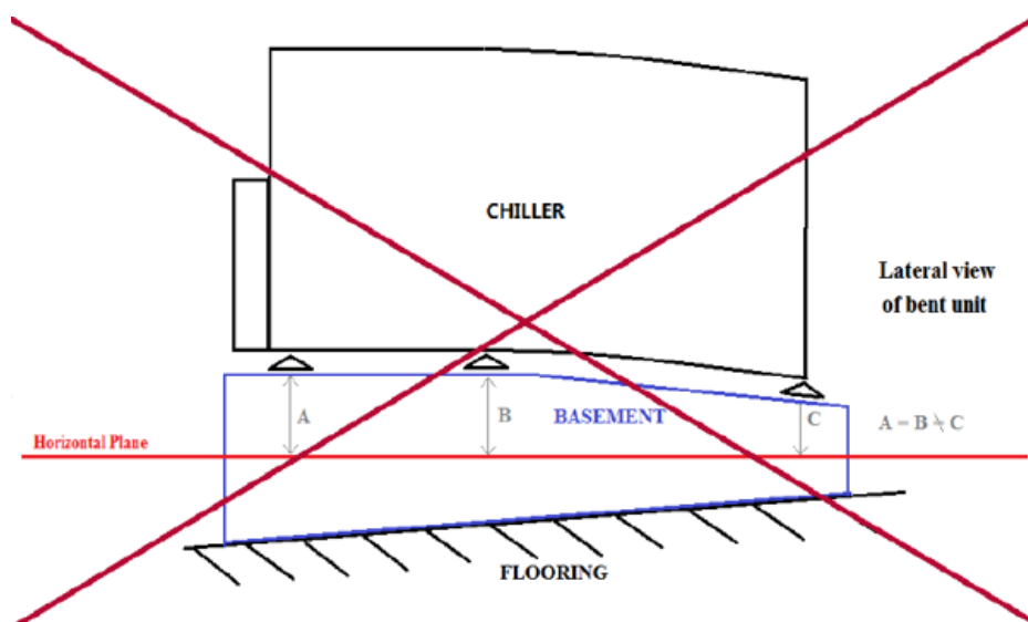
Fig. 13– Livellamento unità
