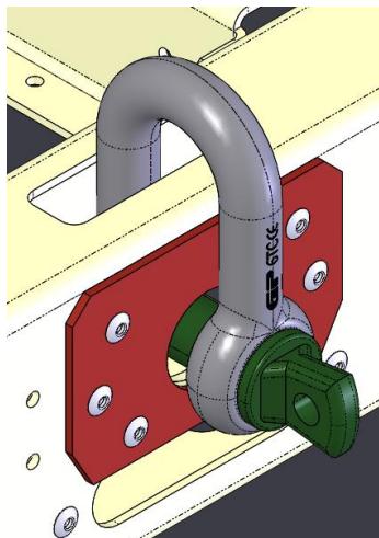
Fig. 10 - Fissaggio dei grilli di sollevamento
