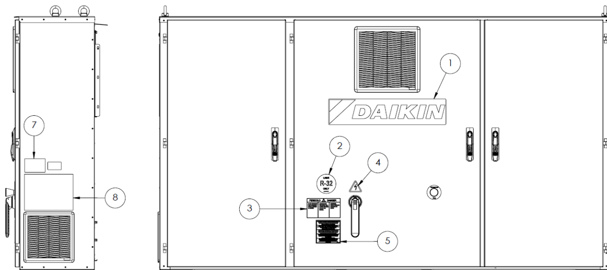
Fig. 23– Descrizione etichette applicate su quadro elettrico(medio)
