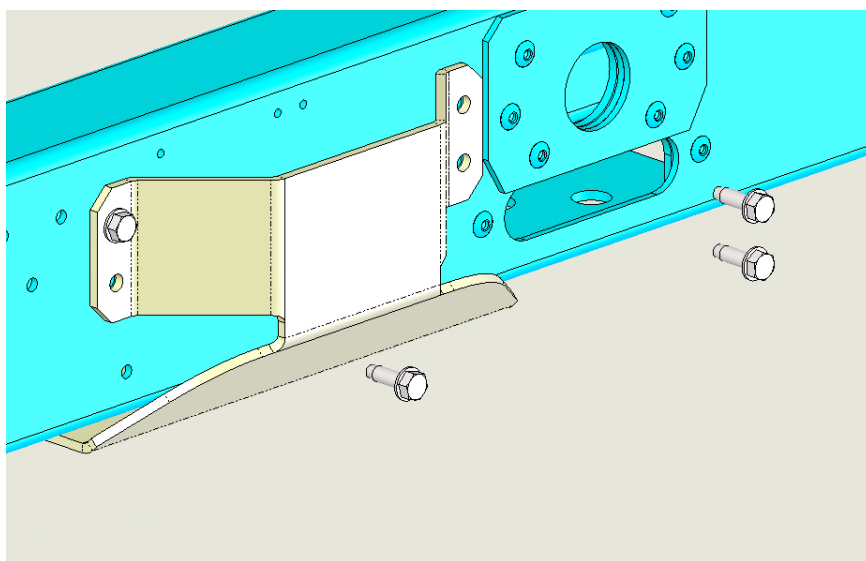
Fig. 12 - Viti M8 per accoppiamento lamiera-telaio
