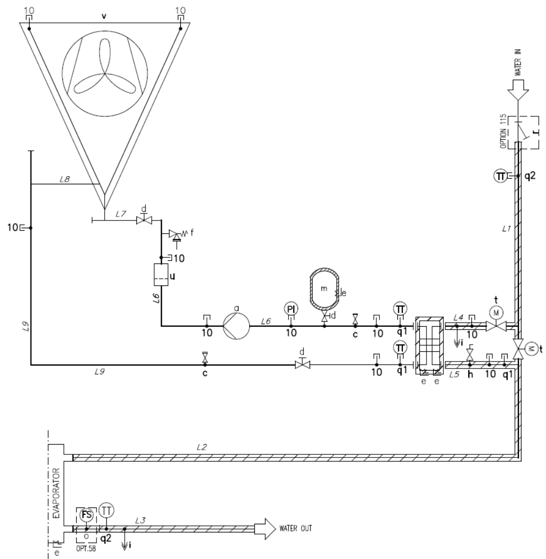
Fig. 21– P&ID del Free cooling idronico a ciclo chiuso (Opt. 231)
