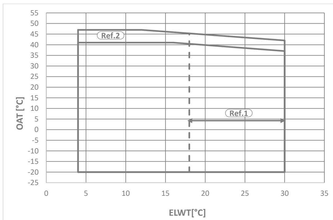
Fig. 6– EWFT-B-C Silver limiti di funzionamento
