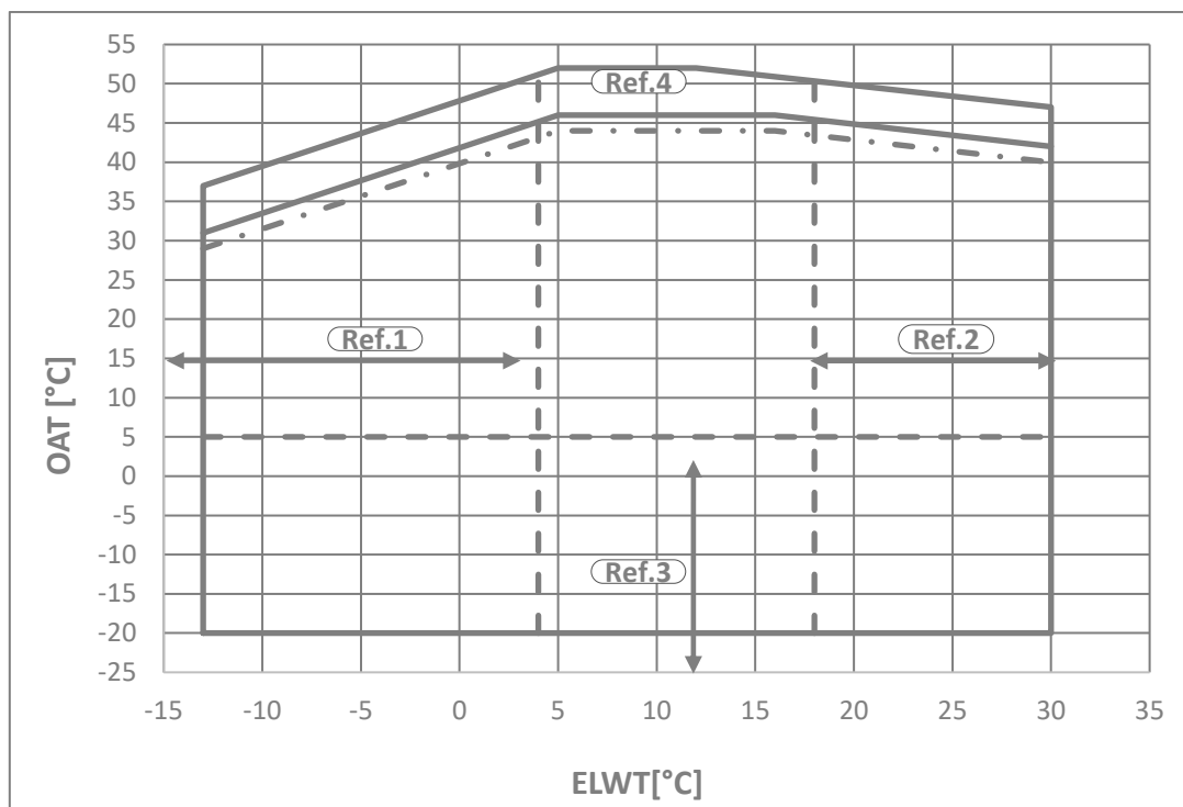
Fig. 5– EWAT-B-C Gold limiti di funzionamento
