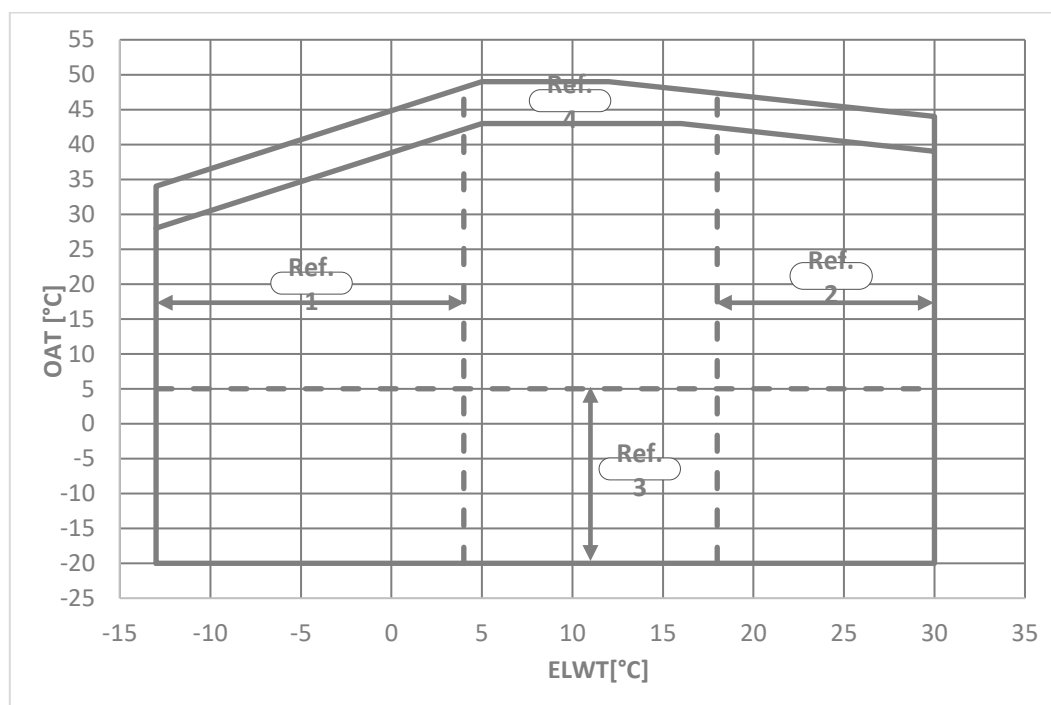
Fig. 4- EWAT-B-C Silver limiti funzionamento
