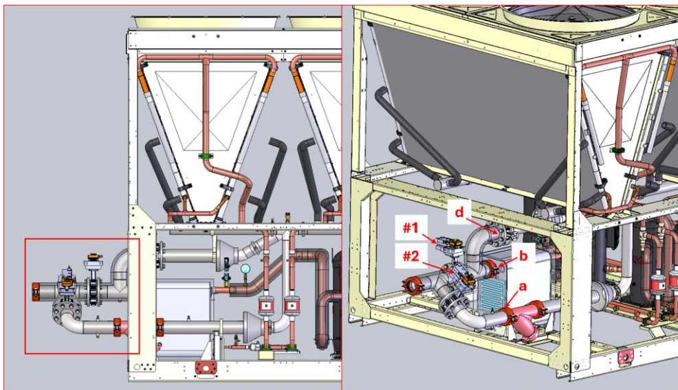
Fig. 17–Dettagli del l'installazione delle tubazioni.
