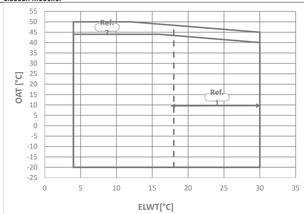
Fig. 7– EWFT-B-C Gold limiti di funzionamento
