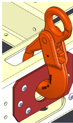
Fig. 9- Attacco del gancio di sicurezza
