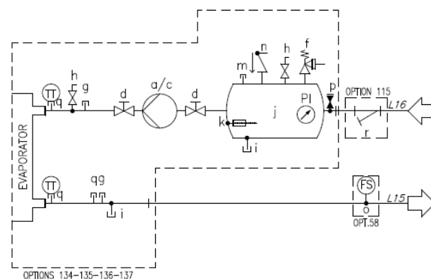
Fig. 19– Schema idraulico (opt. 78-79-80-81/134-135-136-137)
