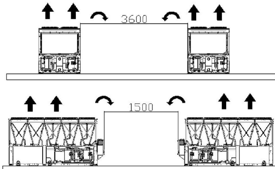
Fig. 14– Requisiti di spazio minimi
