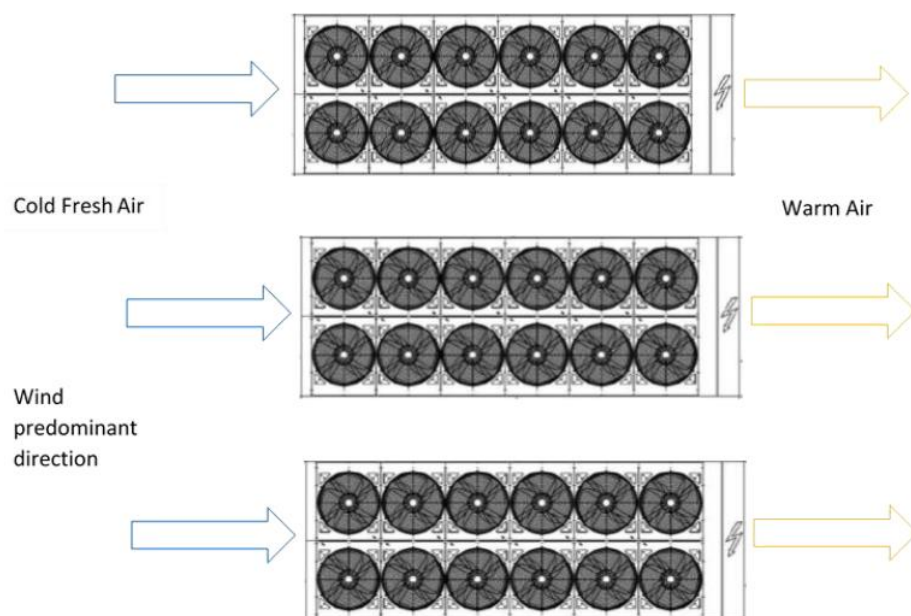
Fig. 15– Instalação de múltiplos refrigeradores
