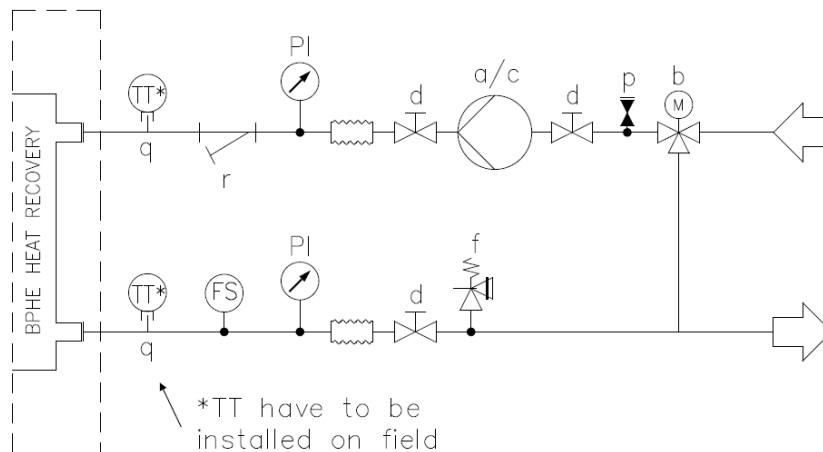
Fig. 20- Esquema hidráulico sem bomba(s) a bordo (pressão máxima de 20 bar)
