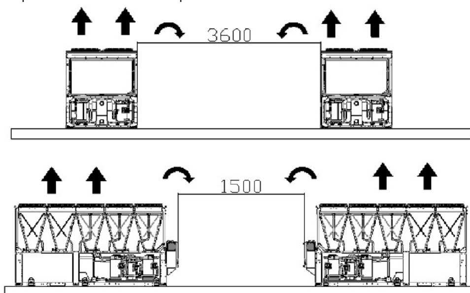
Fig. 14– Requisitos mínimos de espaço
