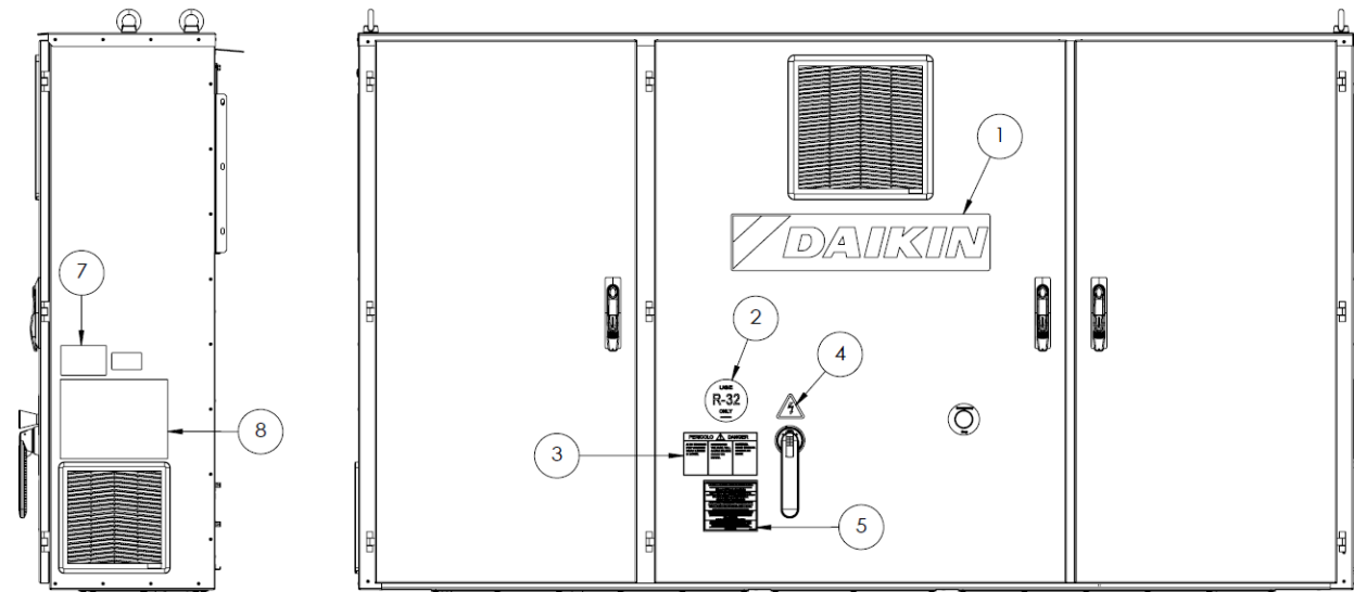
Fig. 22– Descrição das etiquetas aplicadas no painel elétrico (pequeno)
