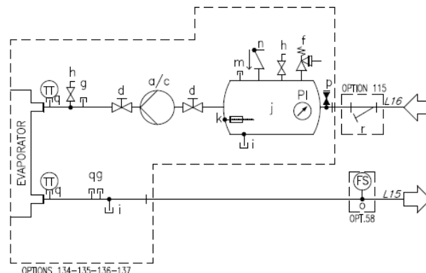
Fig. 19– Esquema hidráulico (opt. 78-79-80-81/134-135-136-137)
