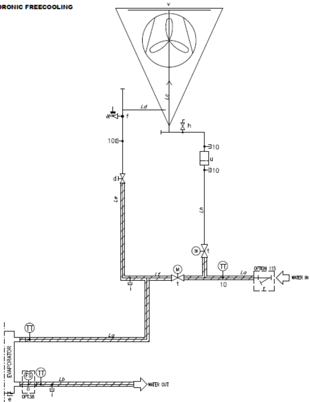
Fig. 3– Sistema hidráulico de arrefecimento livre (P&ID)
