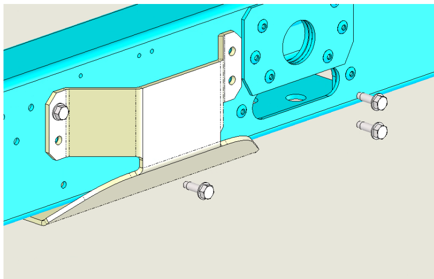
Fig. 12 – Parafusos M8 para ligação placa-estrutura da unidade
