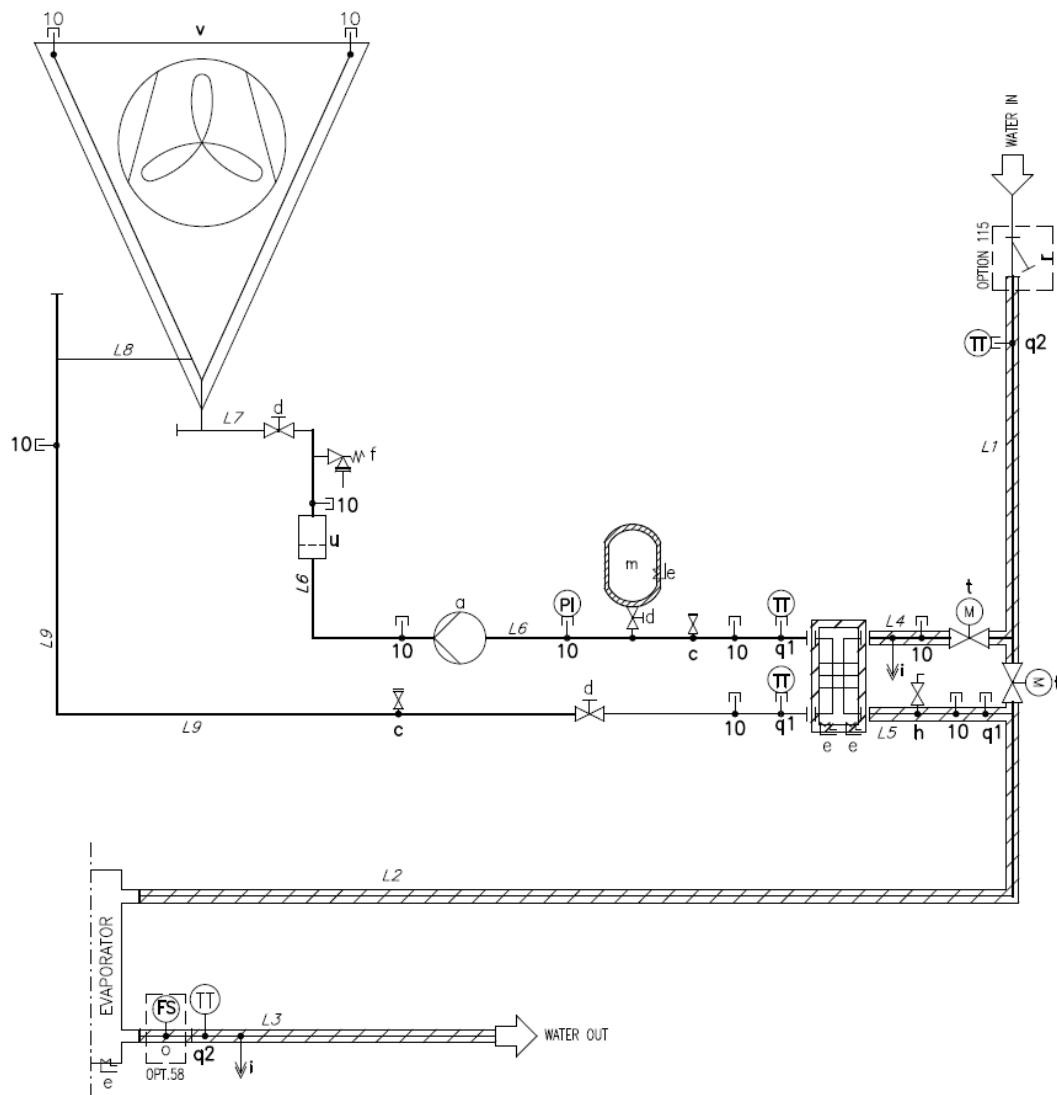
Fig. 21– Circuito fechado Hydronic Free cooling P&ID (Opt. 231)
