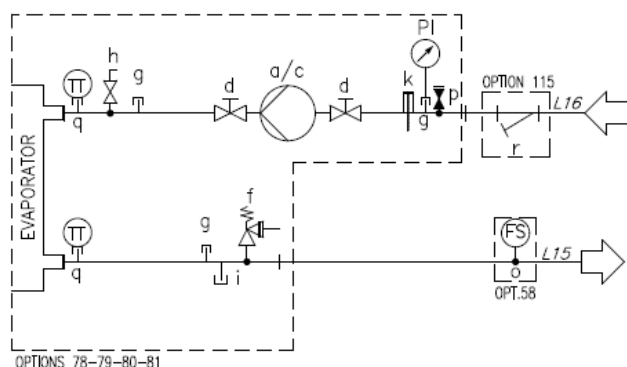
Fig. 19– Diagrama hidraulică (opt. 78-79-80-81/134-135-136-137)
