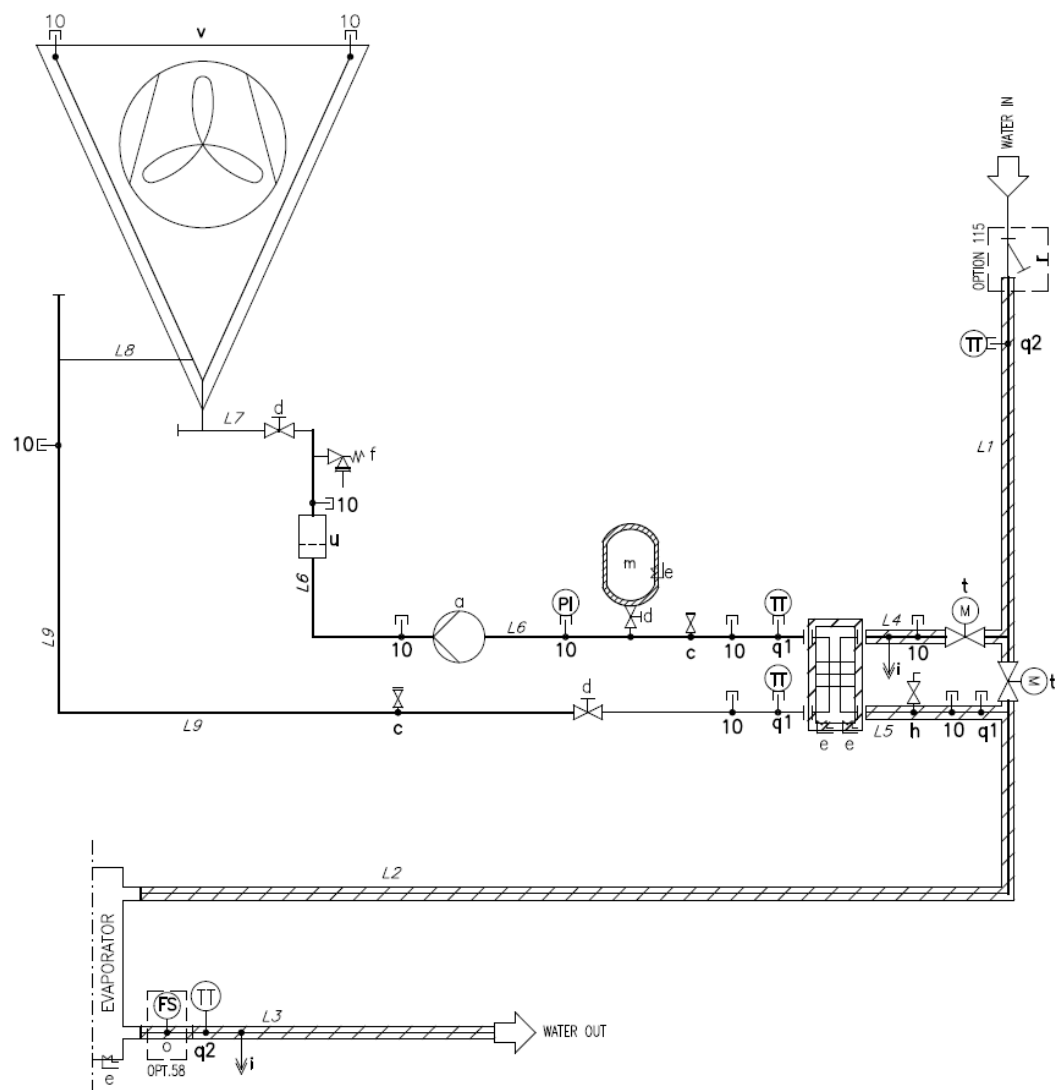
Fig. 21 - Buclă închisă Hidronic Răcire gratuită P&ID (Opt. 231)
