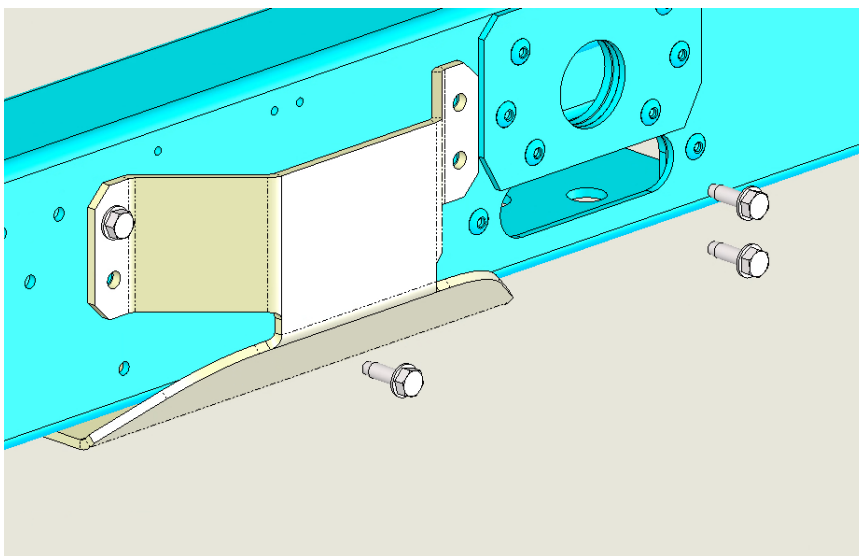
Fig. 12 – Șuruburi M8 pentru conectarea cadrului unității la placă
