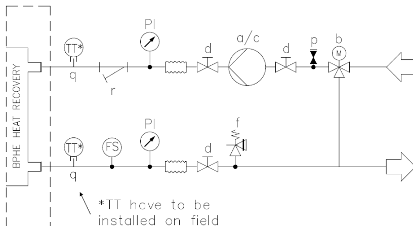
Fig. 20- Conectarea conductelor de apă pentru schimbătoarele de căldură (presiune maximă 20 bari)
