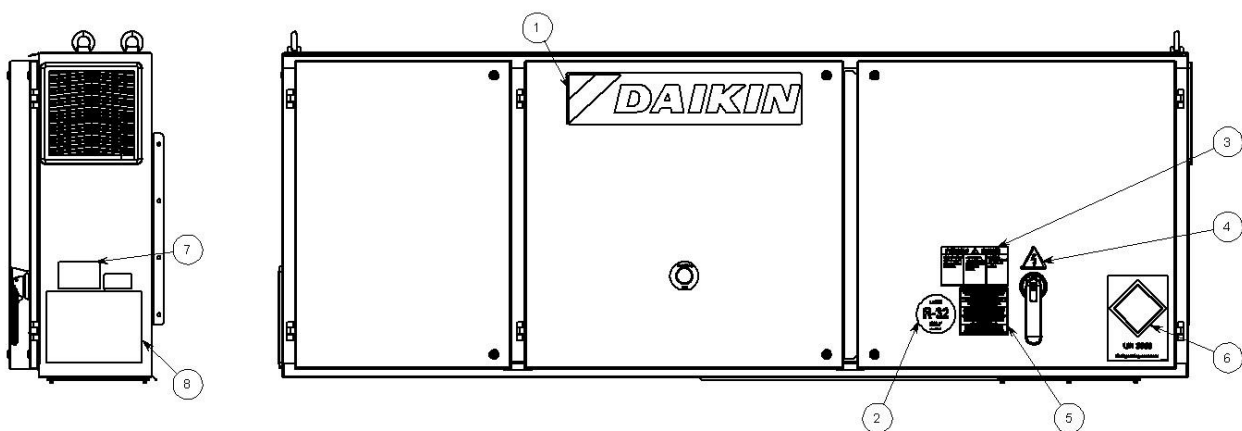
Obr. 27– Popis štítkov umiestnených na elektrickom paneli (malé)
