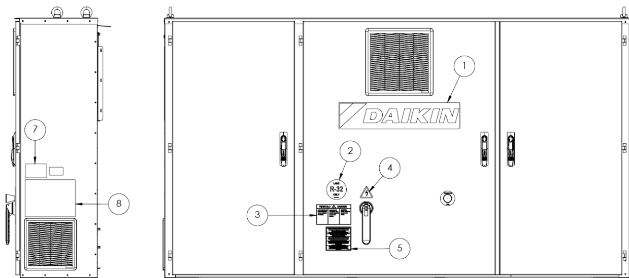
Slika 27– Opis nalepk, nameščenih na električni plošči
