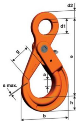
Slika 9– Značilnosti dvížnega kavlja
