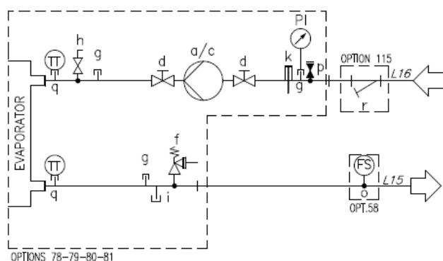
Slika 24– Hidravlični diagram (št. 78-79-80-81/134-135-136-137)
