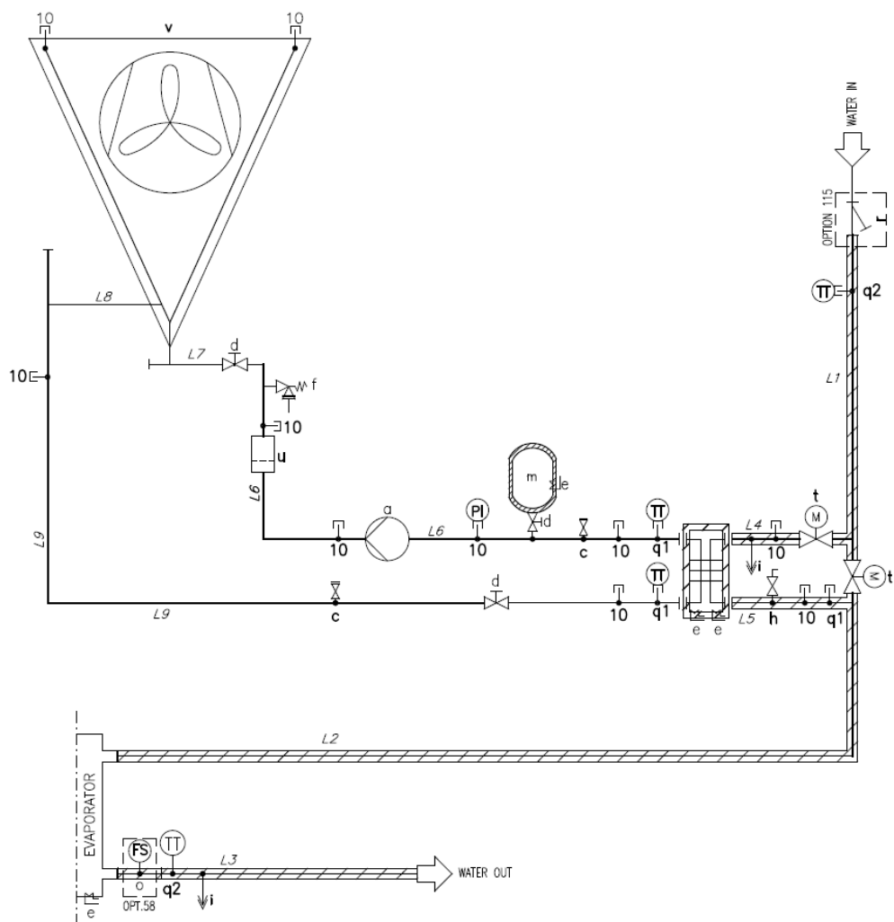
Slika 26 - Zaprta zanka hidroničnega prostega hlajenja P&ID (Opt. 231)
