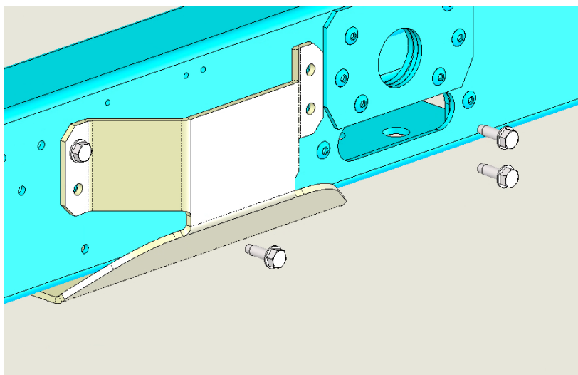
Slika 14 – Vijaki M8 za povezavo plošče in okvirja enote
