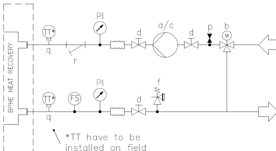
Slika 25- Prikluček vodovodnega cevovoda za izmenjevalnike toplote (najvišji tlak 20 bar)
