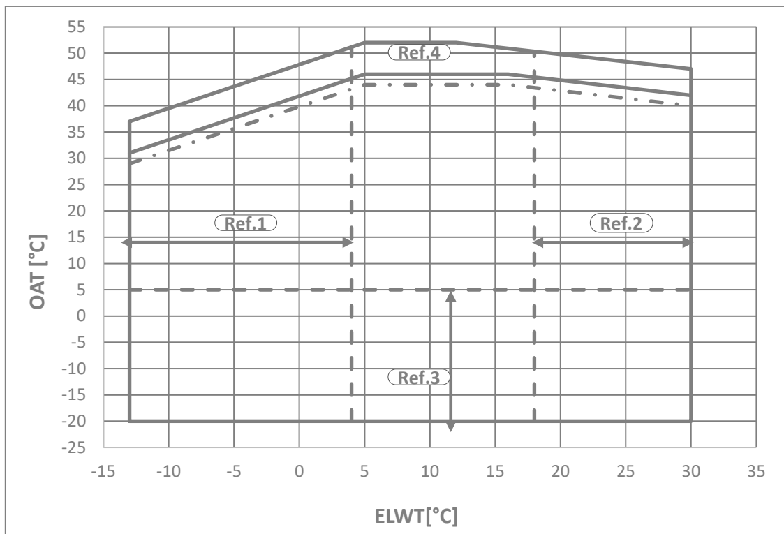
Sl. 5- Ograničenja rada za EWAT-B-C Gold
