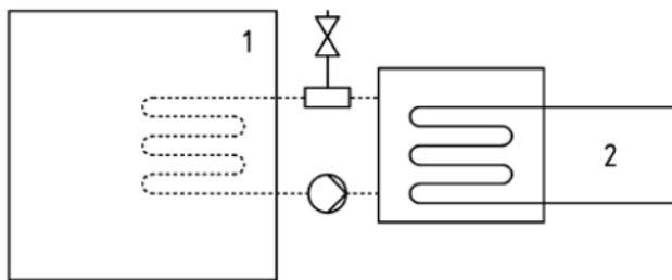
Zatvoreni sistem sa indirektnim ventilacijom
