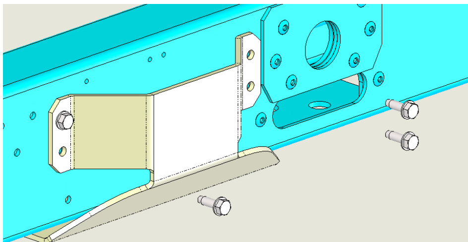
Fig. 12 - Pernos M8 para la conexión placa-marco de la unidad
