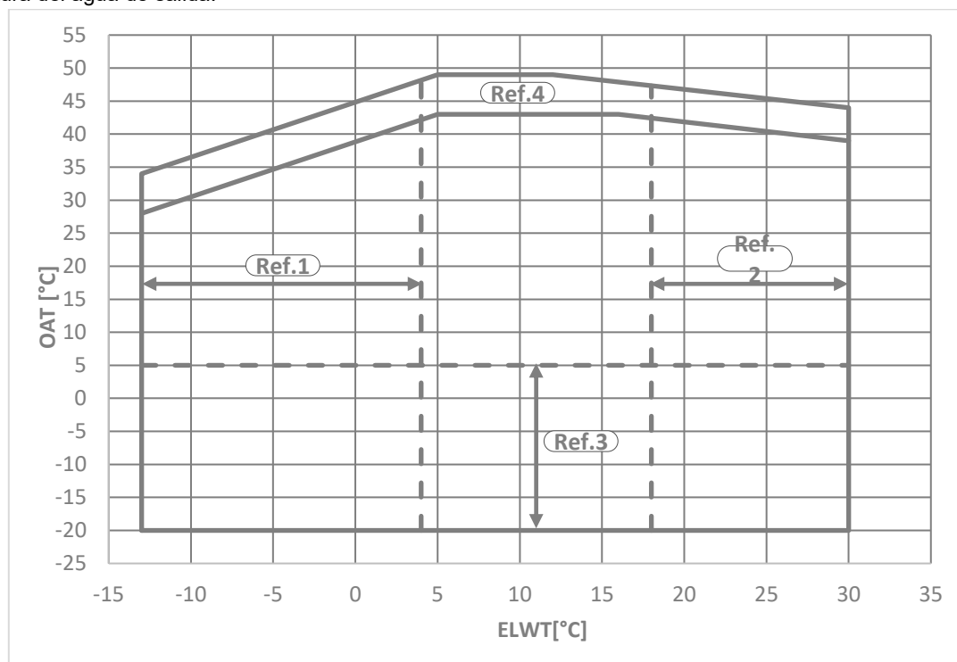
Fig. 4– EWAT-B-C Límites operativos Plata
