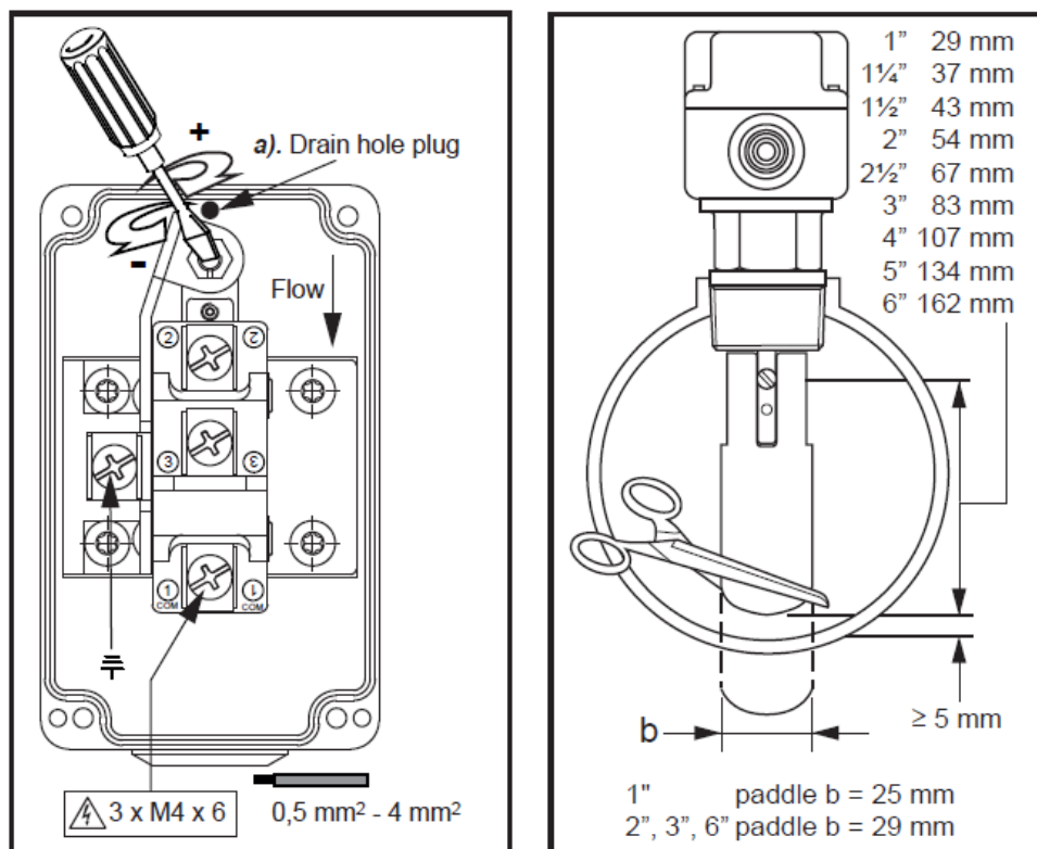
Fig. 20 – Ajuste del interruptor de flujo (modelo F61TB-9100 – Johnson Controls)
