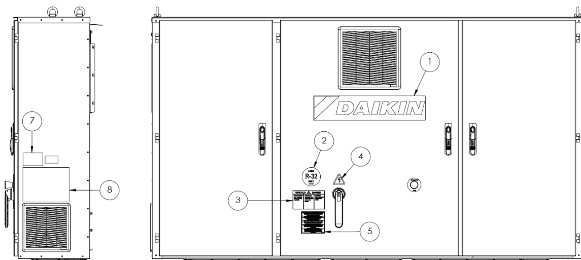
Fig. 24– Descripción de las etiquetas aplicadas al panel eléctrico medio
