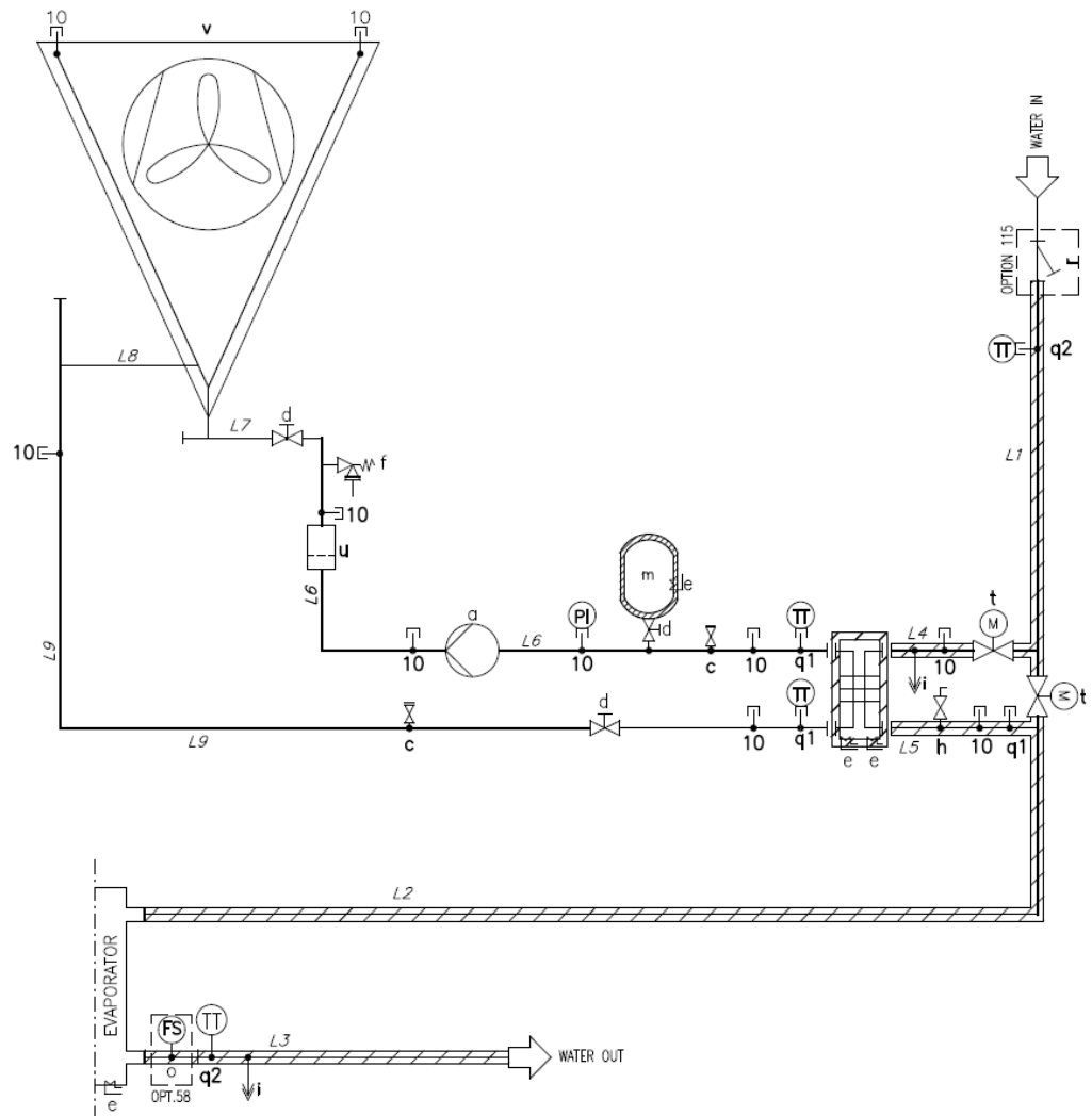
Fig. 22– Circuito cerrado Hidronico Libre de enfriamiento P&ID (Opt. 231)
