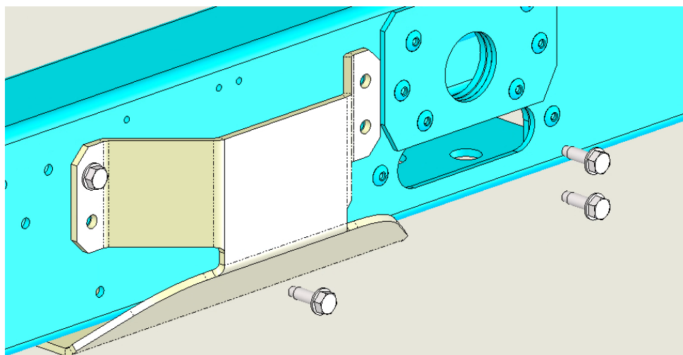
Joonis 14 – M8 poldid plaadi elemendi raami ühendamiseks
