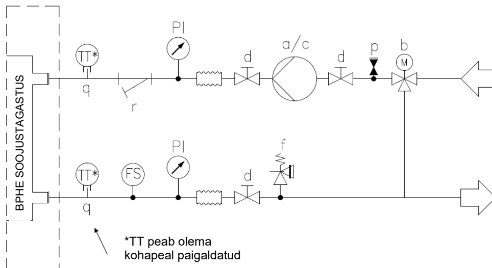
Joonis 26. Soojusvaheti veetorustiku ühendus (maksimaalne rõhk 20 bar)
