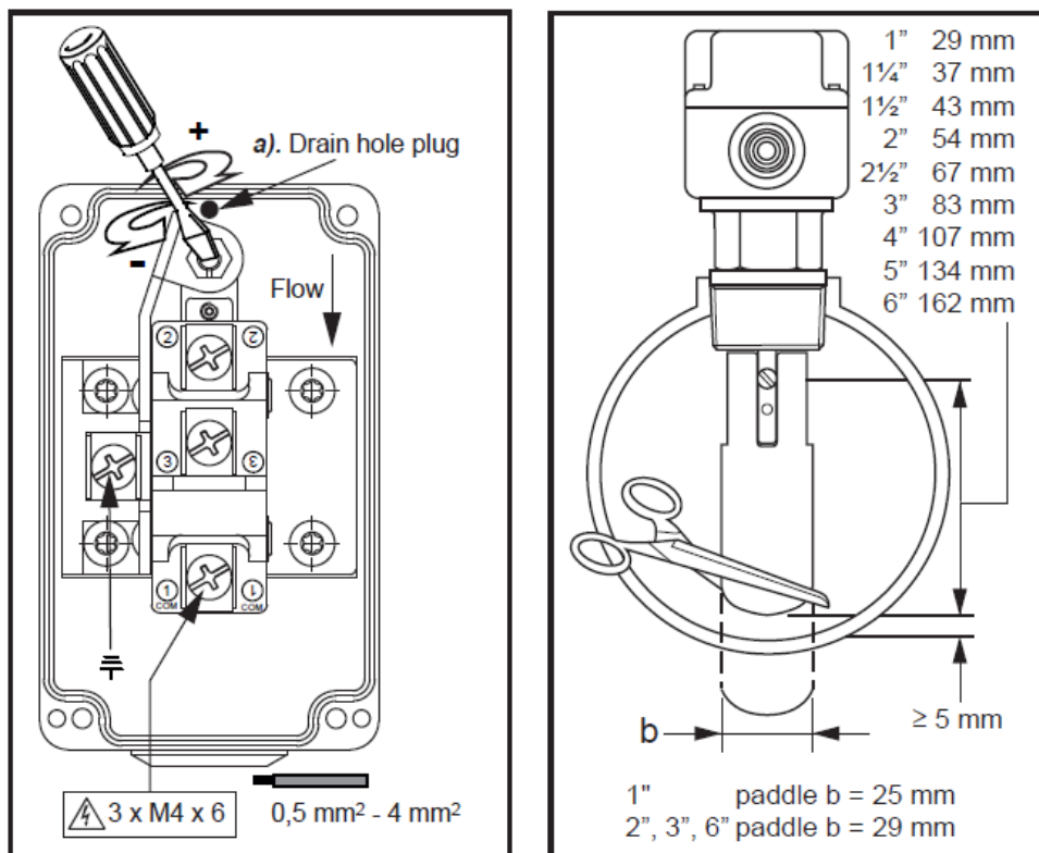
Joonis 25 – voolulüliti reguleerimine (mudel F61TB-9100 – Johnson Controls)
