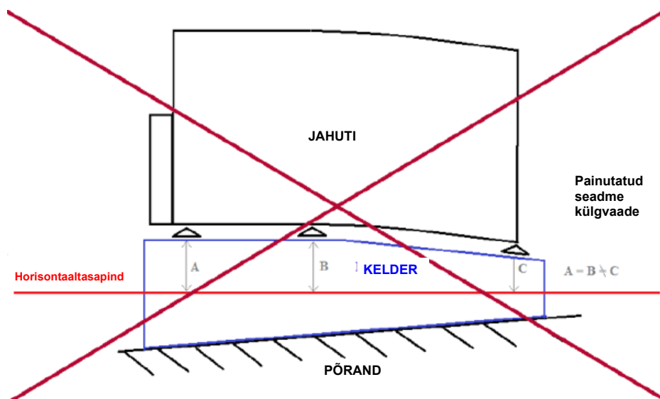
Joonis 15. Seadme loodimine
