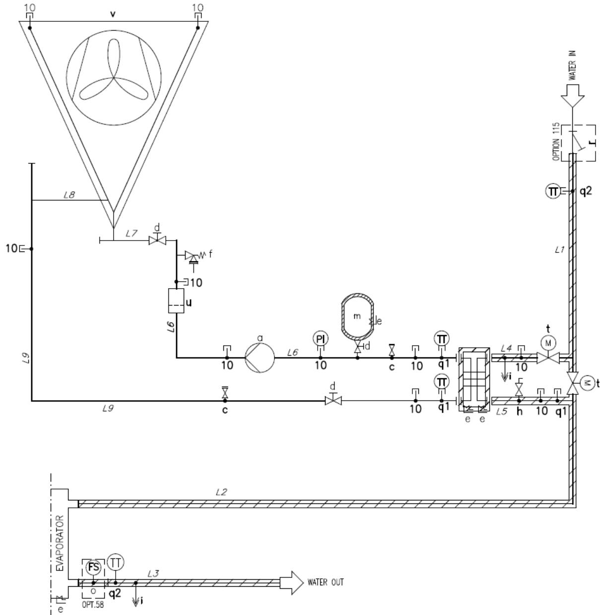
Kuva 27- Suljettu silmukka Hydroninen vapaajäähdytys P&ID (lisävaruste 231)
