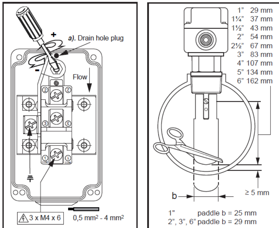
Kuva 25 – Virtauskytkimen säätö (malli F61TB-9100 – Johnson Controls)
