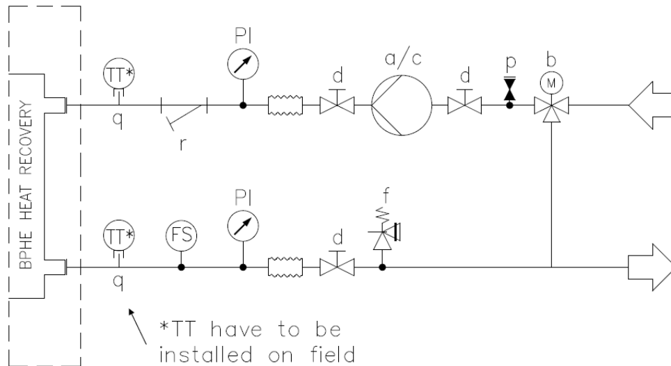
Kuva 26- Lämmöntalteenottovaihtimien vesiputkiliitäntä (enimmäispaine 20 bar)
