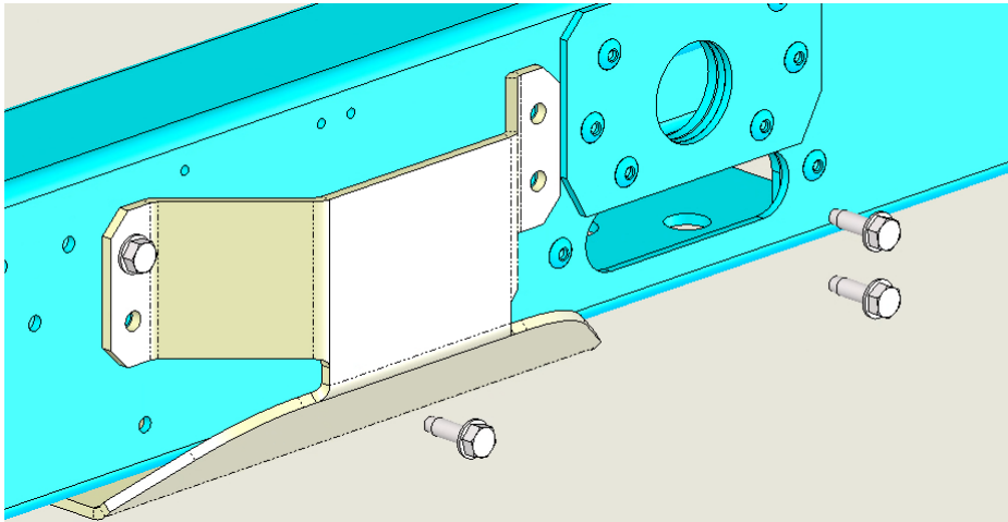
Kuva 14 – M8-pultit levyn ja yksikön rungon liittämiseen
