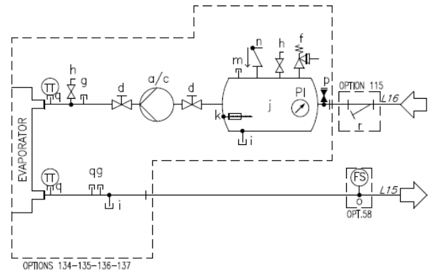
Kuva 24- Hydraulikaavio (lisävaruste 78-79-80-81/134-135-136-137)
