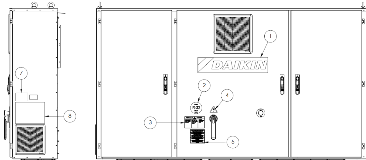
Kuva 29- Sähkötauluun kiinnitettyjen merkintöjen kuvaus keskisuuri.
