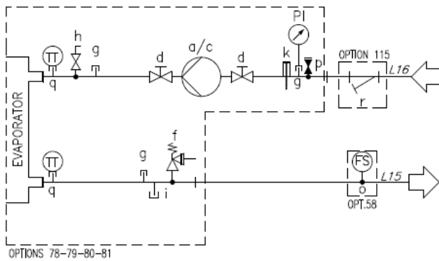
Kuva 24- Hydraulikaavio (lisävaruste 78-79-80-81/134-135-136-137)
