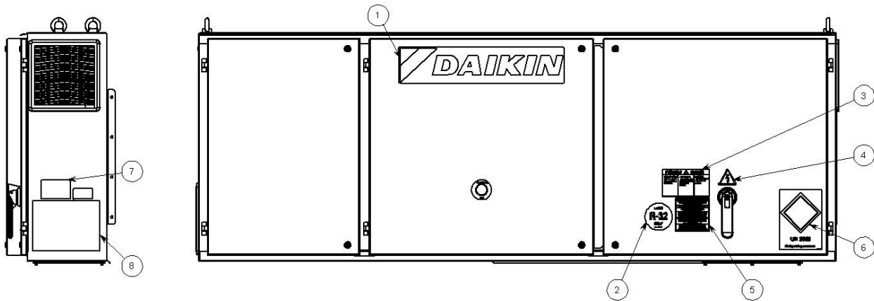
Kuva 28- Sähkötauluun kiinnitettyjen merkintöjen kuvaus pieni
