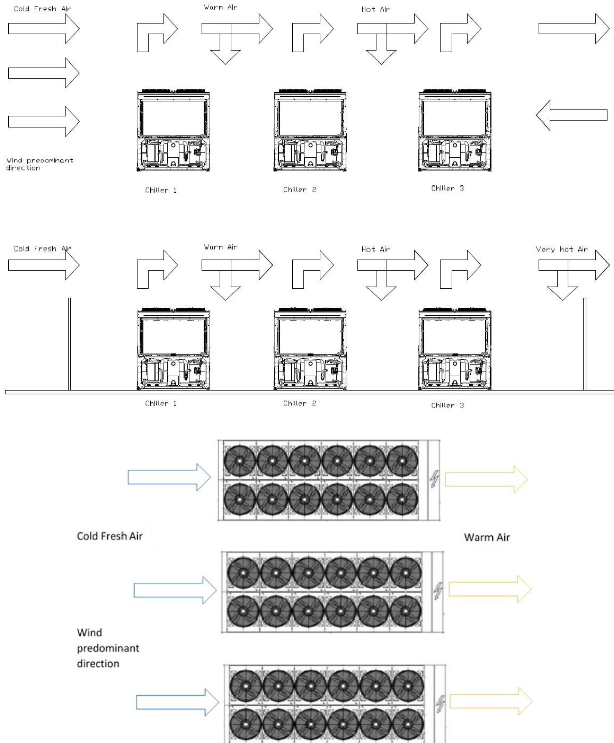
Kuva 17- Usean jäähdyttimen asennus
