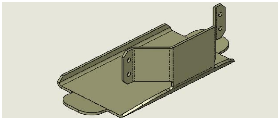
Slika 13 – Ploče OPT 71
