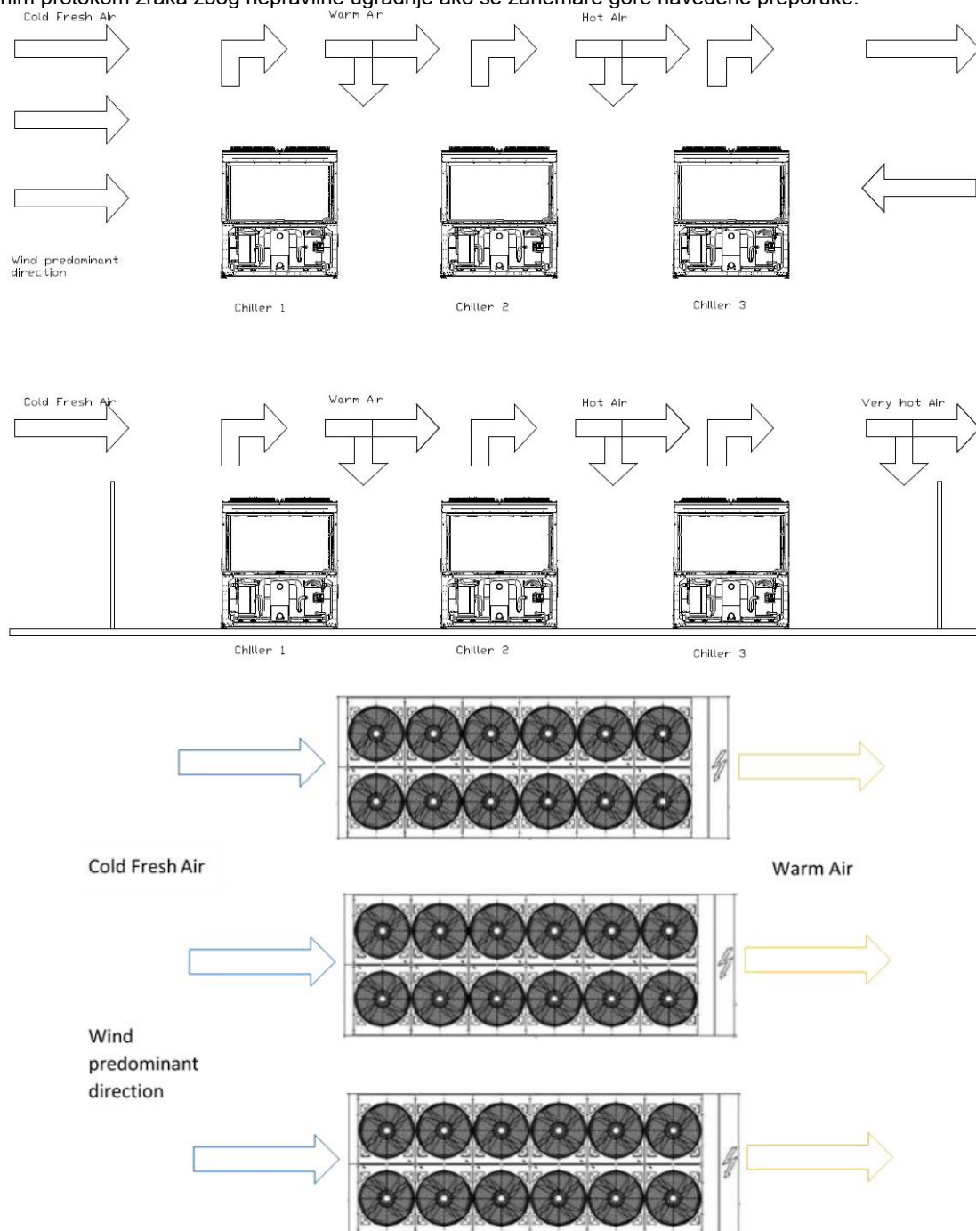
Slika 17– Instalacija više rashladnih uređaja
