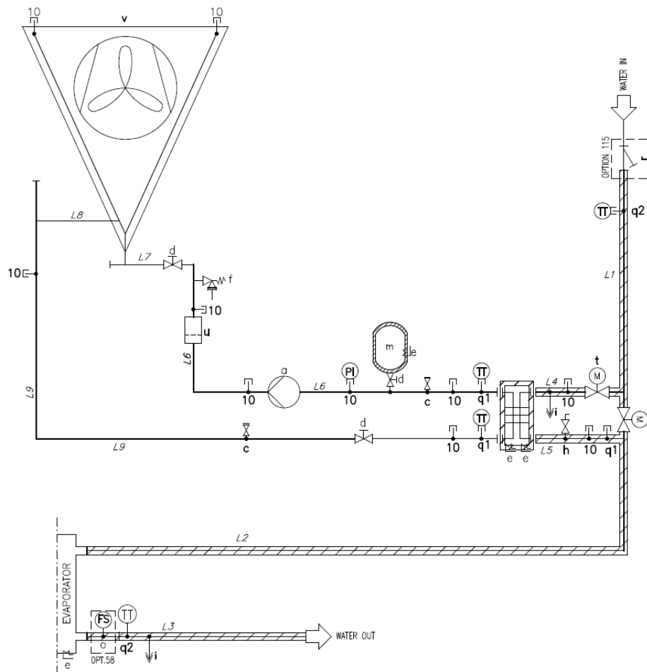
Slika 27–P&ID zatvorene petlje, hidraulično slobodno hlađenje (opcija 231)
