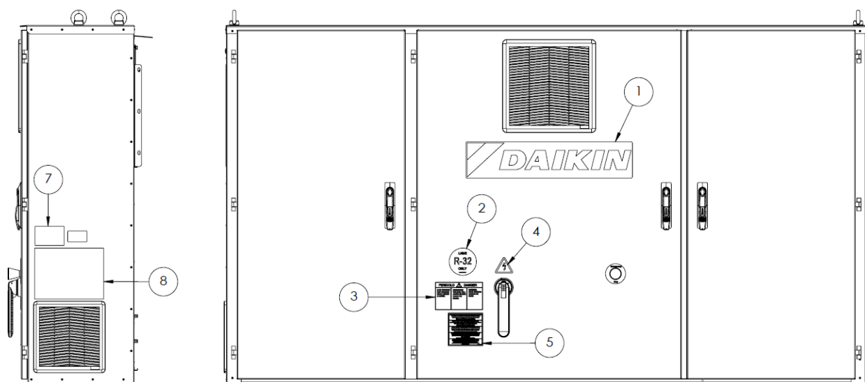
Slika 29– Opis naljepnica primijenjenih na električnu ploču (srednji).
