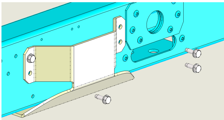
Slika 14 – Vijci M8 za povezivanje ploče i okvira jedinice
