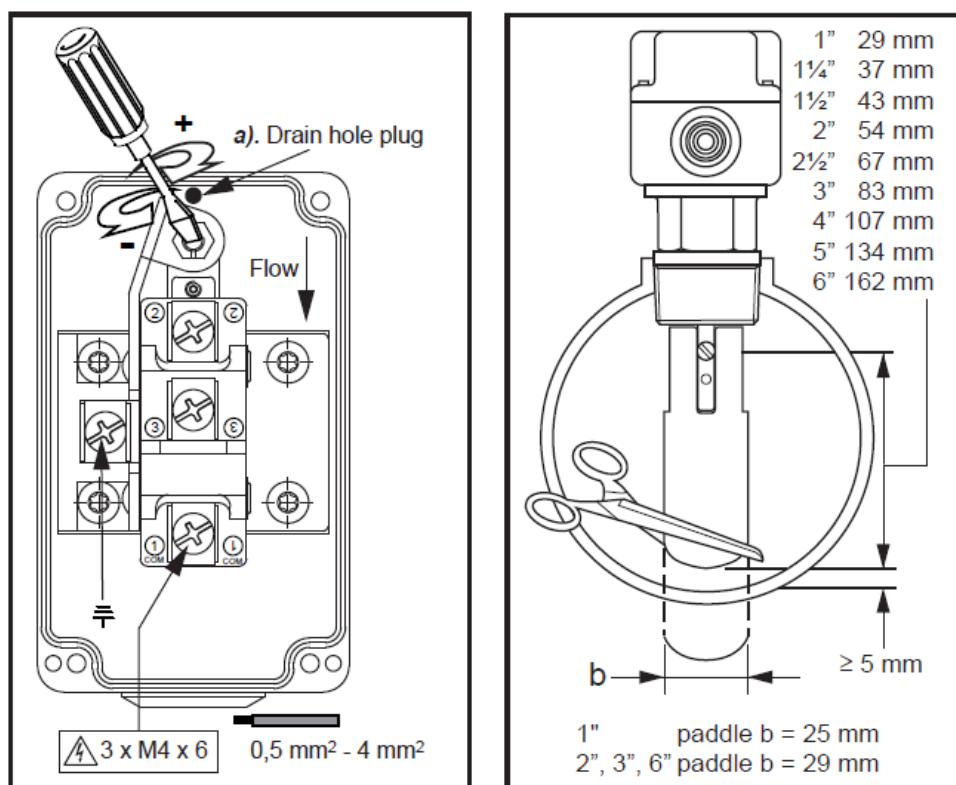
Slika 25 – Namještanje prekidača protoka (model F61TB-9100 – Johnson Controls)
