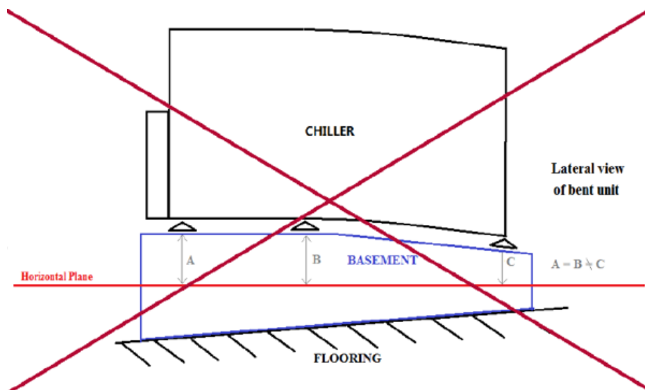
Slika 15– Niveliranje jedinice
