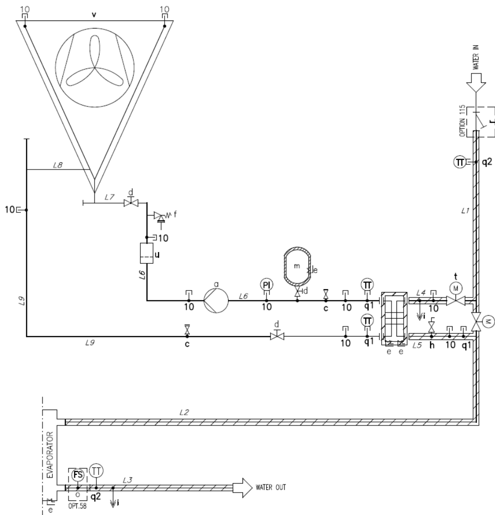
21. ábra – Zárt hurok Hydronic Ingyenes hűtés P&ID (Opt. 231)
