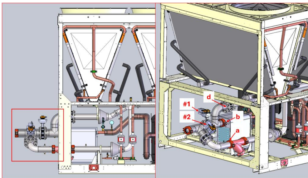
16. ábra – A csövek telepítésének részletei.
