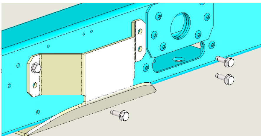
11. ábra – M8 csavarok a lemezegység keretének csatlakoztatásához
