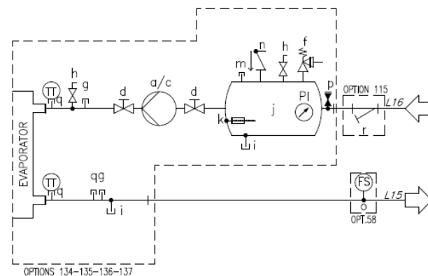
18. ábra – Hidraulikai rajz (opt. 78-79-80-81/134-135-136-137)
