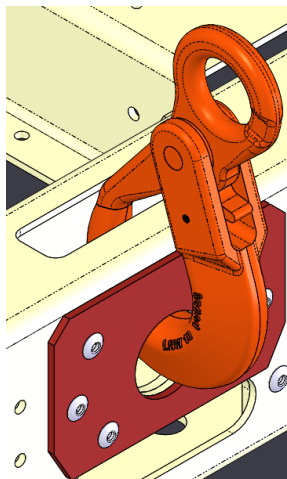
8. ábra - Biztonsági kampó rögzítése
