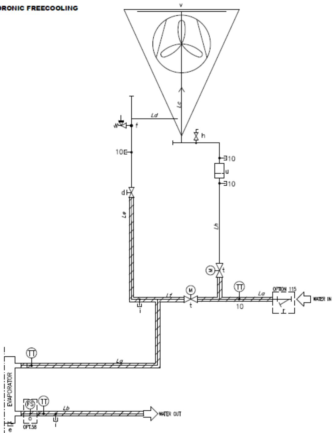
3. ábra: Vízkör diagramja (P&ID) hidronikus szabadhűtéses rendszer
