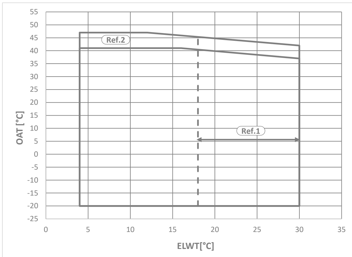
6. ábra – EWFT-B-C Silver egység üzemi tartományai
