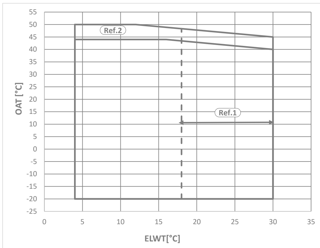
7. ábra – EWFT-B-C Gold egység üzemi tartományai
