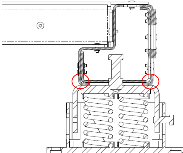
17. ábra: Rezgéscsillapító elemek felszerelése (opcionális)
