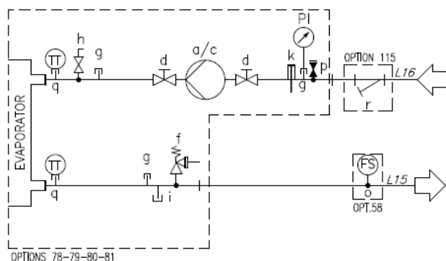
18. ábra – Hidraulikai rajz (opt. 78-79-80-81/134-135-136-137)
