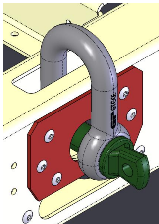
9. ábra - Emelőbilincsek rögzítése
