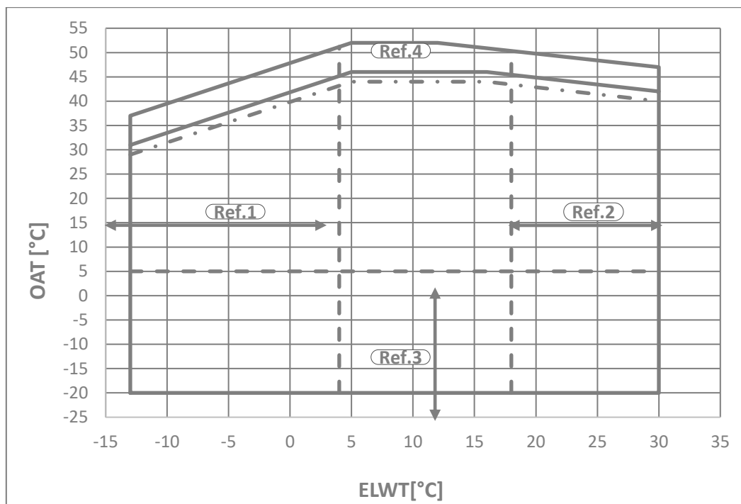
5. ábra – EWAT-B-C Gold egység üzemi tartományai
