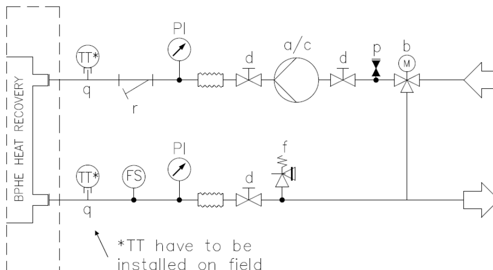
20. ábra - Vízvezeték-csatlakozás hővisszanyerős hőcserélőkhöz (maximális nyomás: 20 bar)
