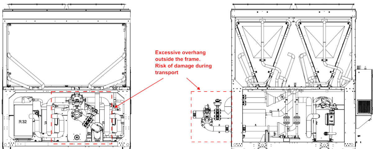
15. ábra – Csővezeték a szabadon hűtő egységek lábnyomán kívül.
