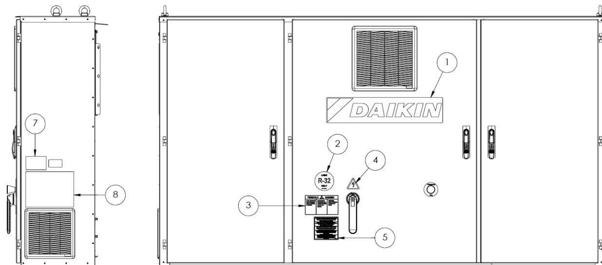
22. ábra – Az elektromos burkolatokon elhelyezett címkek értelmezése kicsi
