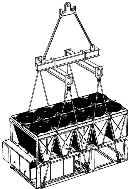
Berendezés 6 emelési ponttal
