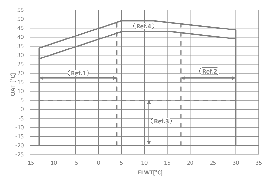
4. ábra – EWAT-B-C Silver egység üzemi tartományai
