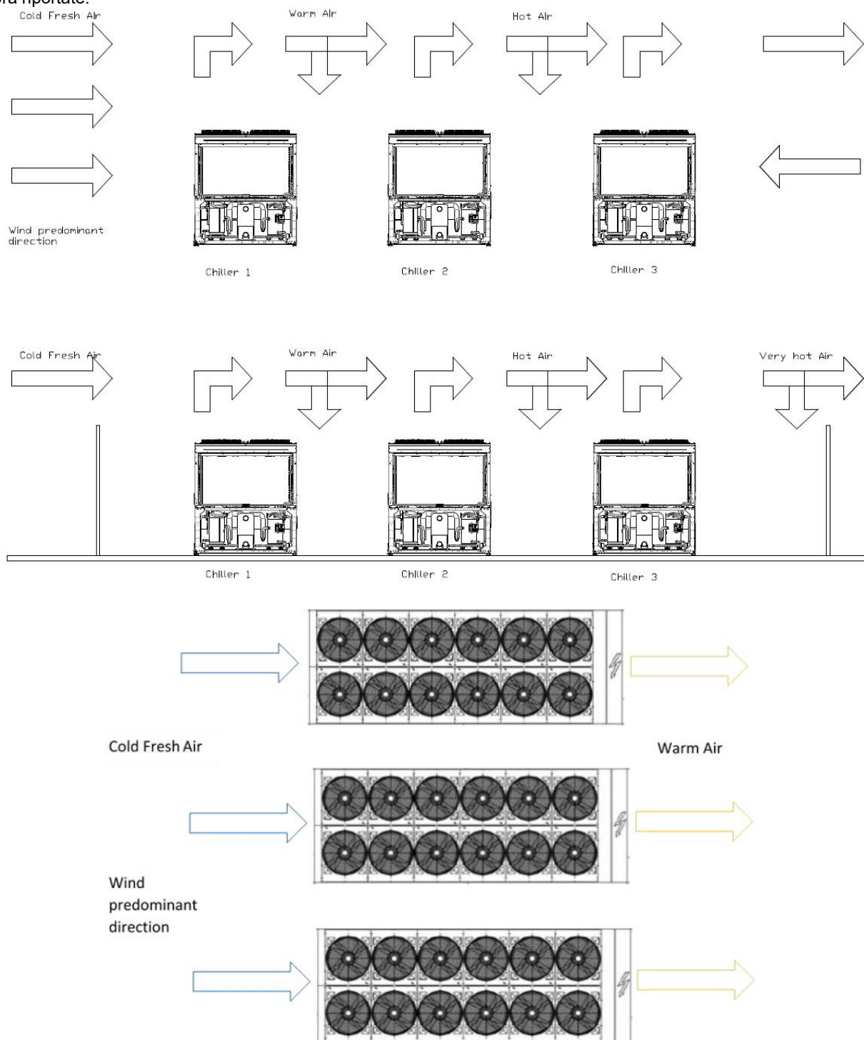
Fig. 15– Installazione di chiller multipli
