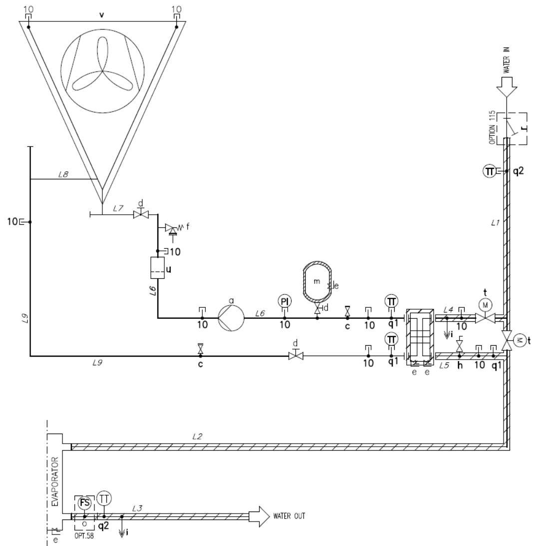
Fig. 22– P&ID del Free cooling idronico a ciclo chiuso (Opt. 231)
