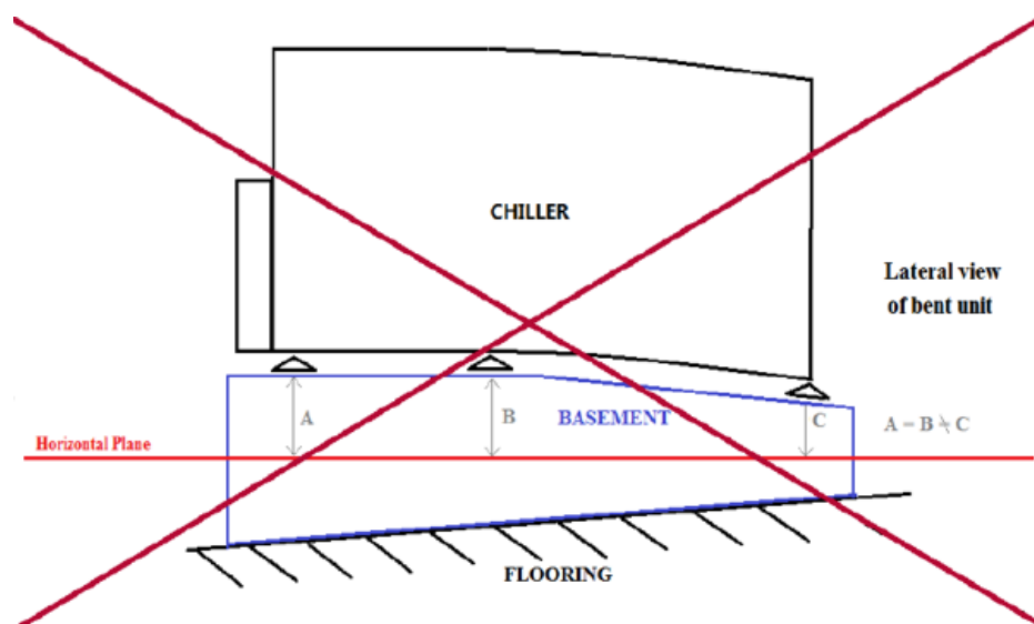
Fig. 13– Livellamento unità
