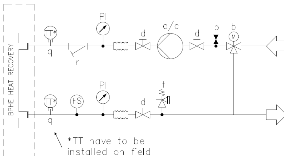
Fig. 21- Collegamento circuito dell'acqua per scambiatori con recupero di calore (pressione massima 20bar)
