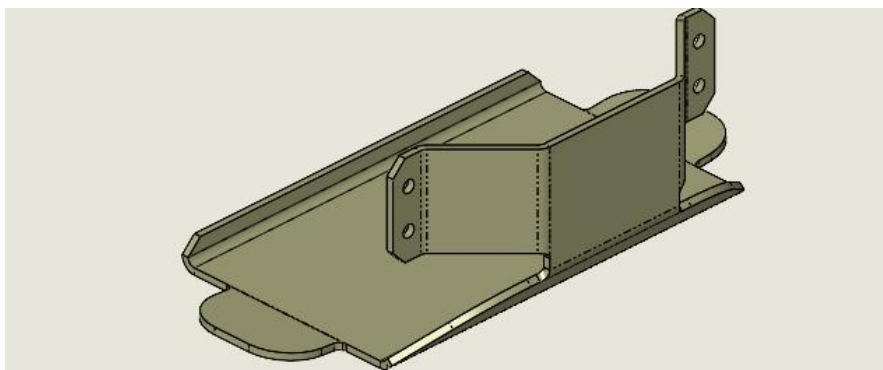
Fig. 11 - Lamiera OPT 71
