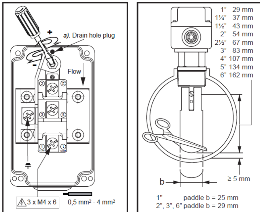
Fig. 20– Regolazione del flussostato (modello F61TB-9100 – Johnson Controls)
