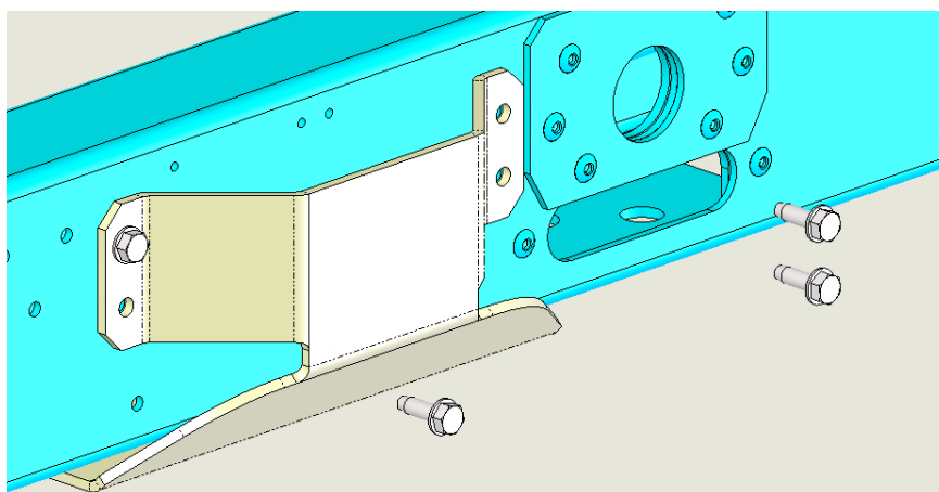
Fig. 12 - Viti M8 per accoppiamento lamiera-telaio
