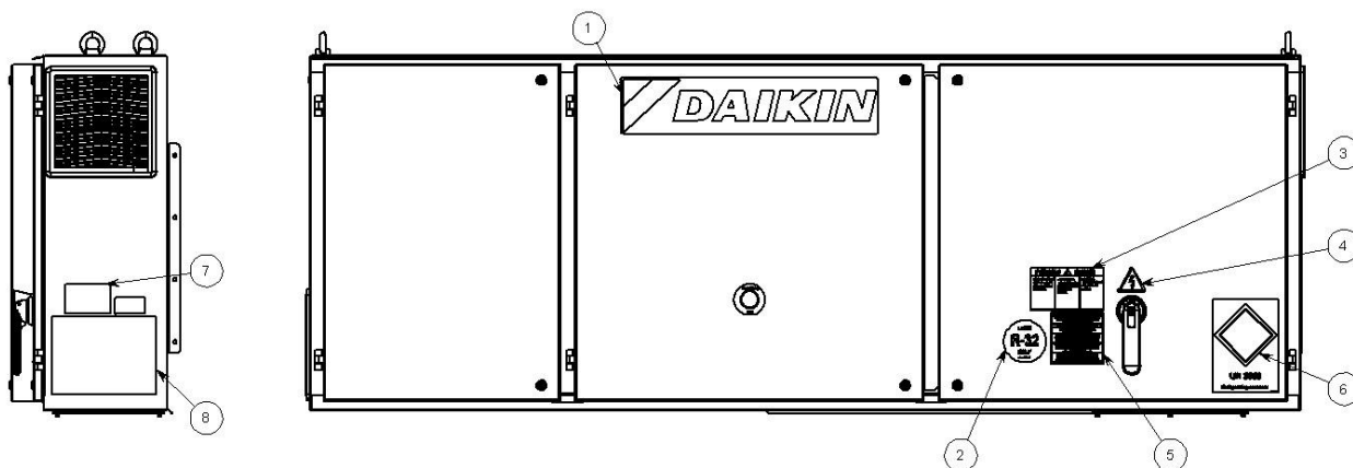
Fig. 23– Descrizione etichette applicate su quadro elettrico(piccolo)
