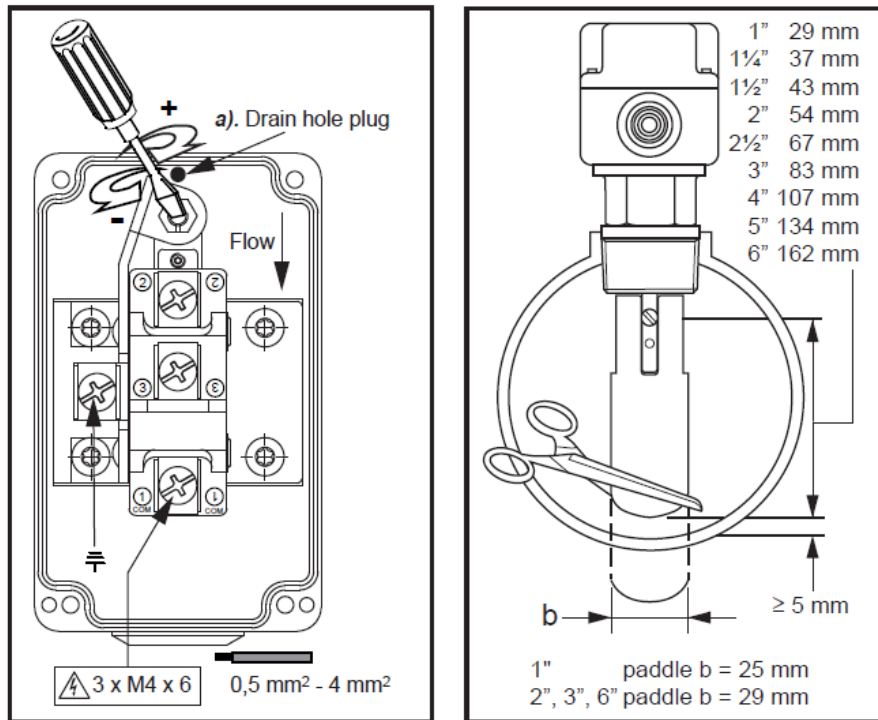
Afb. 20– Afstelling stromingsschakelaar (model F61TB-9100 – Johnson Controls)
