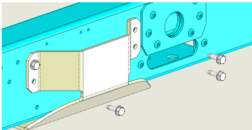
Afb. 12 - M8 bouten voor plaat-unit frame verbinding
