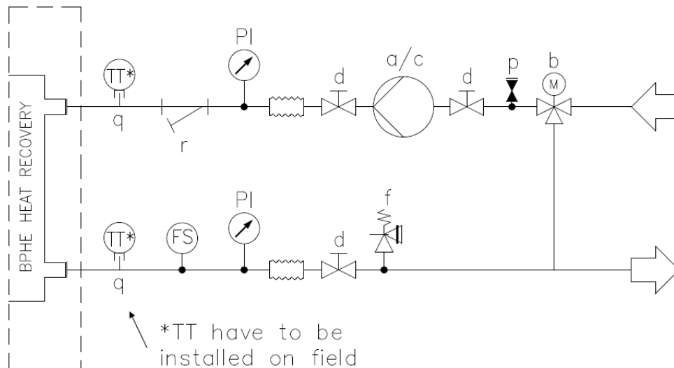
Afb. 21- Aansluiting waterleiding voor warmteterugwinningswisselaars (maximum druk 20 bar)
