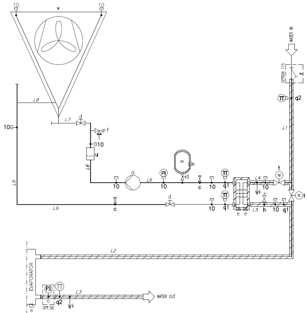
Afb. 22– Gesloten lus Hydronic Gratis koeling P&ID (Opt. 231)
