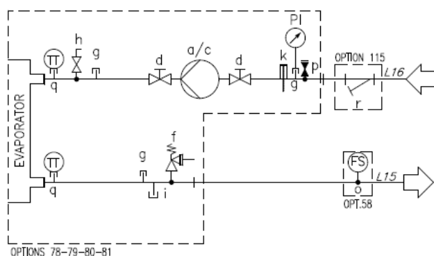
Rys. 19– Schemat hydrauliczny (opt. 78-79-80-81/134-135-136-137)
