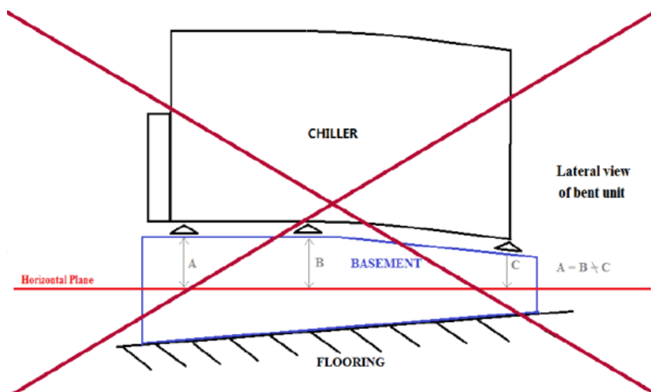
Rys. 13– Poziomowanie jednostki
