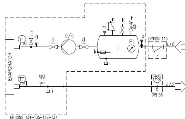
Rys. 19– Schemat hydrauliczny (opt. 78-79-80-81/134-135-136-137)
