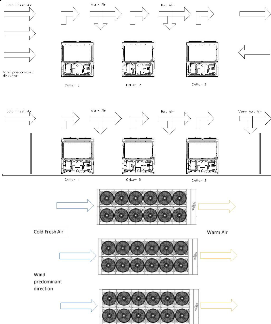
Rys. 15– Montaż kilku wytwornic wody lodowej
