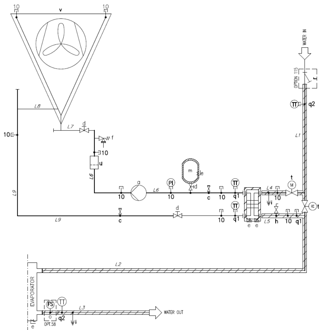
Rys. 22– Zamknięta pętla Hydronic Bezpłatne chłodzenie P&ID (op. 231)
