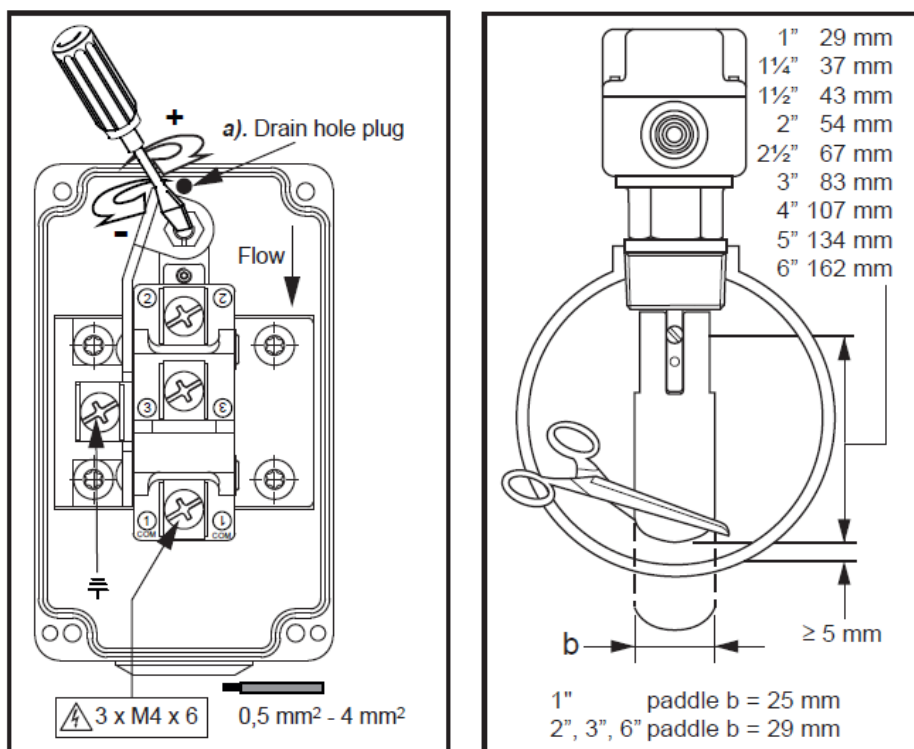
Rys. 20– Regulacja przepływomierza (model F61TB-9100 – Johnson Controls)
