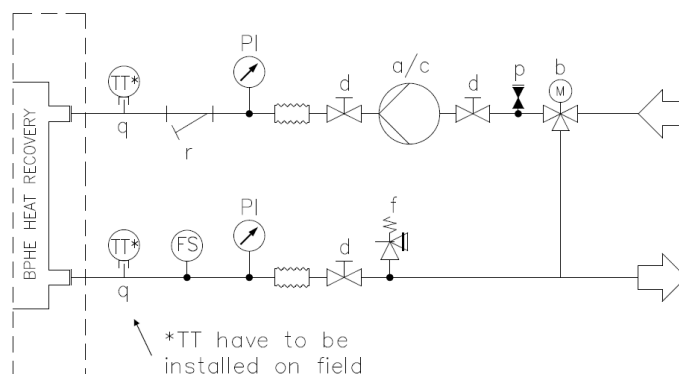
Rys. 21- Podłączenie przewodów wodnych do wymienników z odzyskiem ciepła (maksymalne ciśnienie 20 bar)
