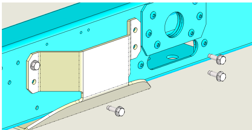
Rys. 12 – Śruby M8 do połączenia płyta-rama urządzenia
