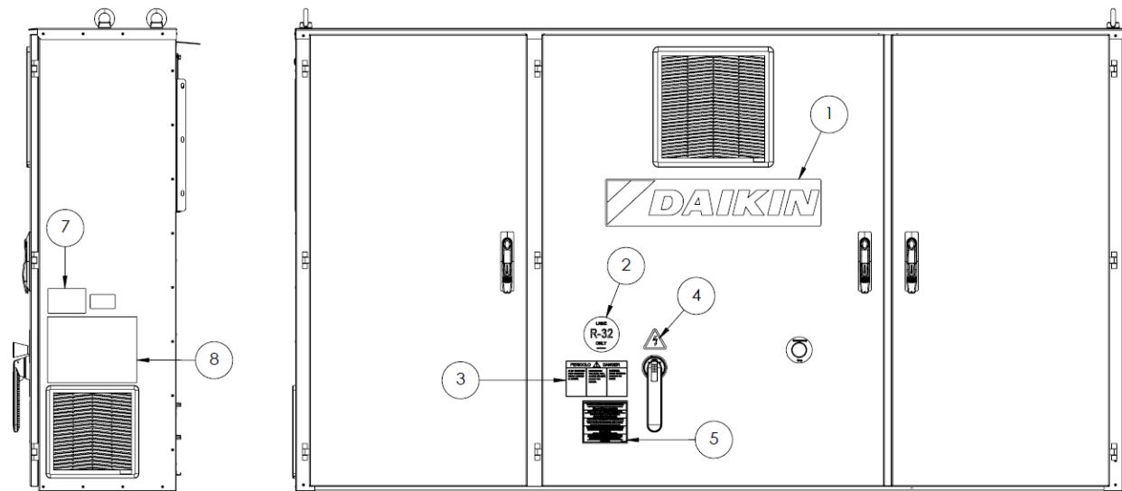
Rys. 23– Opis tabliczek umieszczonych na panelu elektrycznym małym.
