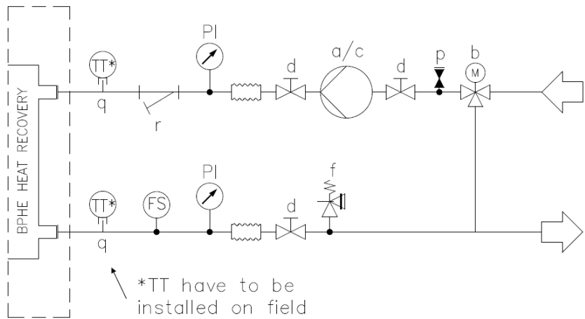
Fig. 21- Esquema hidráulico sem bomba(s) a bordo (pressão máxima de 20 bar)
