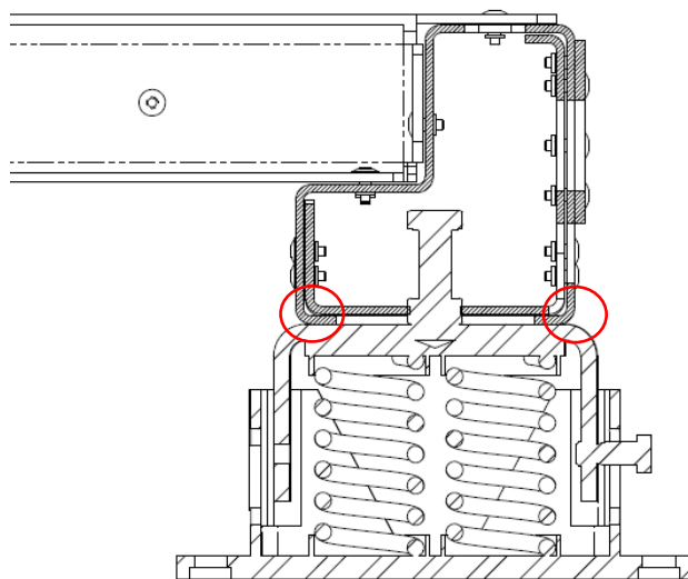
Fig. 18 - Montagem de elementos anti-vibração (fornecidos como opção)
