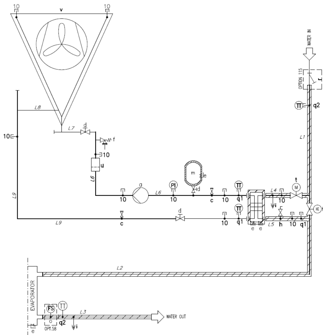
Fig. 22– Circuito fechado Hydronic Free cooling P&ID (Opt. 231)
