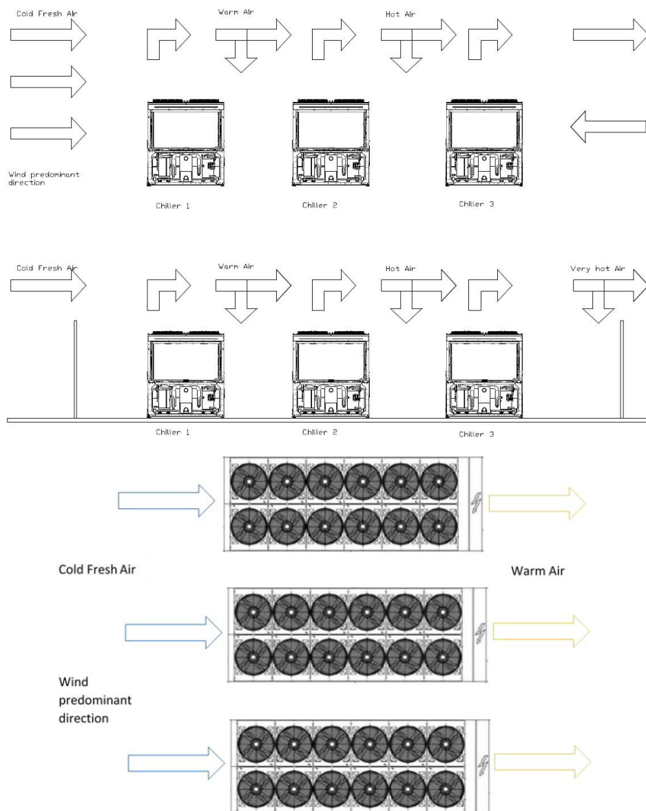
Fig. 15– Instalação de múltiplos refrigeradores
