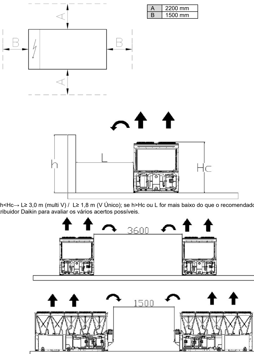
Fig. 14– Requisitos mínimos de espaço
