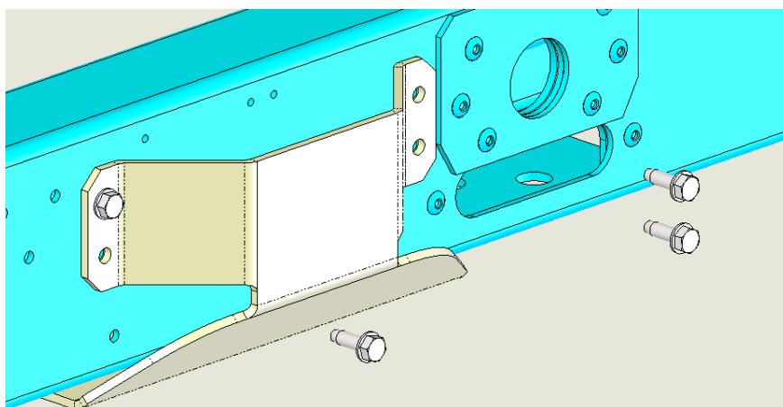
Fig. 12 – Parafusos M8 para ligação placa-estrutura da unidade
