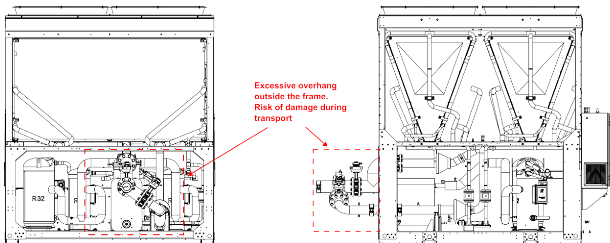
Fig. 16– Tubulação fora da pegada de unidades de refrigeração livre.
