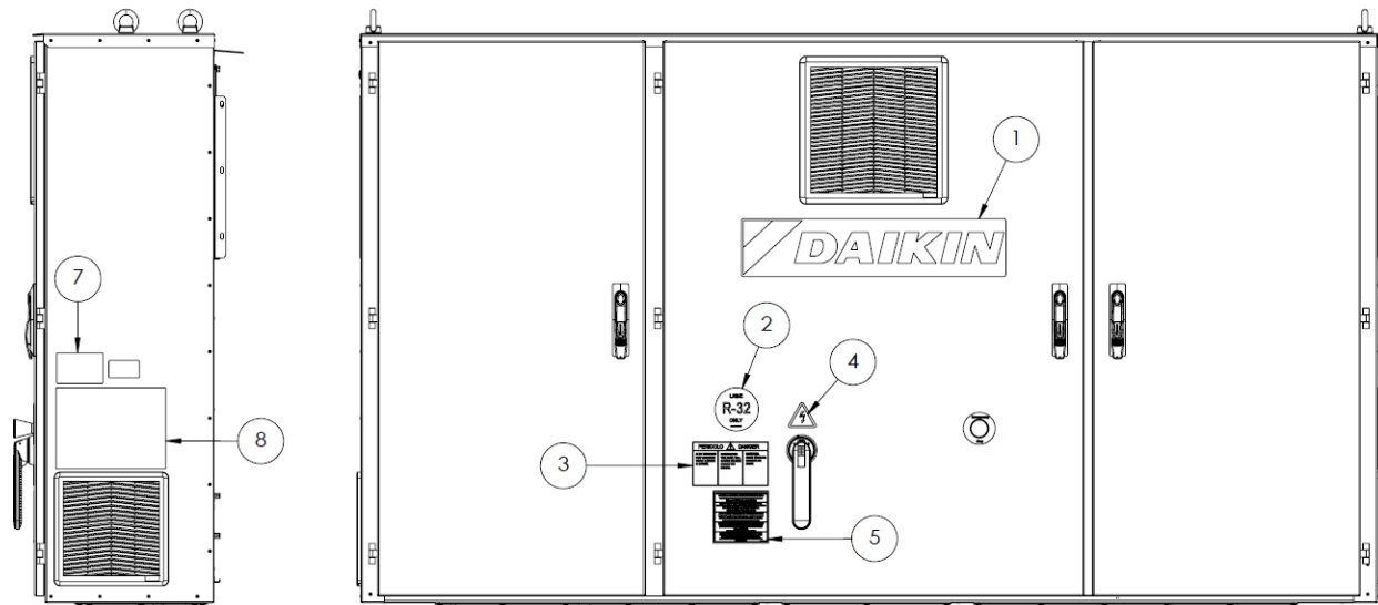
Fig. 23– Descrição das etiquetas aplicadas no painel elétrico (pequeno)
