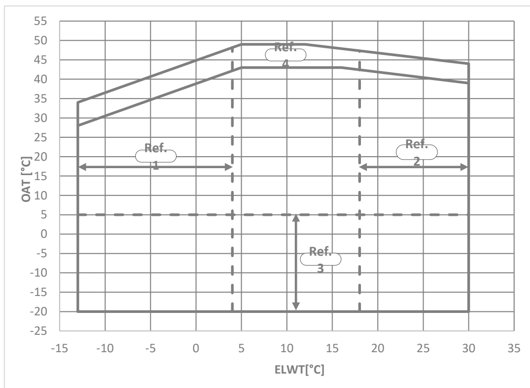
Fig. 4– EWAT-B-C Limites de funcionamento Silver
