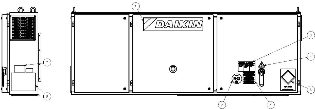
Fig. 23– Descrição das etiquetas aplicadas no painel elétrico (pequeno)
