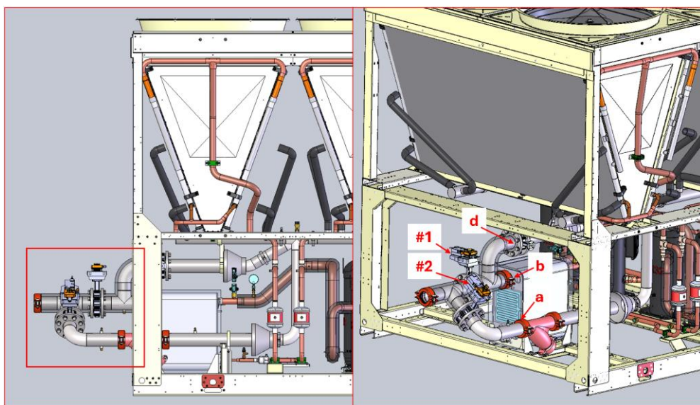
Fig. 17– Detalhes da instalação de tubulação.
