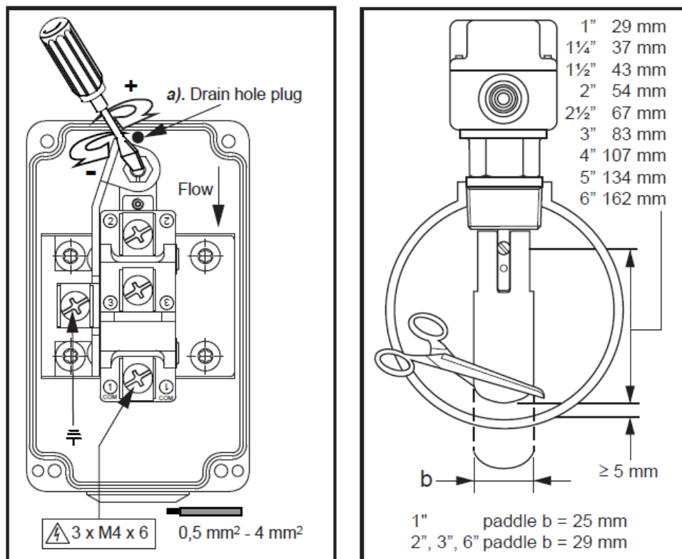
Fig. 20– Ajuste do interruptor de fluxo (modelo F61TB-9100 – Johnson Controls)
