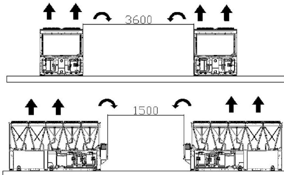
Fig. 14– Cerințe minime de spațiu
