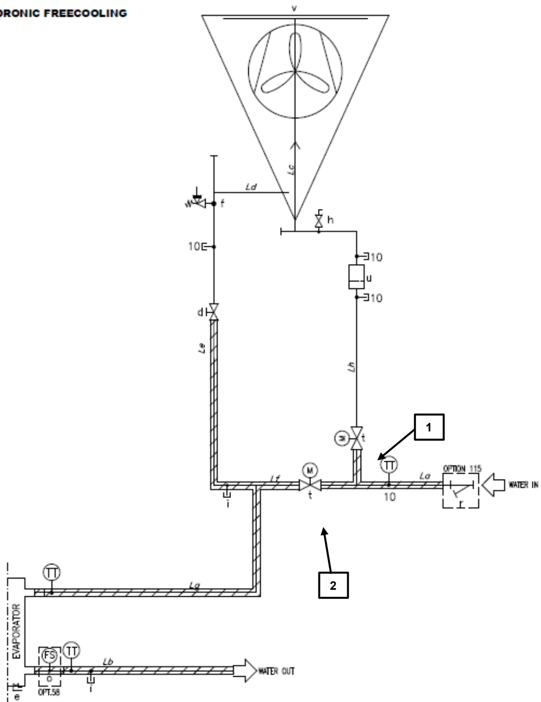
Fig. 3 – Sistem hidronic de răcire liberă (P&ID)
