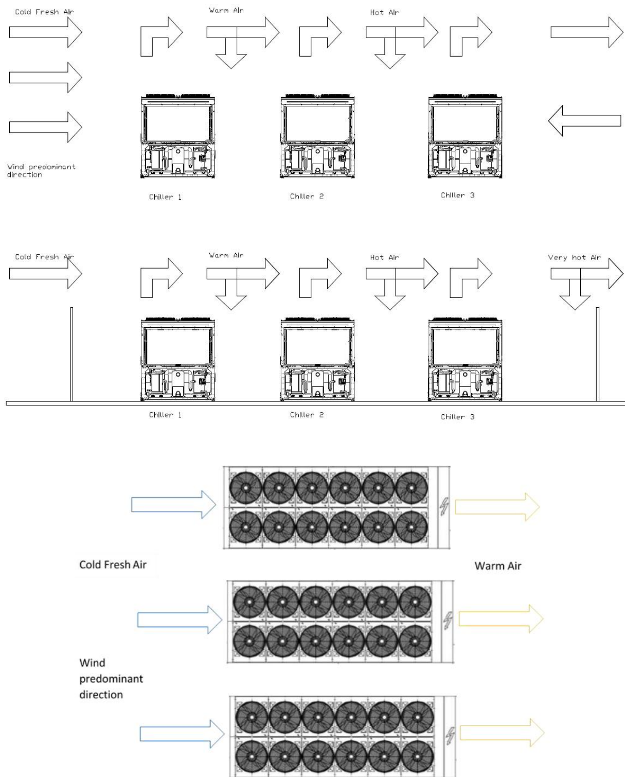
Fig. 15– Instalarea mai multor răcitoare
