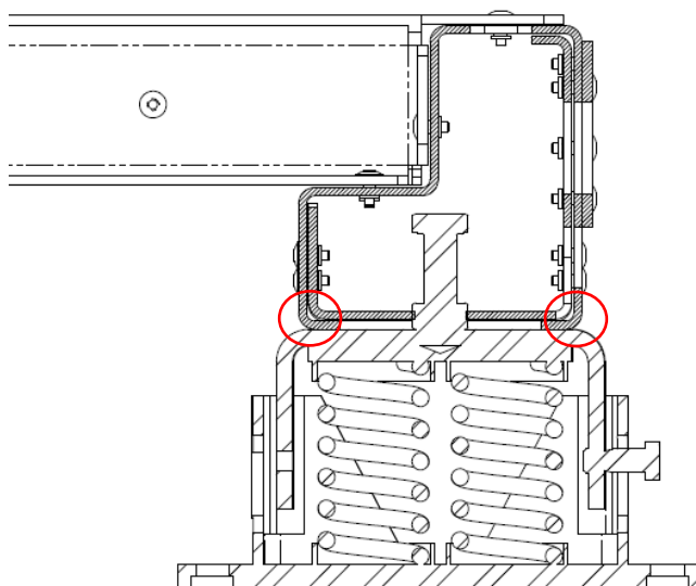
Fig. 18 - Montarea elementelor antivibrații (furnizate opțional)
