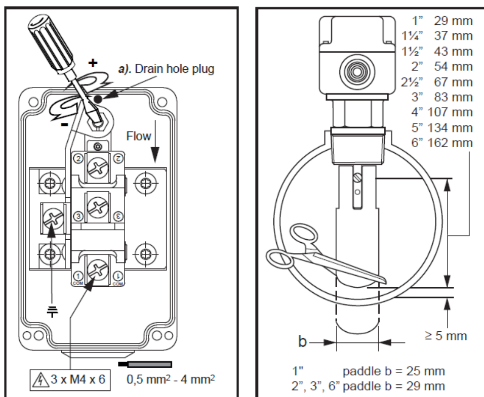
Fig. 20– Reglarea întrerupătorului de debit (model F61TB-9100 – Johnson Controls)
