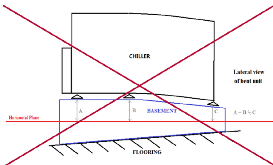
Fig. 13– Aducerea la nivel a unității
