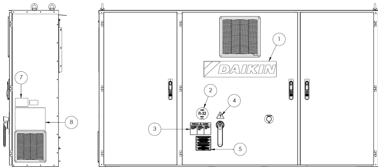
Fig. 24- Descrierea etichetelor aplicate pe panoul electric mediu.
