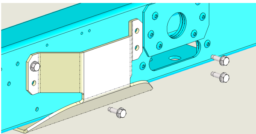
Fig. 12 – Șuruburi M8 pentru conectarea cadrului unității la placă
