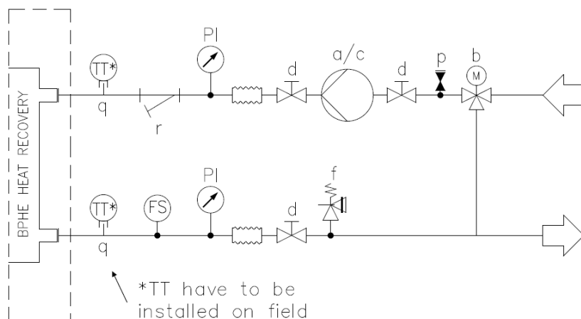
Fig. 21- Conectarea conductelor de apă pentru schimbătoarele de căldură (presiune maximă 20 bari)
