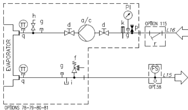
Fig. 19– Diagrama hidraulică (opt. 78-79-80-81/134-135-136-137)
