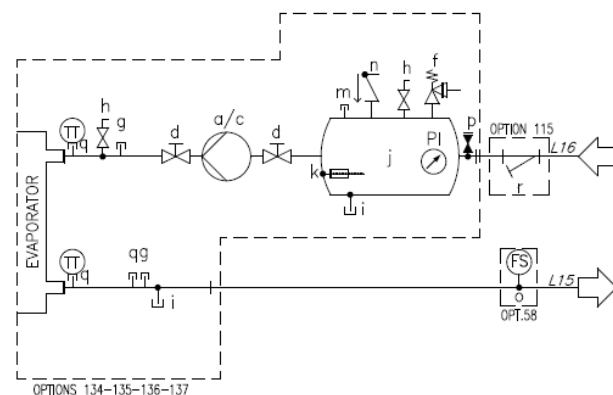
Fig. 19– Diagrama hidraulică (opt. 78-79-80-81/134-135-136-137)
