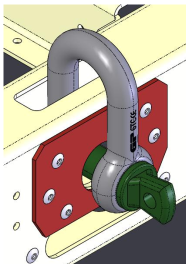
Fig. 10 - Fixarea cătușelor de ridicare
