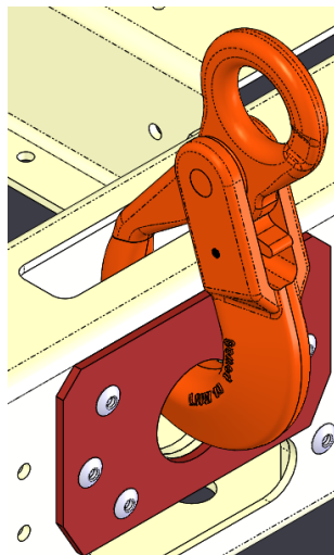
Fig. 9- Fixarea cârligului de siguranță
