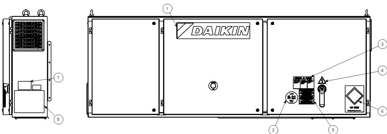
Obr. 28– Popis štítkov umiestnených na elektrickom paneli (malé)
