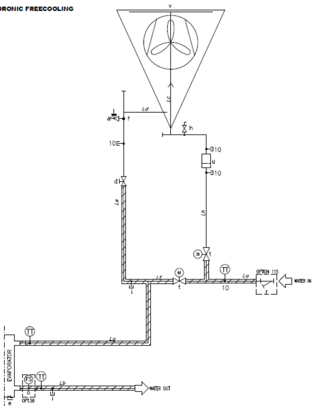
Obr. 3 – Hydraulický systém s voľným chladením (P&ID)
