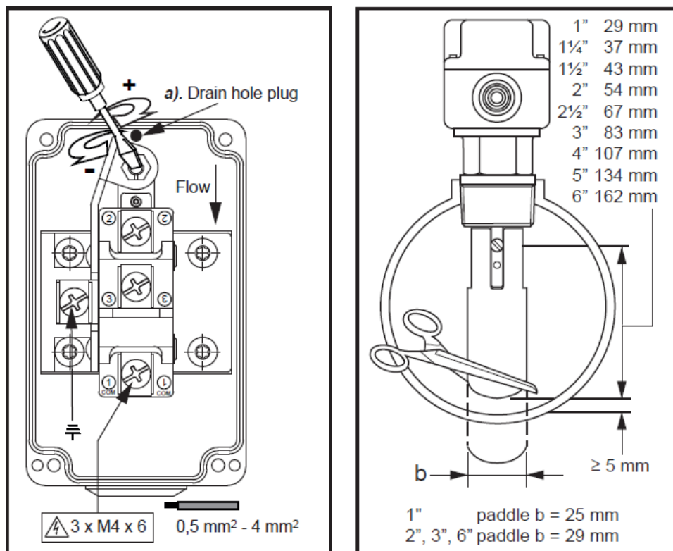
Obr. 25 - Nastavenie prietokového spínača (model F61TB-9100 – Johnson Controls)
