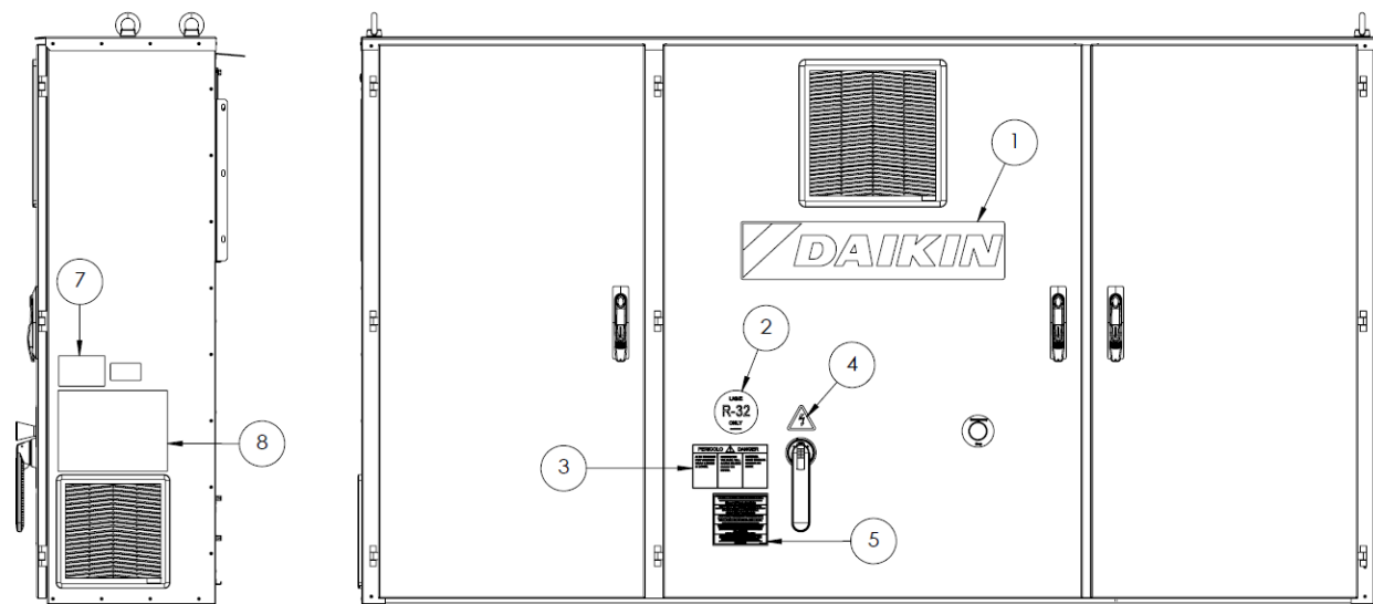
Obr. 29– Popis štítkov umiestnených na elektrickom paneli (stredne)
