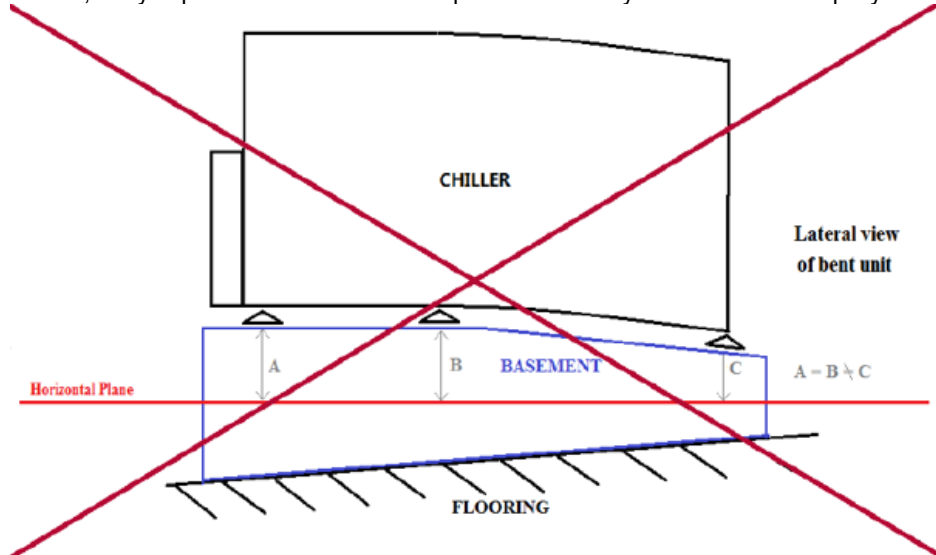
Obr. 15 – Vyrovnanie jednotky
