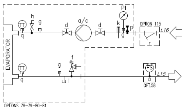
Obr. 24– Hydraulická schéma (vol. 78-79-80-81/134-135-136-137)
