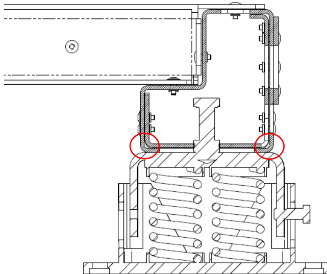
Obr. 20 - Montáž antivibračných prvkov (dodávajú sa ako voliteľné príslušenstvo)
