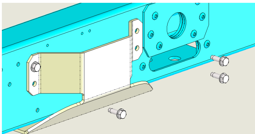
Obr. 14 – M8 skrutky pre pripojenie platne k rámu jednotky
