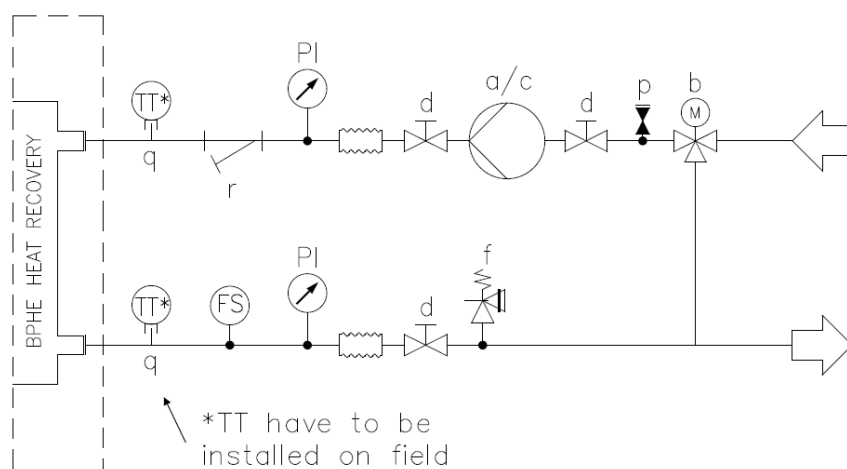
Obr. 26- Pripojenie vodovodného potrubia pre rekuperačné výmenníky (maximálny tlak 20 bar)
