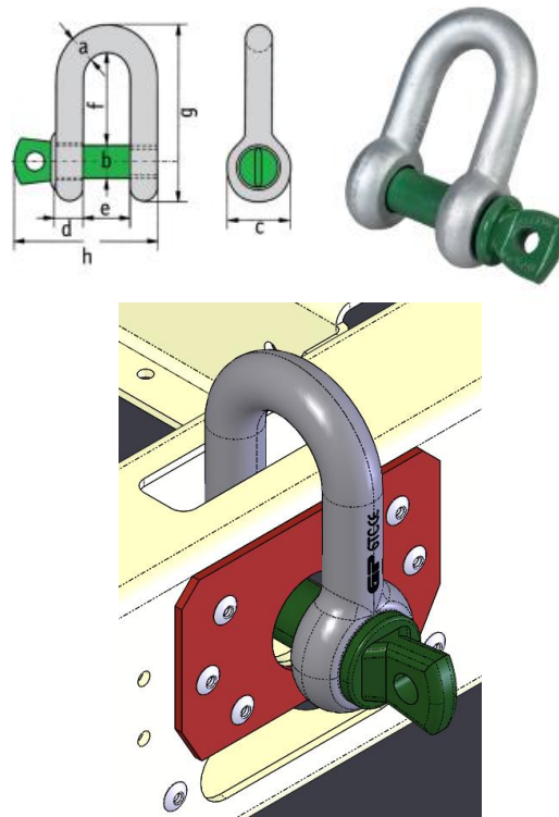
Fig. 20 Fijación de los grilletes de elevación
