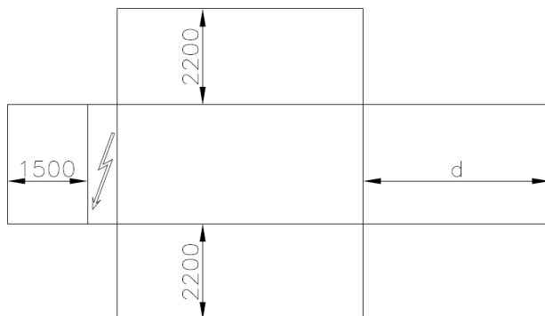
Fig. 25 - Requisitos de espacio mínimo
