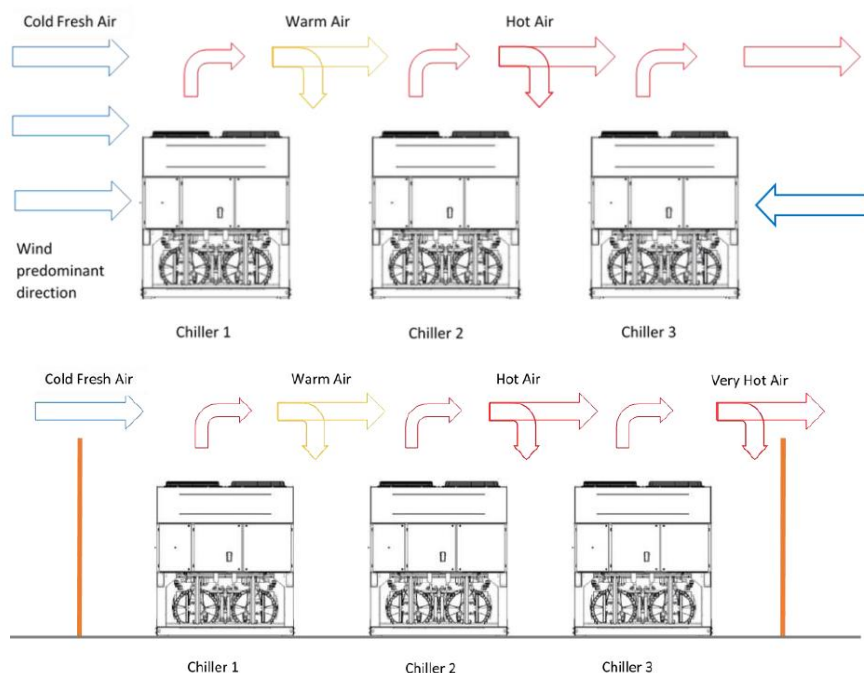
Fig. 26 – Instalación de Múltiples Refrigeradores
