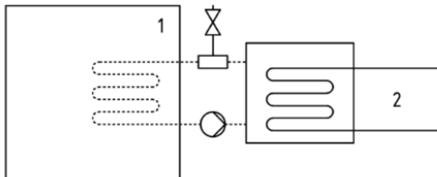
17. ábra - Közvetett szellőzésű zárt rendszer
