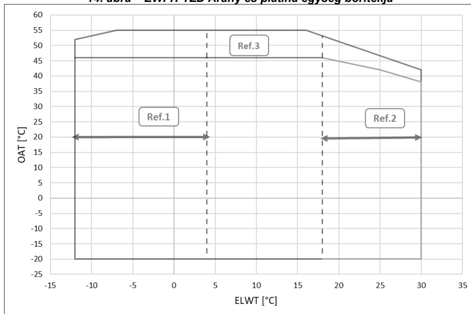
14. ábra – EWFD-TZD Arany és platina egység borítékja
