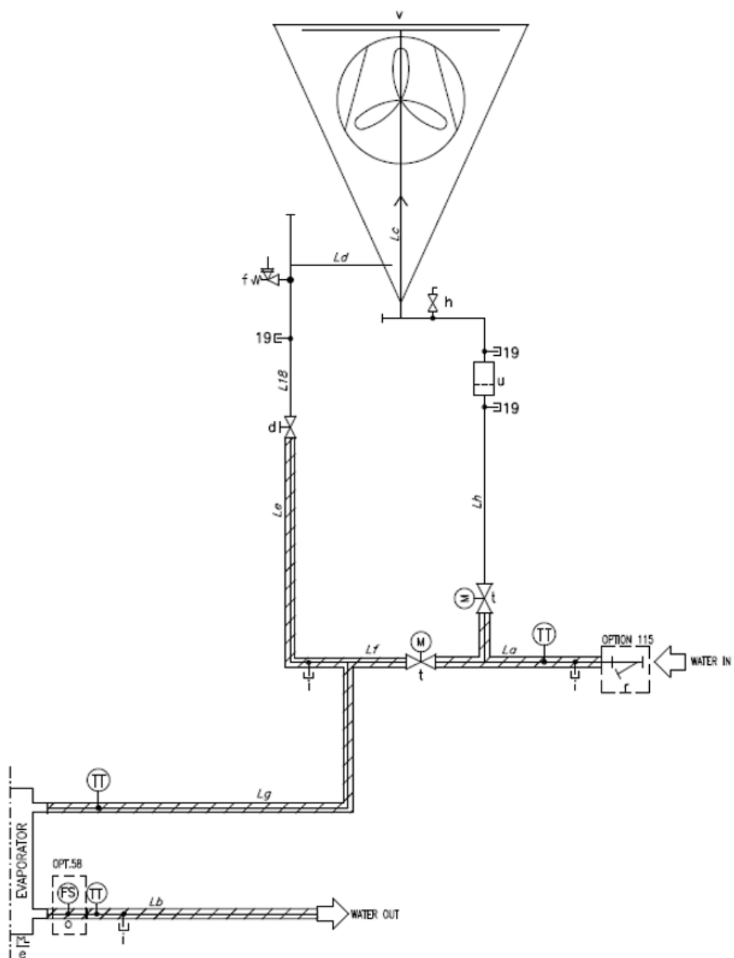
Figura 28– Schemă P&ID răcire hidronică liberă
