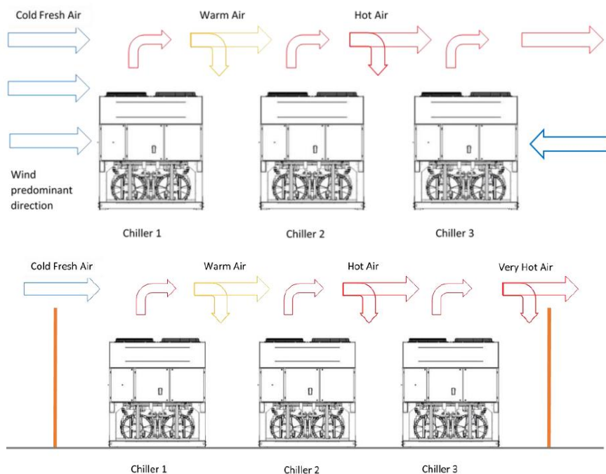
Εικ. 26 – Εγκατάσταση πολλών ψυκτών
