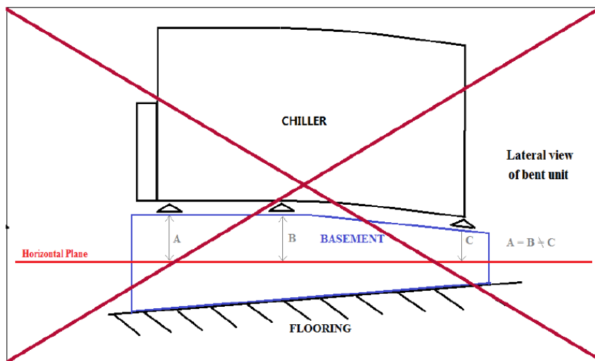
Εικ. 21 – Οριζοντίωση μονάδας
