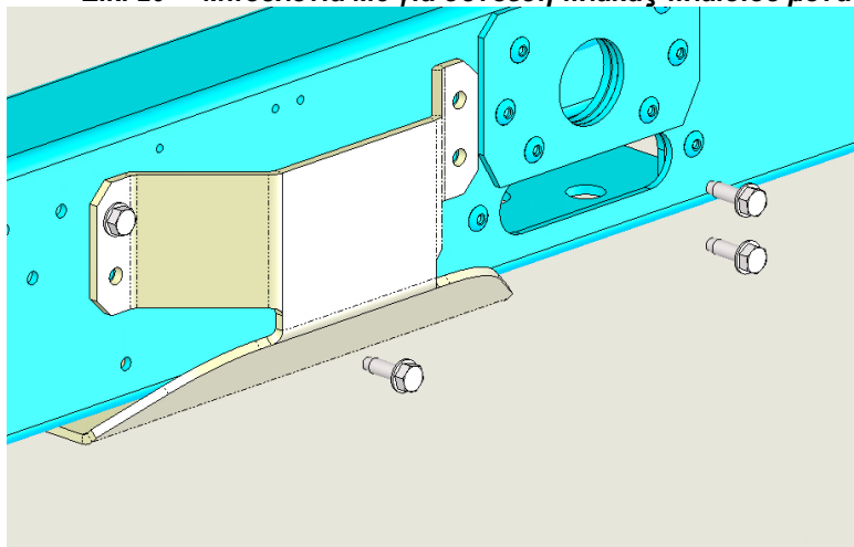
Εικ. 20 – Μπουλόνια M8 για σύνδεση πλάκας-πλαισίου μονάδας
