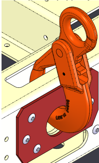
Εικ. 23 - Προσάρτηση γάντζου ασφαλείας
