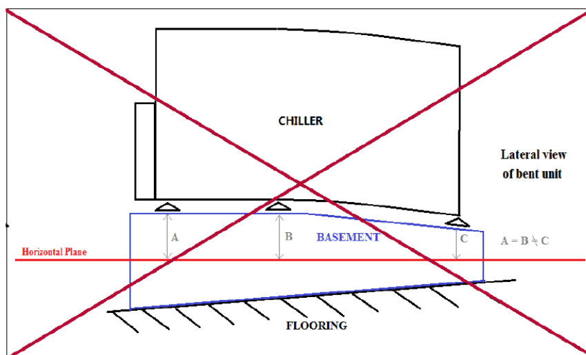
Rys. 23– Pозиomowanie jednostki
