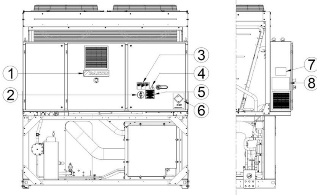
Rys. 3. - Opis tabliczek umieszczonych na panelu elektrycznym małej.
