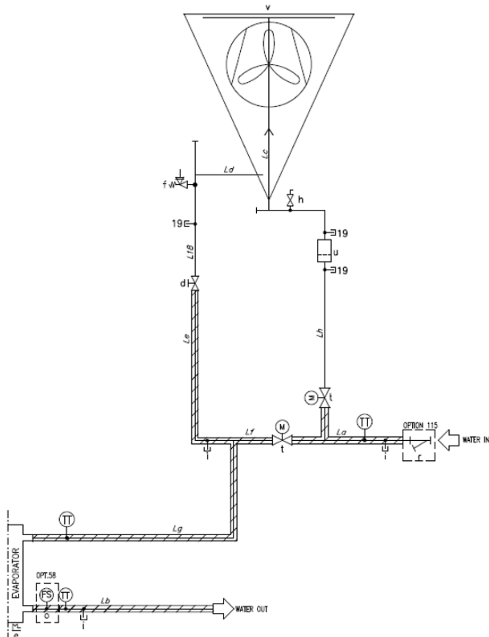
Fig. 28— Hydronisk frikylning P&ID
