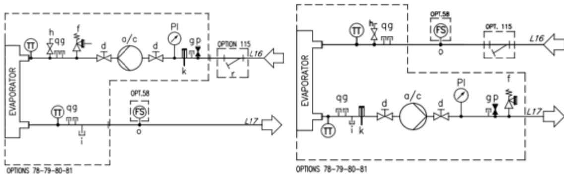
Abb. 27 – Hydraulikschema (opt. 78-79-80-81)
