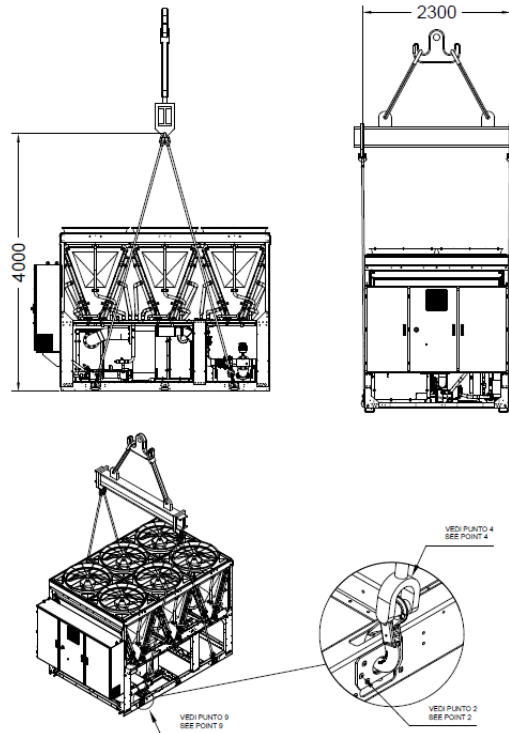
Abb. 18 – Hebeanleitung
