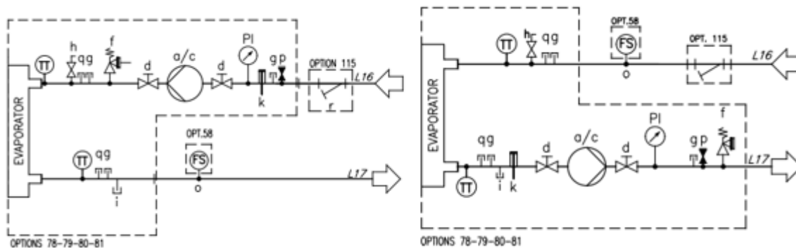
Εικ. 27 – Διάγραμμα υδραυλικού (επιλογή 78-79-80-81)
