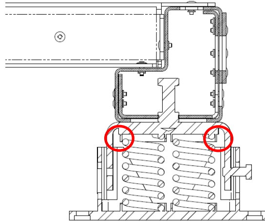
Εικ. 22 – Τοποθέτηση αντικραδασμικών στοιχείων (παρέχονται ως προαιρετικά)
