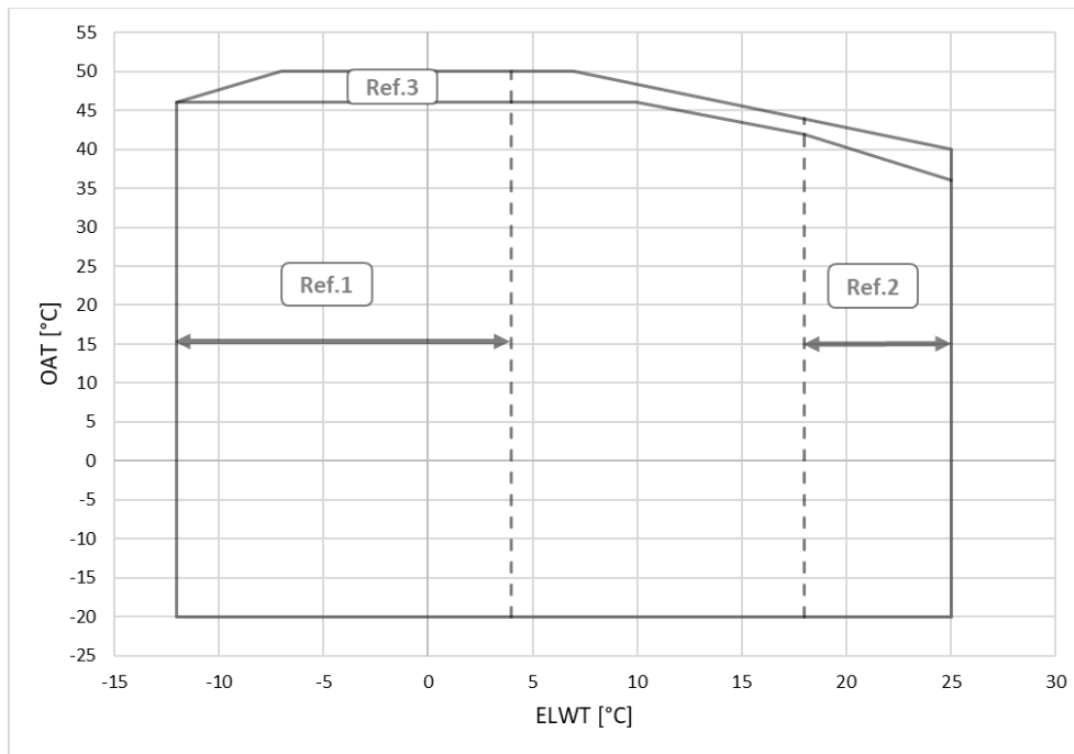
Fig. 8 – EWAD-TZD envelope unité Silver
