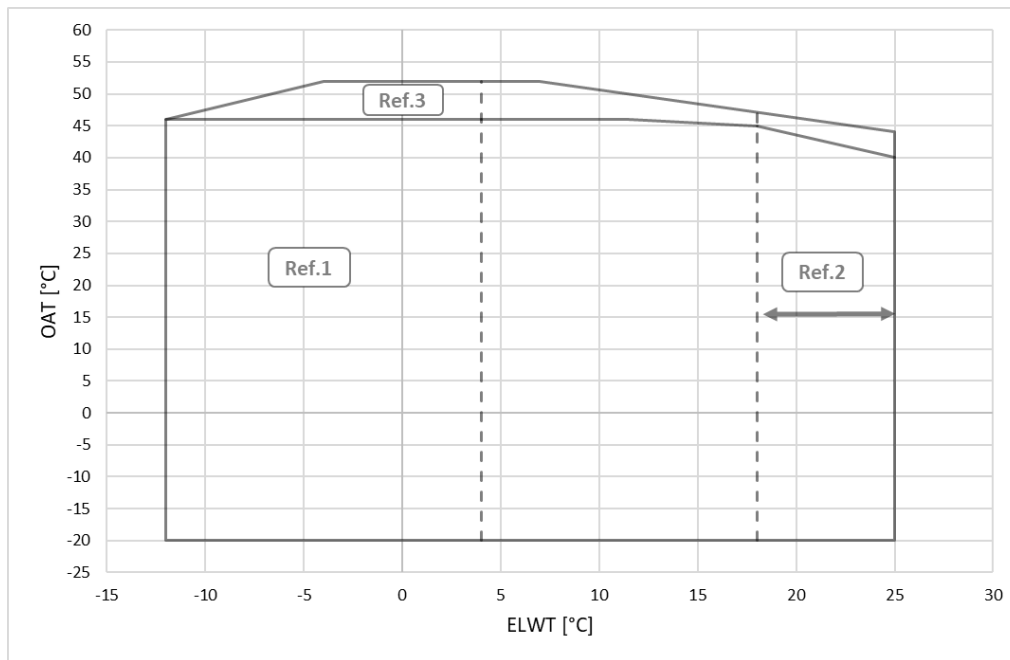
Fig. 9 – EWAD-TZD enveloppe unité Gold et Platinum
