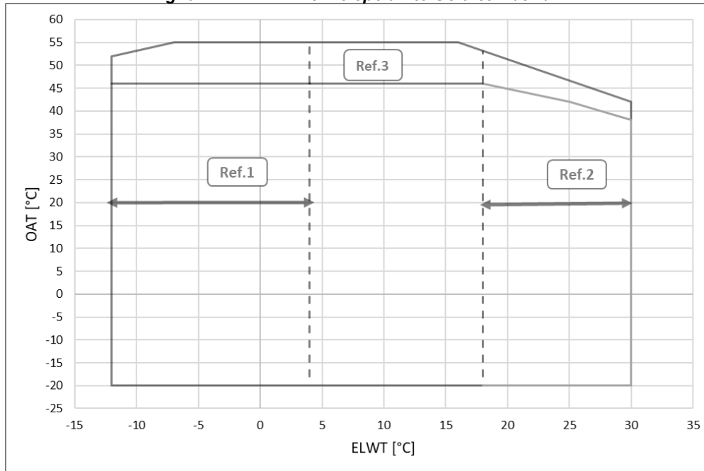
Fig. 6 – EWAH-TZD enveloppe unité Gold et Platinum
