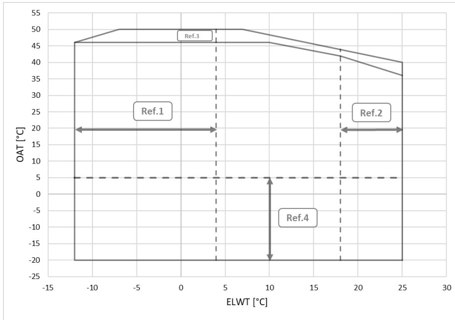
Fig. 8 – EWAD-TZD envelope unité Silver
