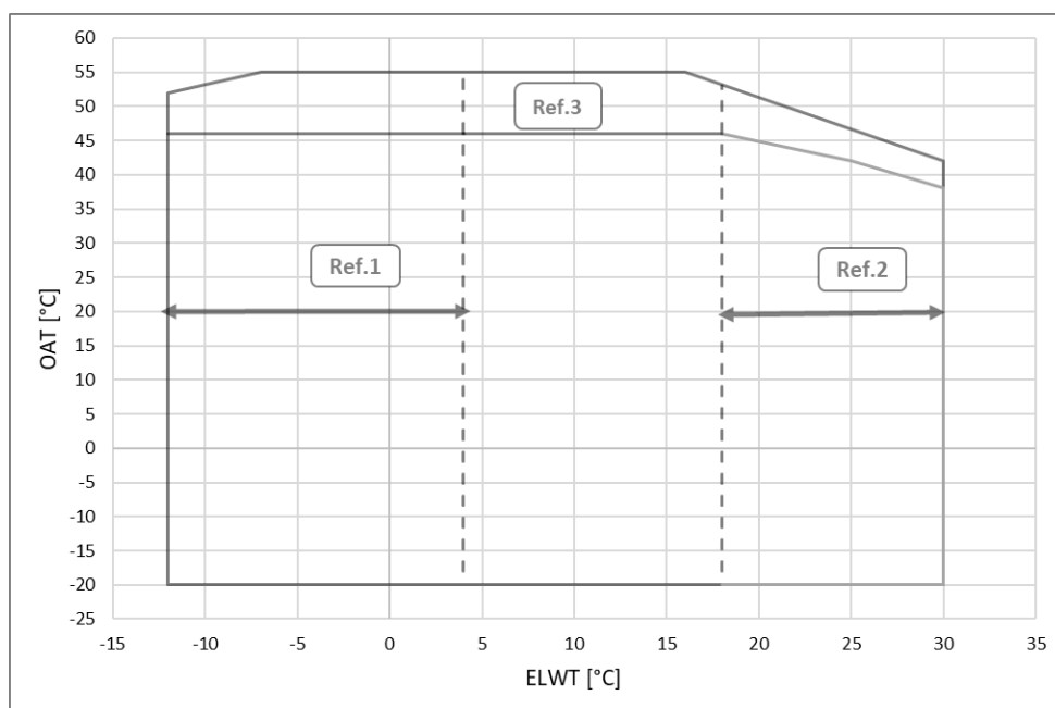
Fig. 14 – EWFH-TZD enveloppe unité Gold et Platinum
