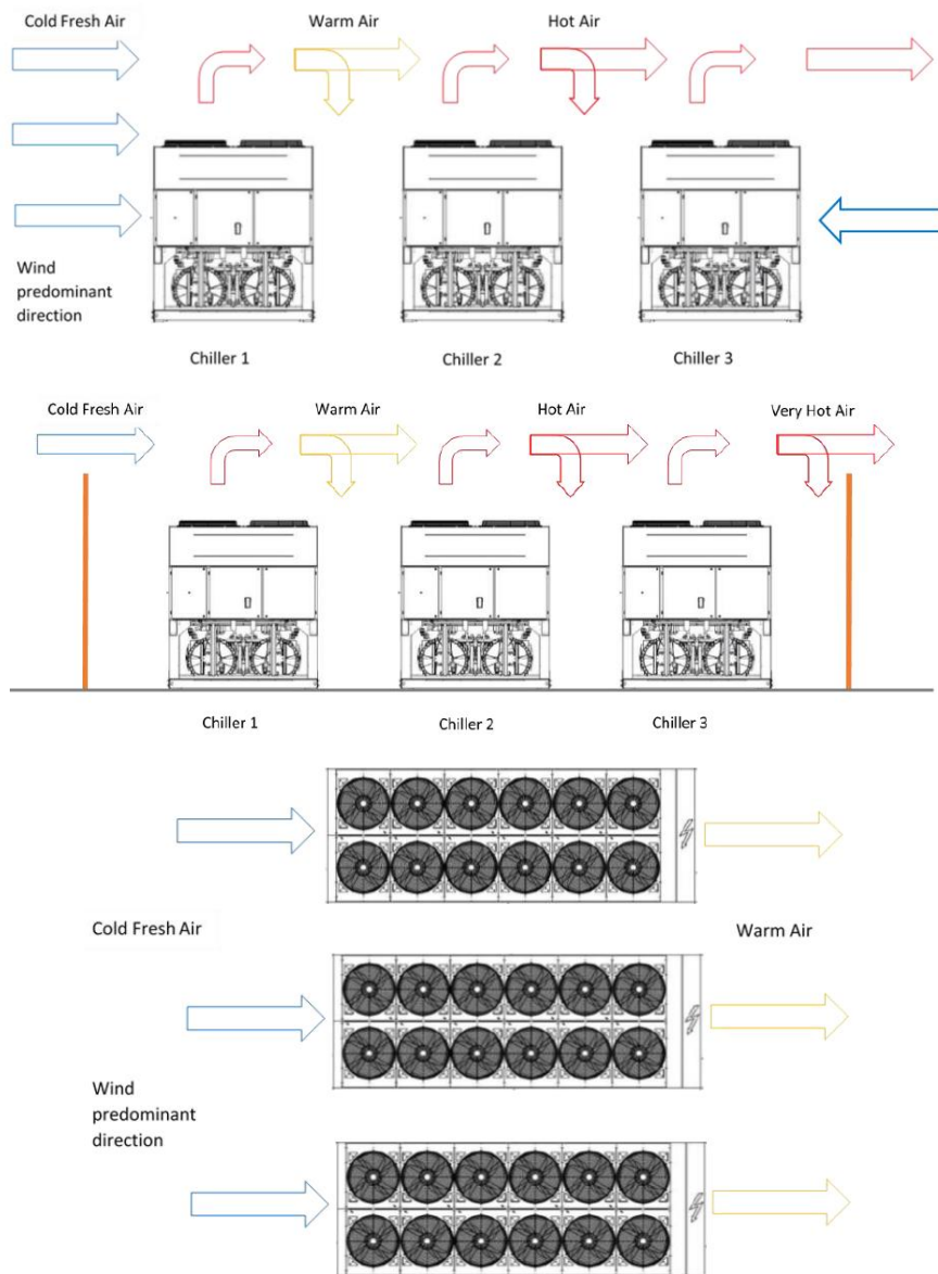
Fig. 26 – Installation de refroidisseurs multiples
