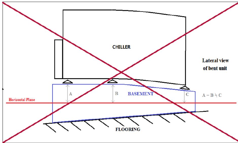
Fig. 23 – Nivellement de l'unité
