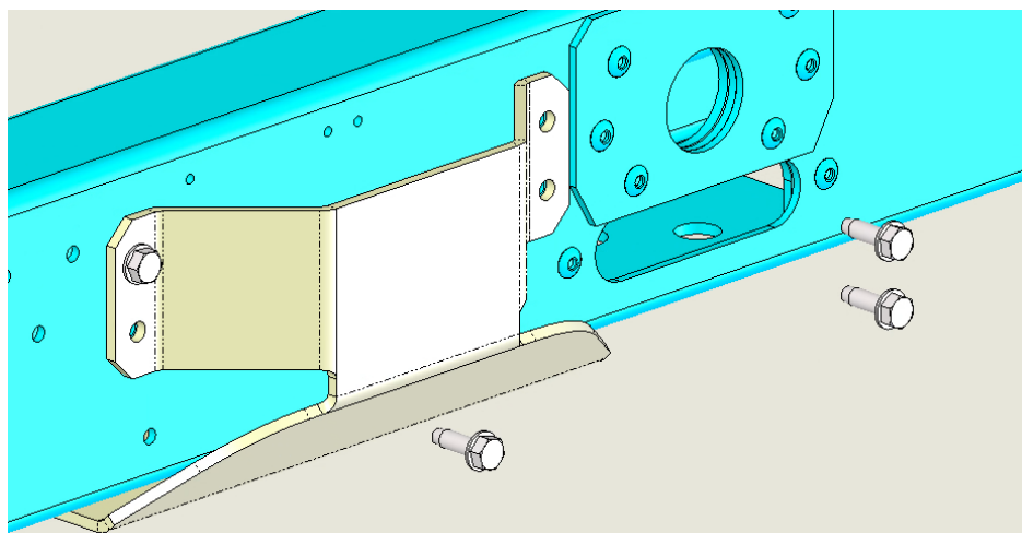
Figura 22 – Șuruburi M8 pentru conectarea cadrului unității la placă
