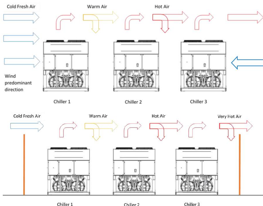
Figura 26. – Instalarea mai multor dispozitive de răcire
