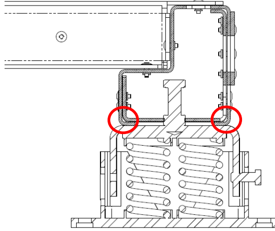
Şek. 24- Titreşim önleyici elemanların montajı (isteğe bağlı olarak temin edilir)
