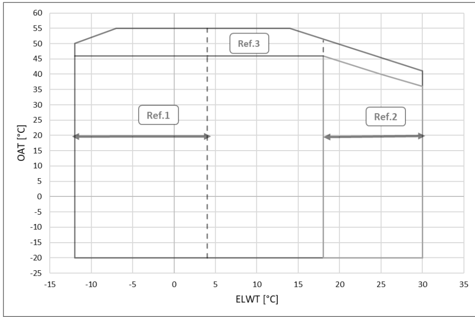
Şekil 14- EFWH-TZD Altın ve Platin ünite zarfı
