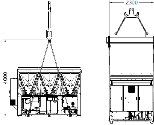
Şek. 18– Kaldırma talimatları
