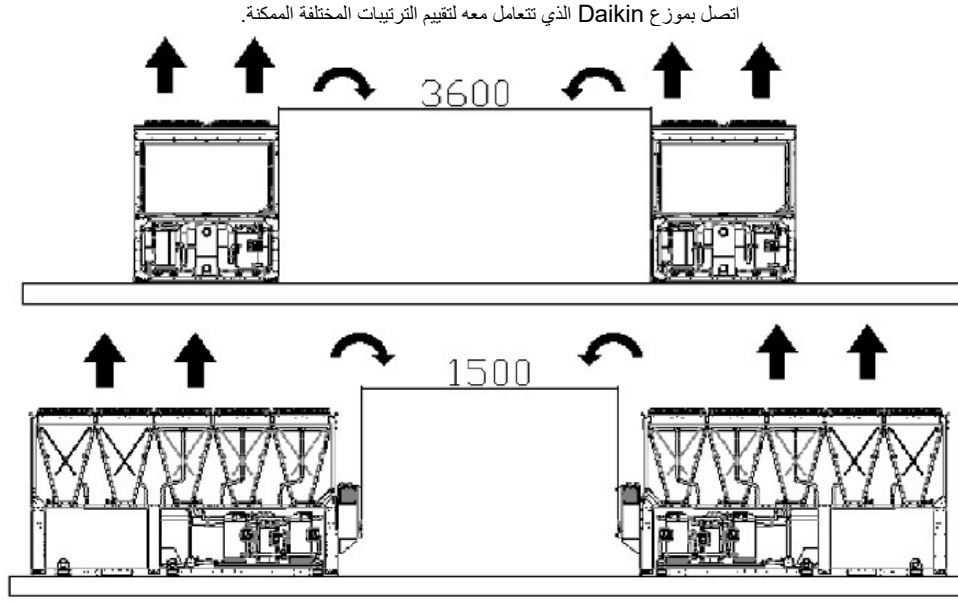
الشكل 16 – الحد الأدنى لمتطلبات الخلوص
