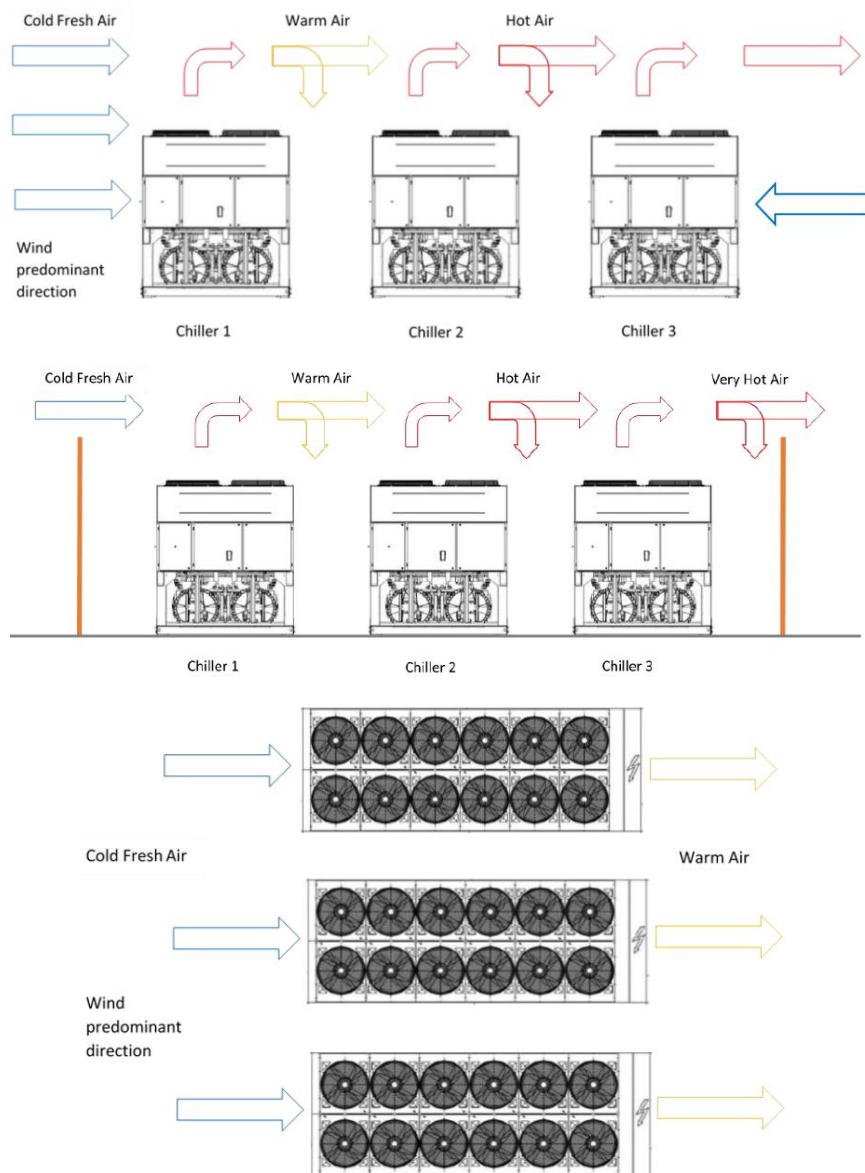
الشكل 17 - تركيب أكثر من مبرد واحد
