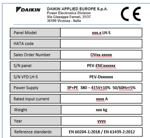
Фиг.9 - Идентификационен етикет за електрическо табло
